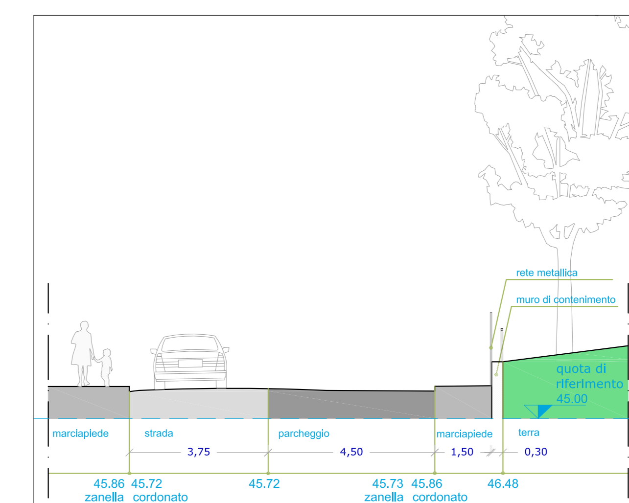
sezione f_ progetto | scala 1:100
