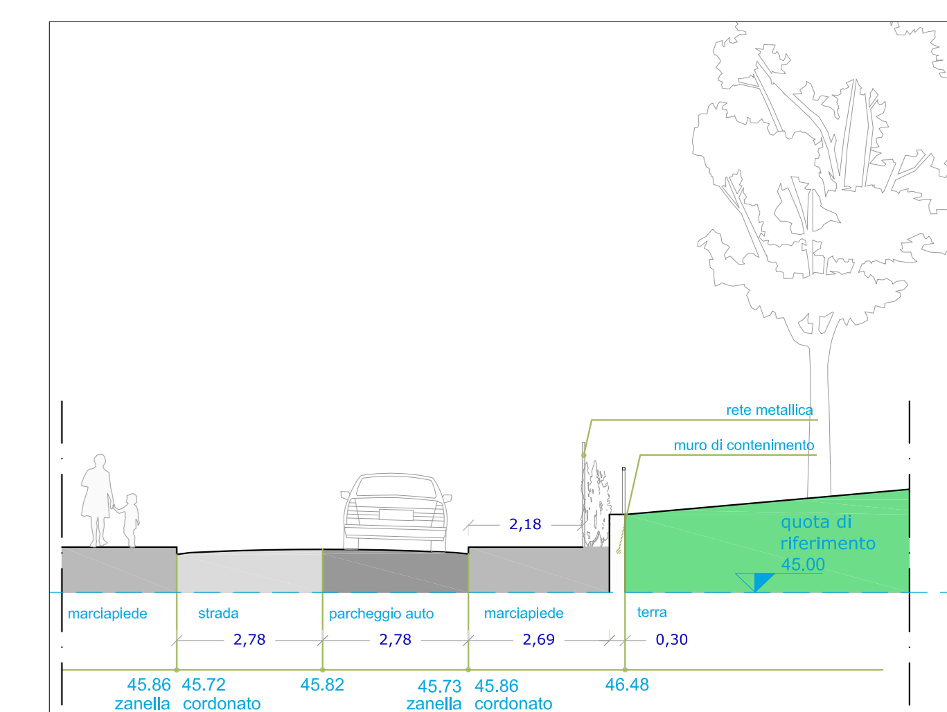
sezione f_ attuale | scala 1:100
