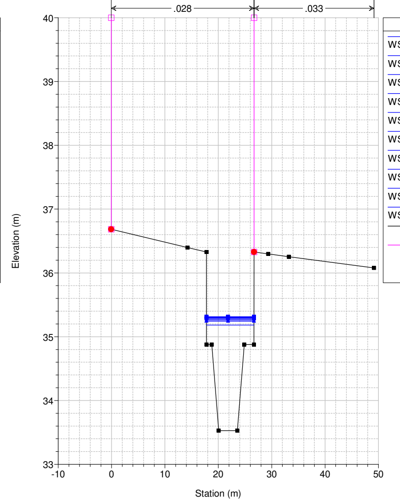
Studio Scandicci Torrenti Greve-Vingone River = Fosso Rigone Reach = Rigone 03 RS = 28 RI1016_C
