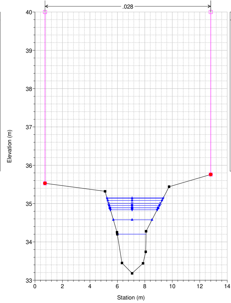
Studio Scandicci Torrenti Greve-Vingone River = Fosso Stagnolo Reach = Stagnolo RS = 32 ST0046_A
