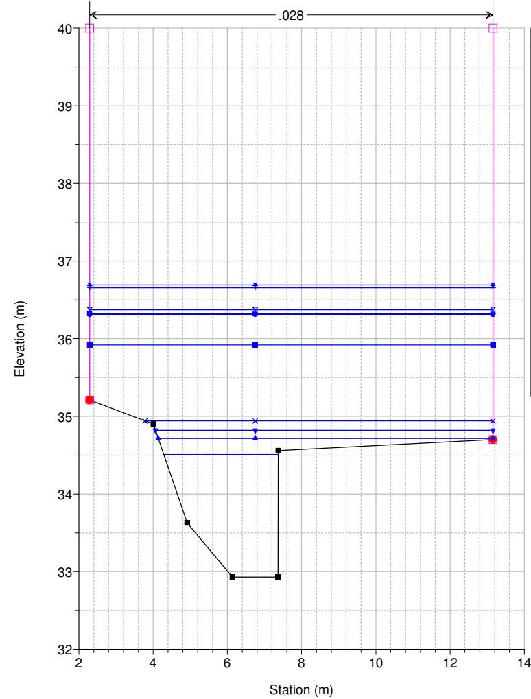
Studio Scandicci Torrenti Greve-Vingone River = Fosso Stagno Reach = Stagno RS = 15 SG0046_A
