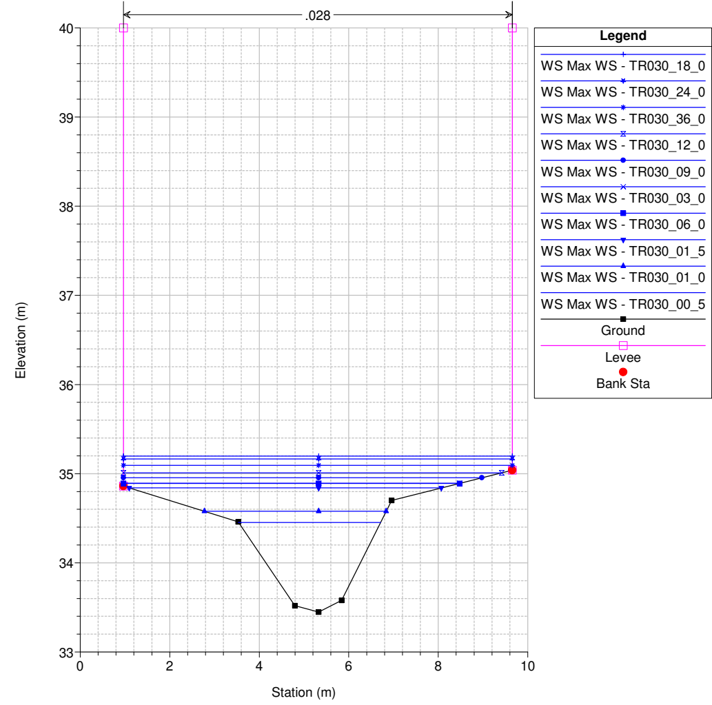
Studio Scandicci Torrenti Greve-Vingone River = Fosso Stagnolo Reach = Stagnolo RS = 57 ST0030__
