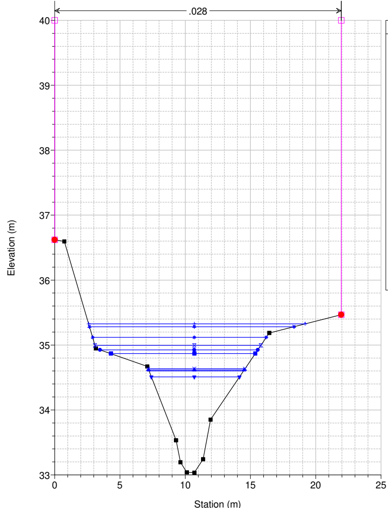
Studio Scandicci Torrenti Greve-Vingone River = Fosso Stagno Reach = Stagno RS = 74 SG0017_B
