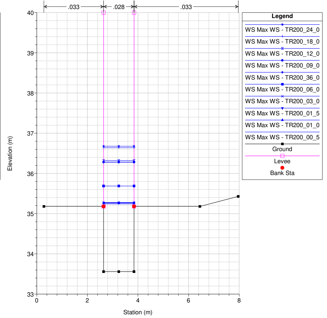
Studio Scandicci Torrenti Greve-Vingone River = Fosso Stagnacci Reach = Stagnacci RS = 4 SR0003_C
