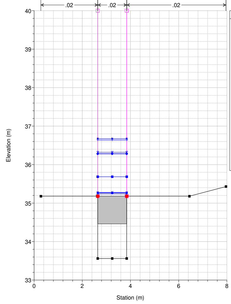
Studio Scandicci Torrenti Greve-Vingone River = Fosso Stagnacci Reach = Stagnacci RS = 4.5 BR
