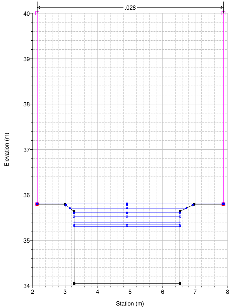
Studio Scandicci Torrenti Greve-Vingone River = Fosso Rigone Reach = Rigone 03 RS = 54 RI0006_B
