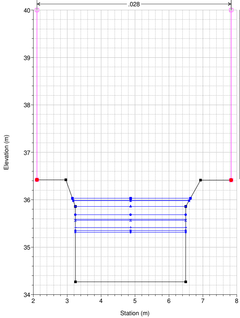
Studio Scandicci Torrenti Greve-Vingone River = Fosso Rigone Reach = Rigone 03 RS = 55.4
