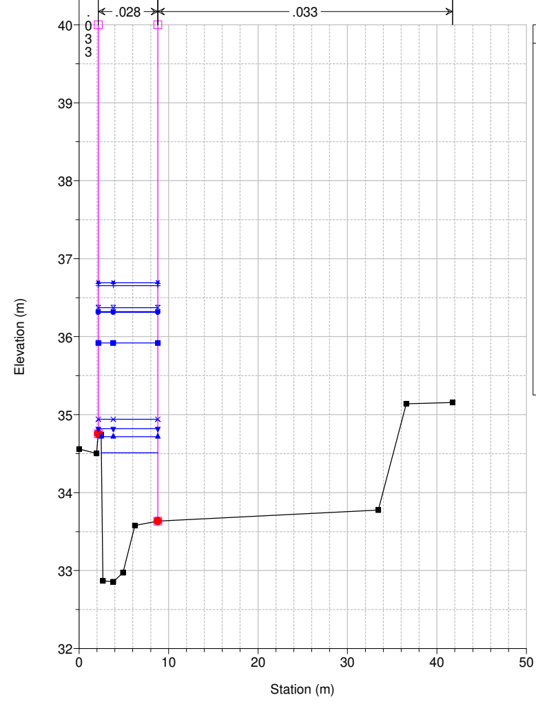
Studio Scandicci Torrenti Greve-Vingone River = Fosso Stagno Reach = Stagno RS = 37 SG0030__
