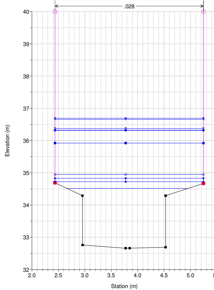
Studio Scandicci Torrenti Greve-Vingone River = Fosso Stagno Reach = Stagno RS = 46.75 BR
