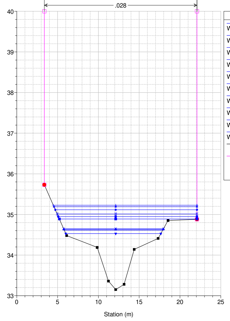
Studio Scandicci Torrenti Greve-Vingone River = Fosso Stagno Reach = Stagno RS = 83 SG0012_A
