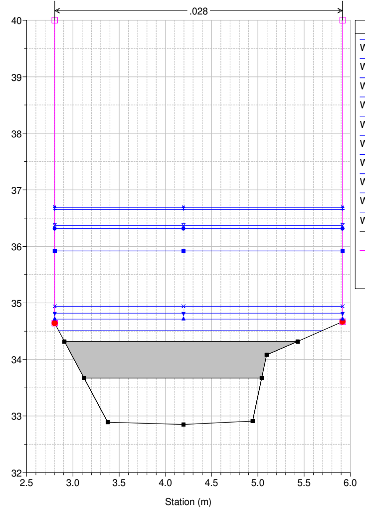
Studio Scandicci Torrenti Greve-Vingone River = Fosso Stagno Reach = Stagno RS = 26 SG0038_D
