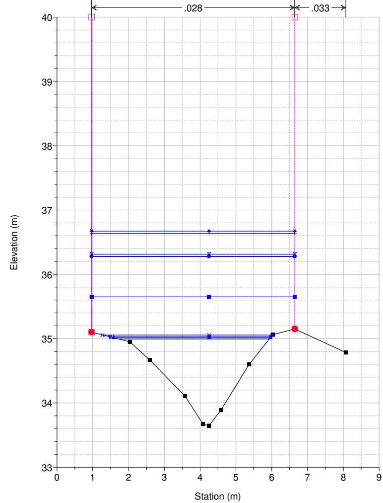
Studio Scandicci Torrenti Greve-Vingone River = Fosso Botteghino Reach = Botteghino RS = 6 SD0003_
