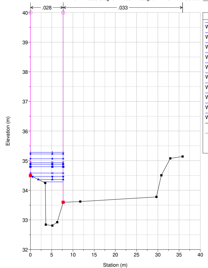
Studio Scandicci Torrenti Greve-Vingone River = Fosso Stagno Reach = Stagno RS = 36 SG0031__
