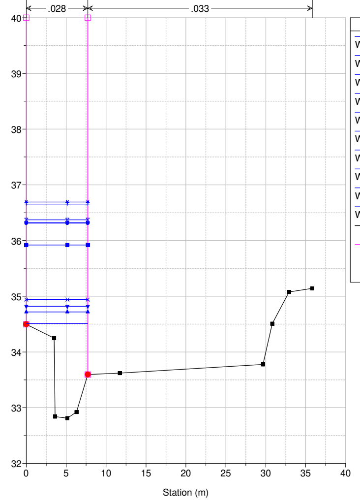
Studio Scandicci Torrenti Greve-Vingone River = Fosso Stagno Reach = Stagno RS = 36 SG0031__
