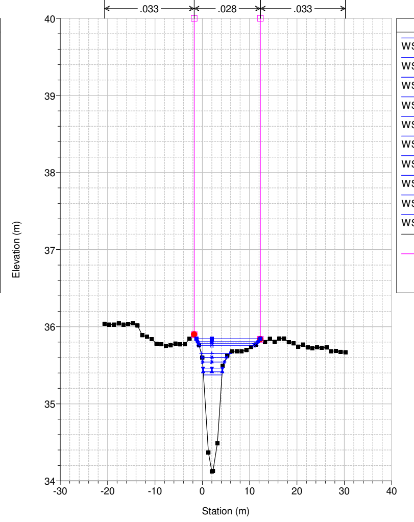
Studio Scandicci Torrenti Greve-Vingone River = Fosso Dogaione Reach = Dogaione RS = 48 DG0009_D
