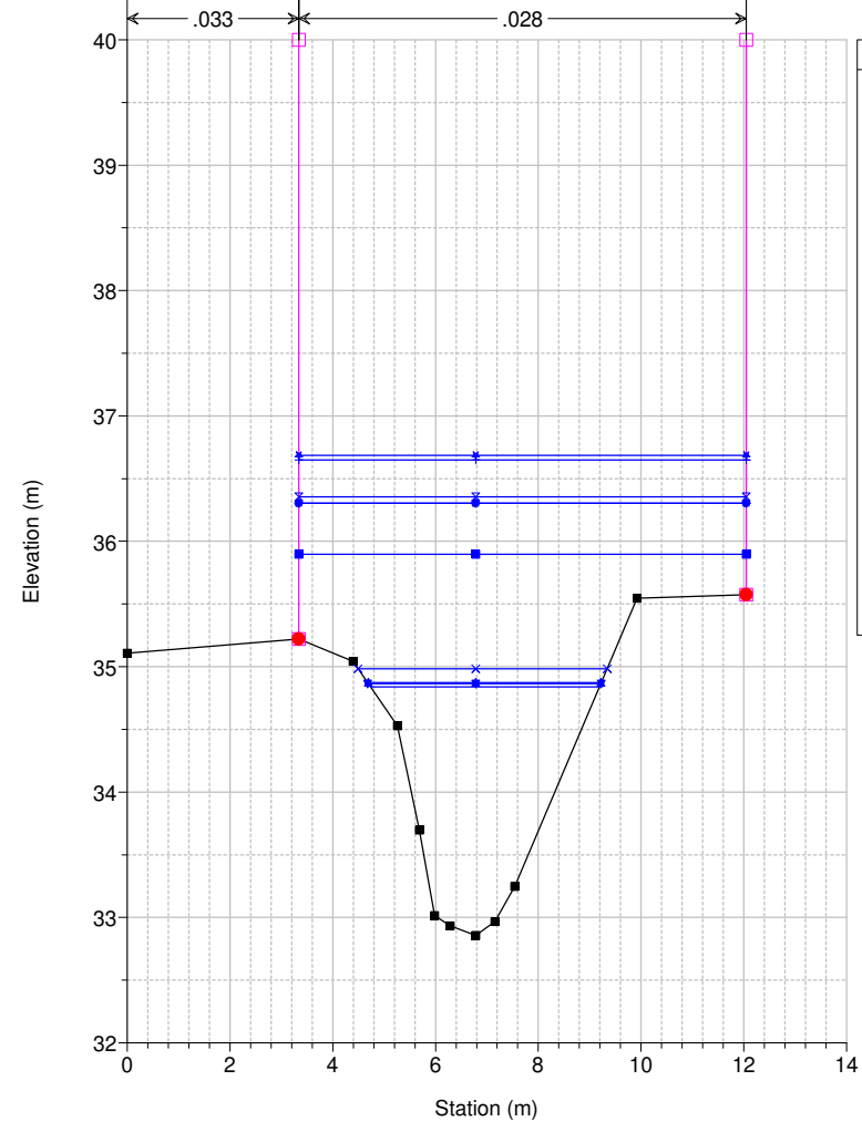
Studio Scandicci Torrenti Greve-Vingone River = Fosso Stagnolo Reach = Stagnolo RS = 20 ST0052_
