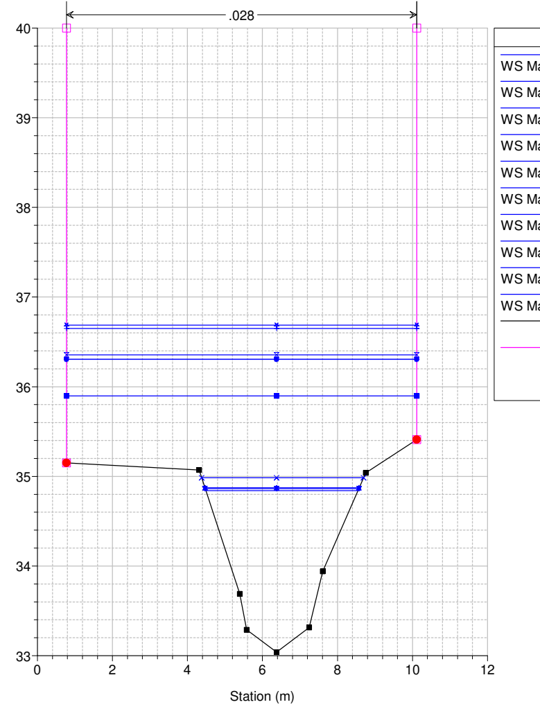
Studio Scandicci Torrenti Greve-Vingone River = Fosso Stagnolo Reach = Stagnolo RS = 23.5 BR
