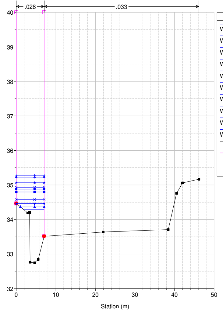
Studio Scandicci Torrenti Greve-Vingone River = Fosso Stagno Reach = Stagno RS = 30 SG0037
