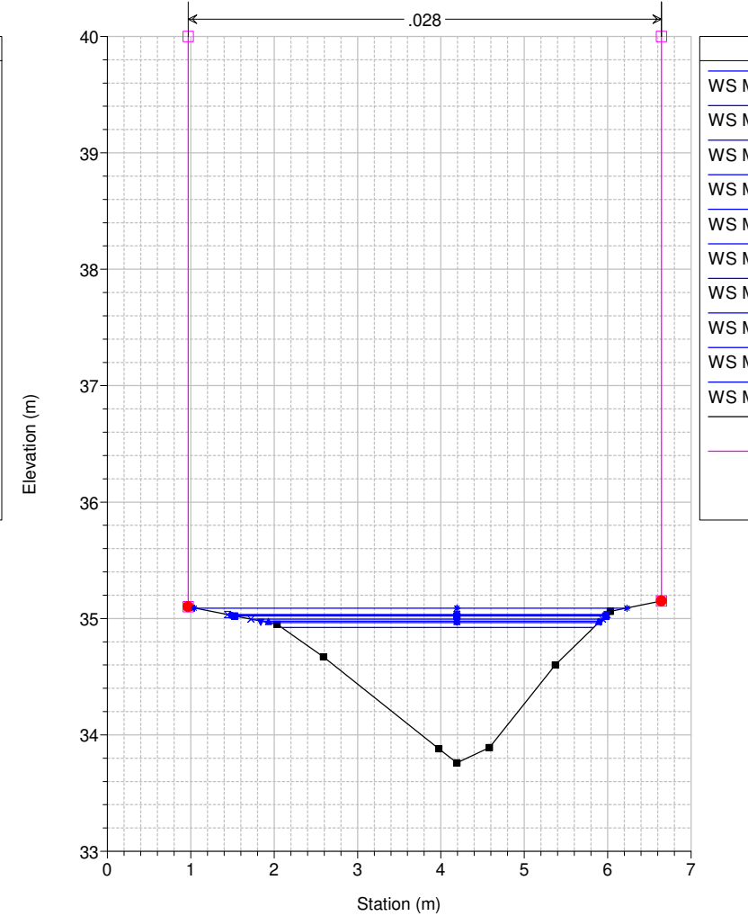
Studio Scandicci Torrenti Greve-Vingone River = Fosso Botteghino Reach = Botteghino RS = 10.5 BR
