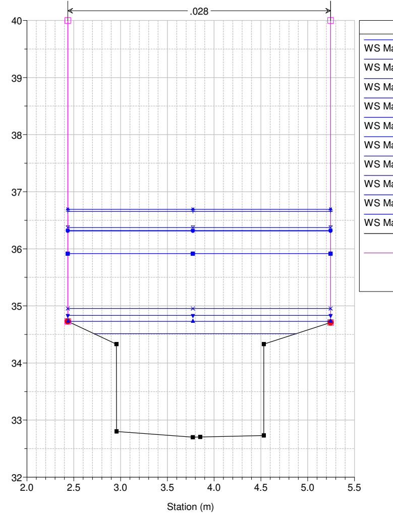
Studio Scandicci Torrenti Greve-Vingone River = Fosso Stagno Reach = Stagno RS = 48.7
