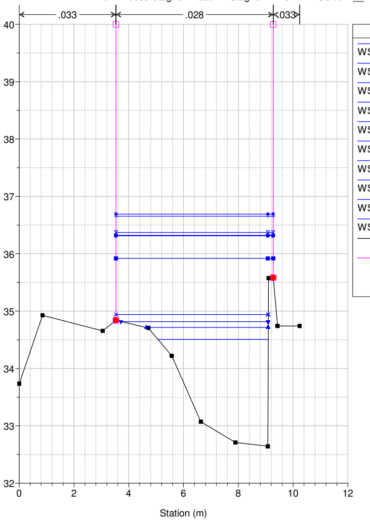
Studio Scandicci Torrenti Greve-Vingone River = Fosso Stagno Reach = Stagno RS = 11 SG0047_
