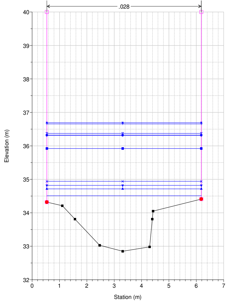
Studio Scandicci Torrenti Greve-Vingone River = Fosso Stagno Reach = Stagno RS = 23 SG0039_C
