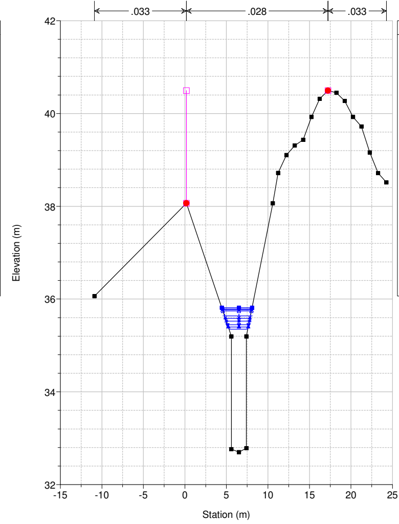
Studio Scandicci Torrenti Greve-Vingone River = Fosso Dogaione Reach = Dogaione RS = 2.6
