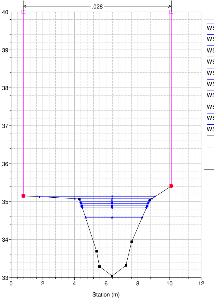
Studio Scandicci Torrenti Greve-Vingone River = Fosso Stagnolo Reach = Stagnolo RS = 23.5 BR
