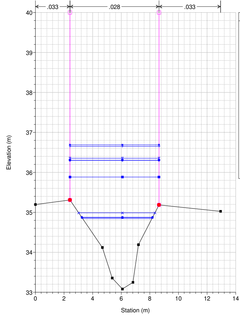
Studio Scandicci Torrenti Greve-Vingone River = Fosso Stagnolo Reach = Stagnolo RS = 52 ST0035_
