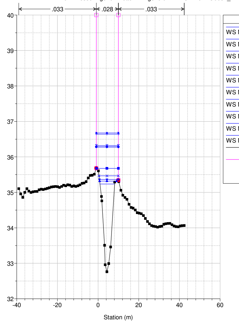
Studio Scandicci Torrenti Greve-Vingone River = Fosso Rigone Reach = Rigone 01 RS = 10 DO0032_D
