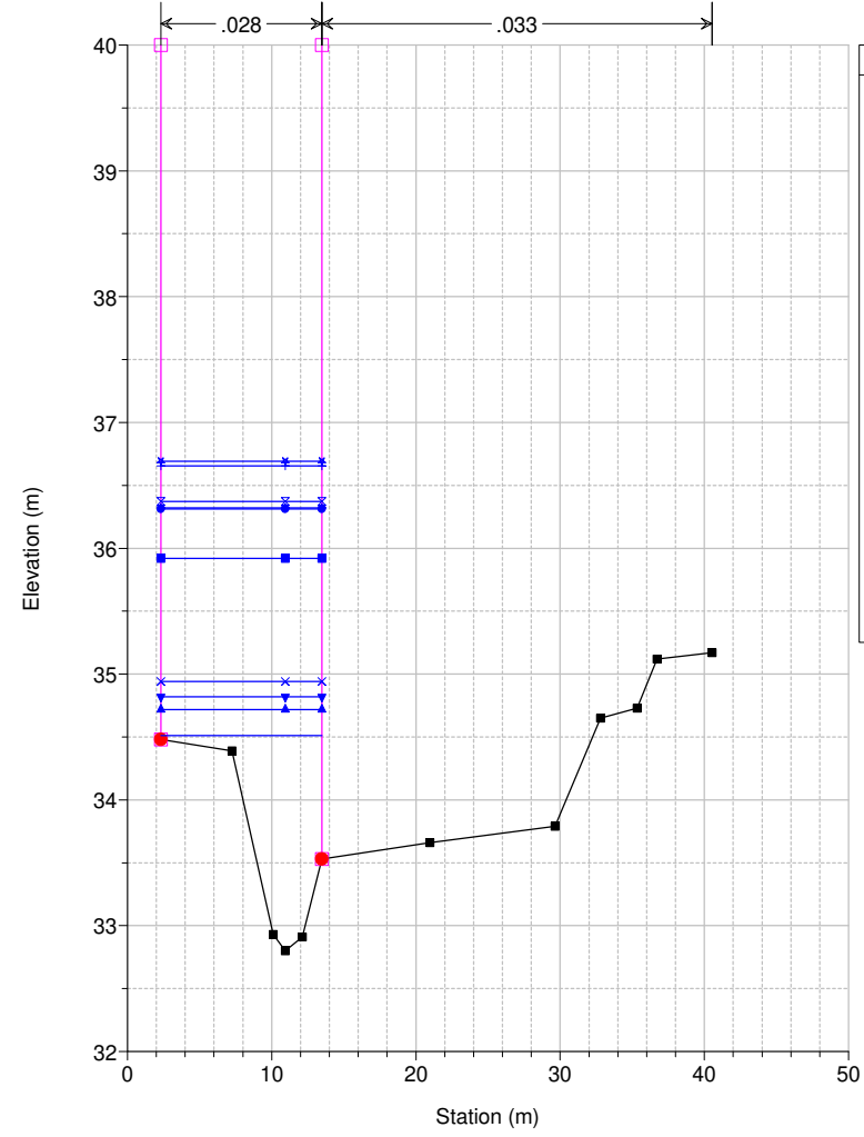
Studio Scandicci Torrenti Greve-Vingone River = Fosso Stagno Reach = Stagno RS = 31 SG0036
