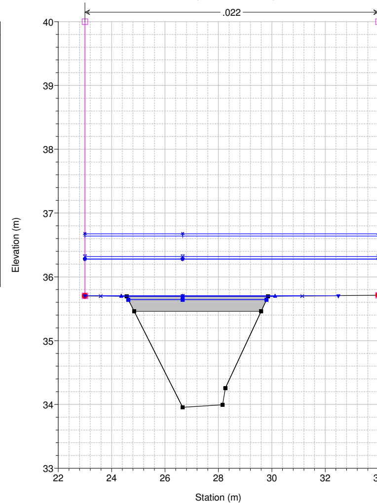
Studio Scandicci Torrenti Greve-Vingone River = Fosso Rigone Reach = Rigone 03 RS = 53.5 BR
