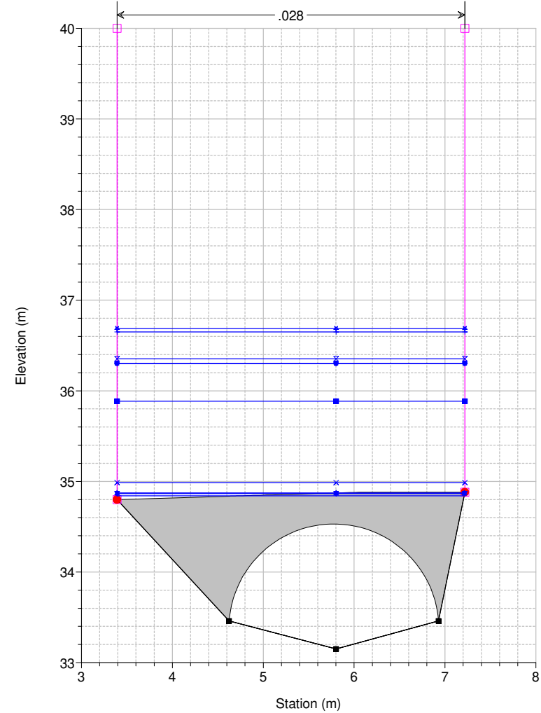
Studio Scandicci Torrenti Greve-Vingone River = Fosso Stagnolo Reach = Stagnolo RS = 47 ST0037_D
