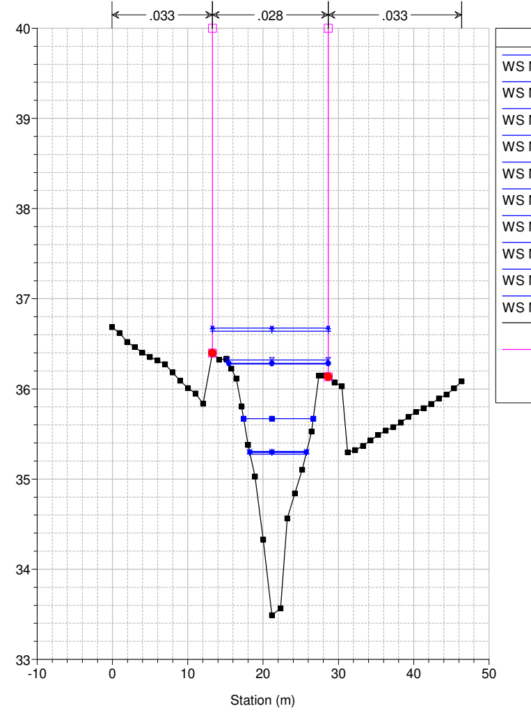
Studio Scandicci Torrenti Greve-Vingone River = Fosso Rigone Reach = Rigone 03 RS = 28.5 BR
