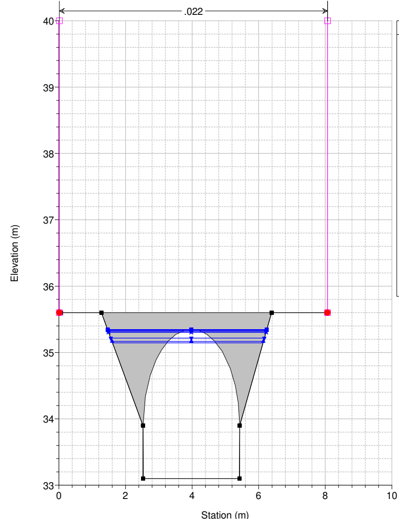
Studio Scandicci Torrenti Greve-Vingone River = Fosso Rigone Reach = Rigone 02 RS = 10.6
