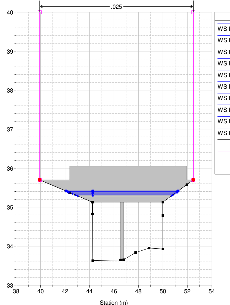
Studio Scandicci Torrenti Greve-Vingone River = Fosso Rigone Reach = Rigone 03 RS = 41 RI1011_D
