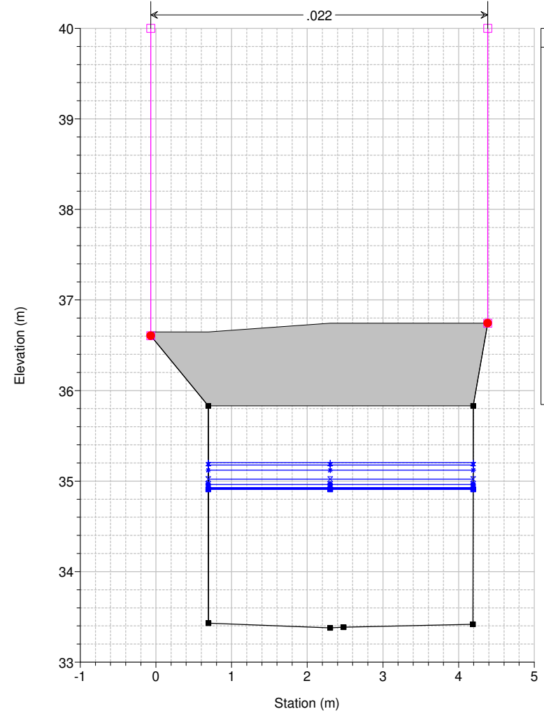
Studio Scandicci Torrenti Greve-Vingone River = Fosso Stagnolo Reach = Stagnolo RS = 100 ST0005_A
