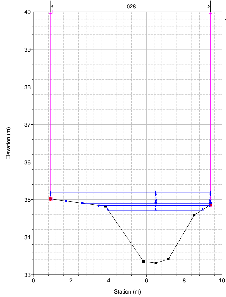
Studio Scandicci Torrenti Greve-Vingone River = Fosso Stagnolo Reach = Stagnolo RS = 82 ST0014_
