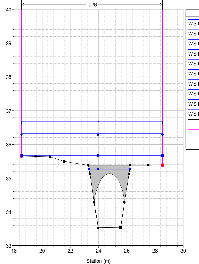
Studio Scandicci Torrenti Greve-Vingone River = Fosso Rigone Reach = Rigone 03 RS = 32.5 BR
