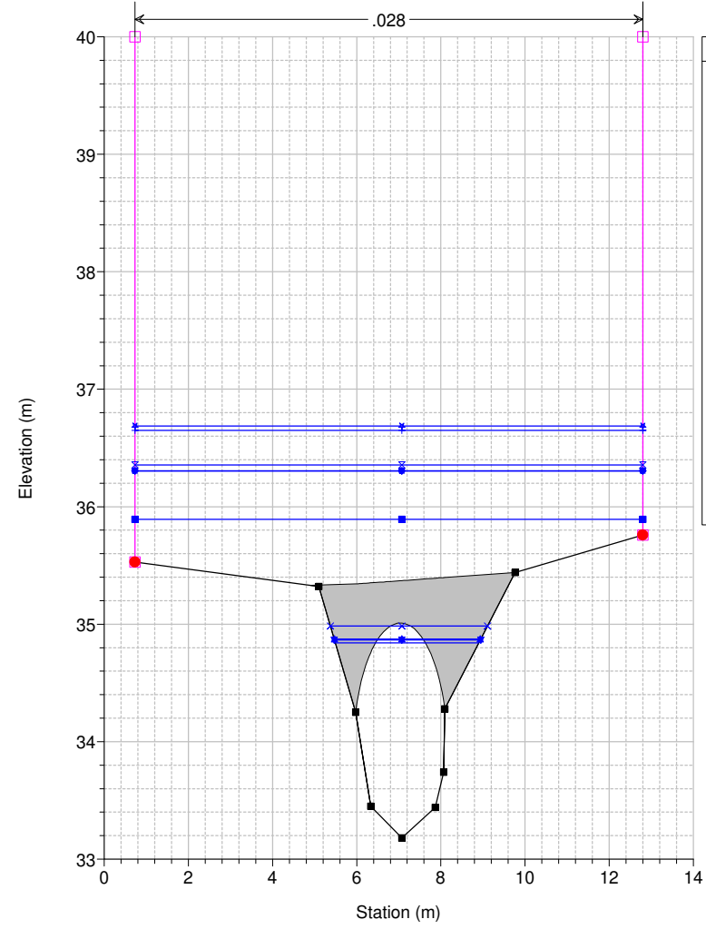
Studio Scandicci Torrenti Greve-Vingone River = Fosso Stagnolo Reach = Stagnolo RS = 34 ST0044_D
