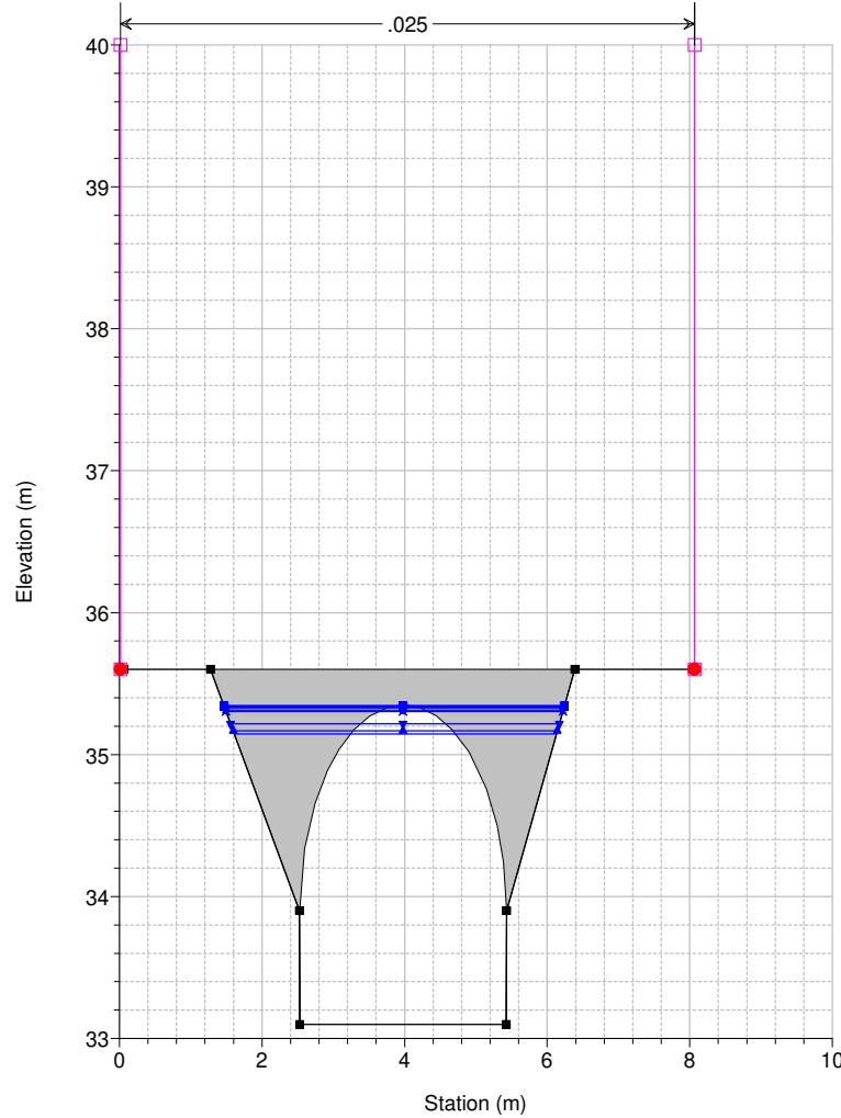
Studio Scandicci Torrenti Greve-Vingone River = Fosso Rigone Reach = Rigone 02 RS = 12.75 BR
