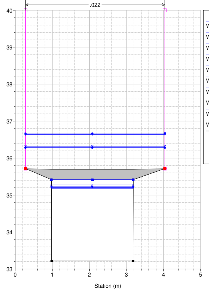
Studio Scandicci Torrenti Greve-Vingone River = Fosso Rigone Reach = Rigone 02 RS = 13.75 Culv
