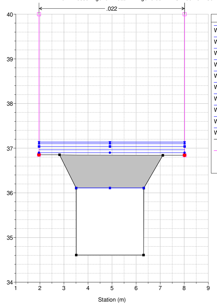
Studio Scandicci Torrenti Greve-Vingone River = Fosso Rigone Reach = Rigone 03 RS = 56.75 Culv
