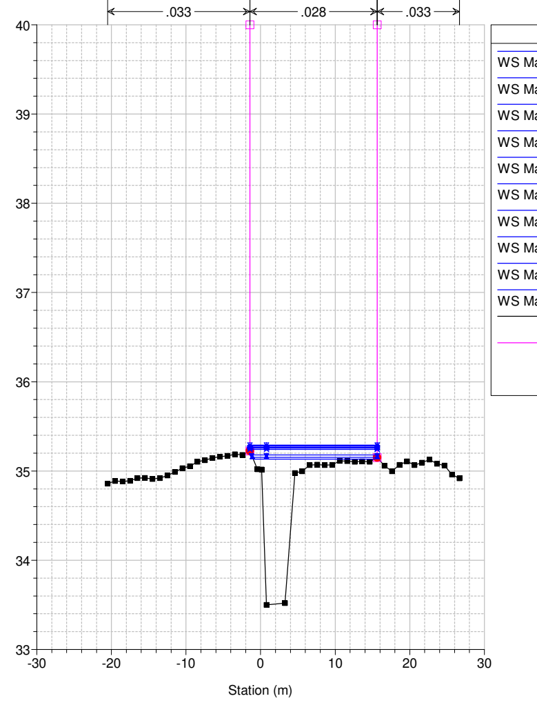
Studio Scandicci Torrenti Greve-Vingone River = Fosso Rigone Reach = Rigone 02 RS = 16 RI0021_A
