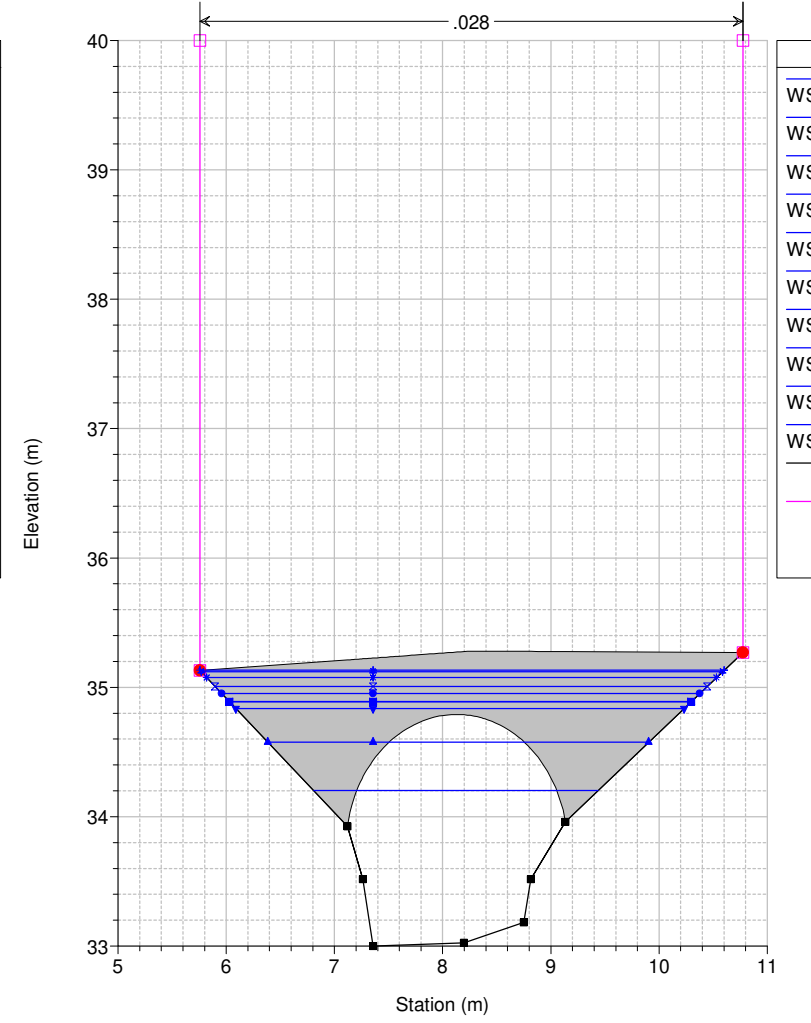
Studio Scandicci Torrenti Greve-Vingone River = Fosso Stagnolo Reach = Stagnolo RS = 28 ST0047_
