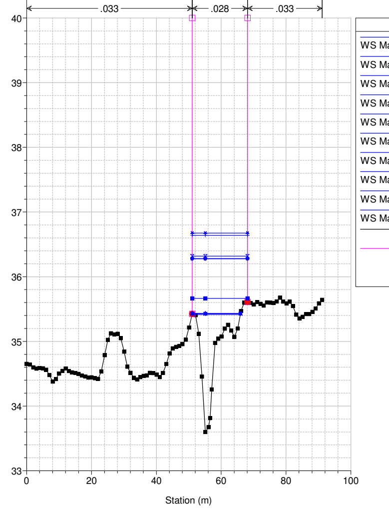
Studio Scandicci Torrenti Greve-Vingone River = Fosso Rigone Reach = Rigone 03 RS = 41 RI1011_D
