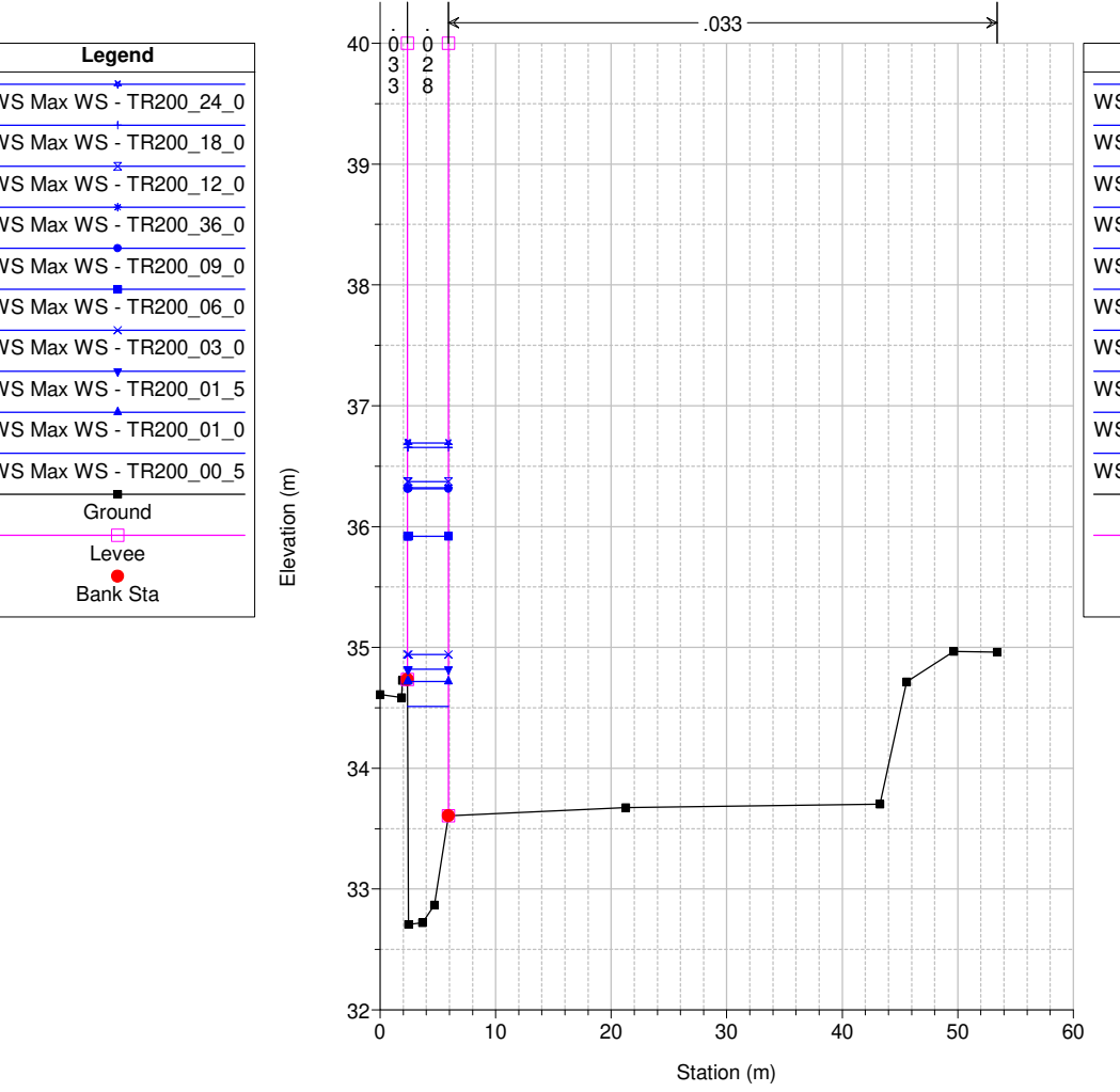
Studio Scandicci Torrenti Greve-Vingone River = Fosso Stagno Reach = Stagno RS = 29 SG0038_A
