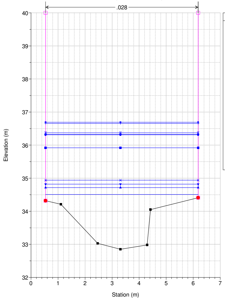
Studio Scandicci Torrenti Greve-Vingone River = Fosso Stagno Reach = Stagno RS = 22 SG0039_D
