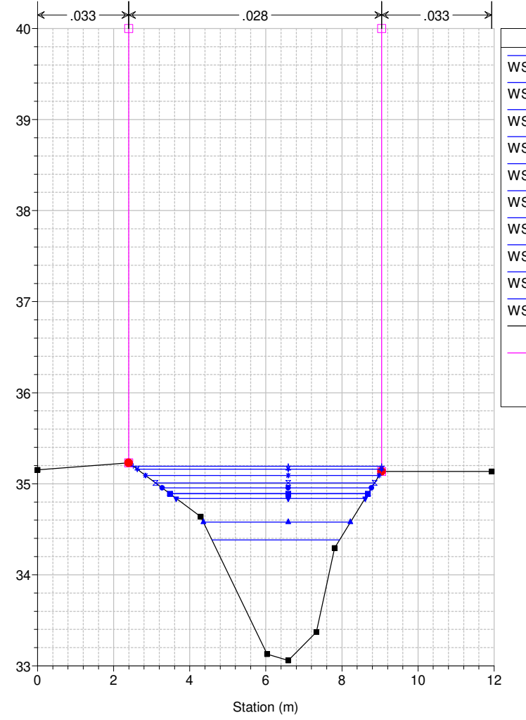
Studio Scandicci Torrenti Greve-Vingone River = Fosso Stagnolo Reach = Stagnolo RS = 51 ST0036__
