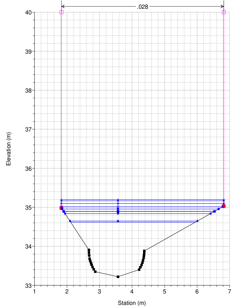
Studio Scandicci Torrenti Greve-Vingone River = Fosso Stagnolo Reach = Stagnolo RS = 72 ST0021_A
