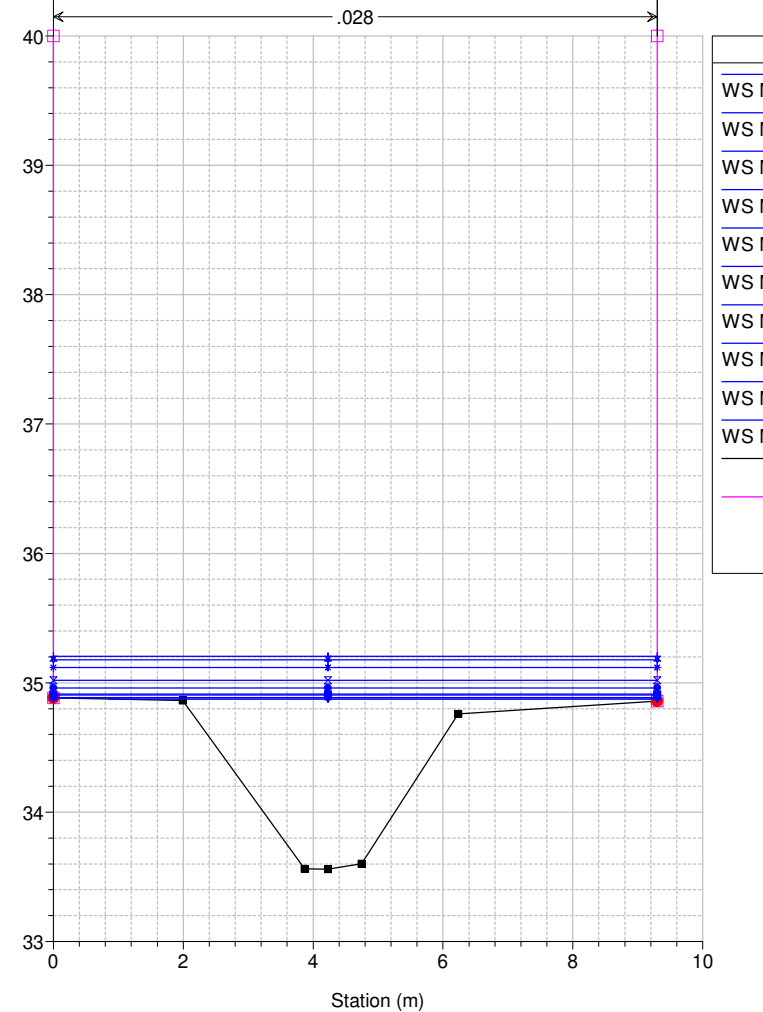
Studio Scandicci Torrenti Greve-Vingone River = Fosso Stagnolo Reach = Stagnolo RS = 95 ST0007_
