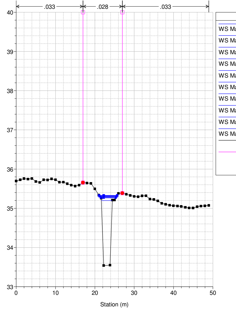
Studio Scandicci Torrenti Greve-Vingone River = Fosso Rigone Reach = Rigone 03 RS = 32.5 BR
