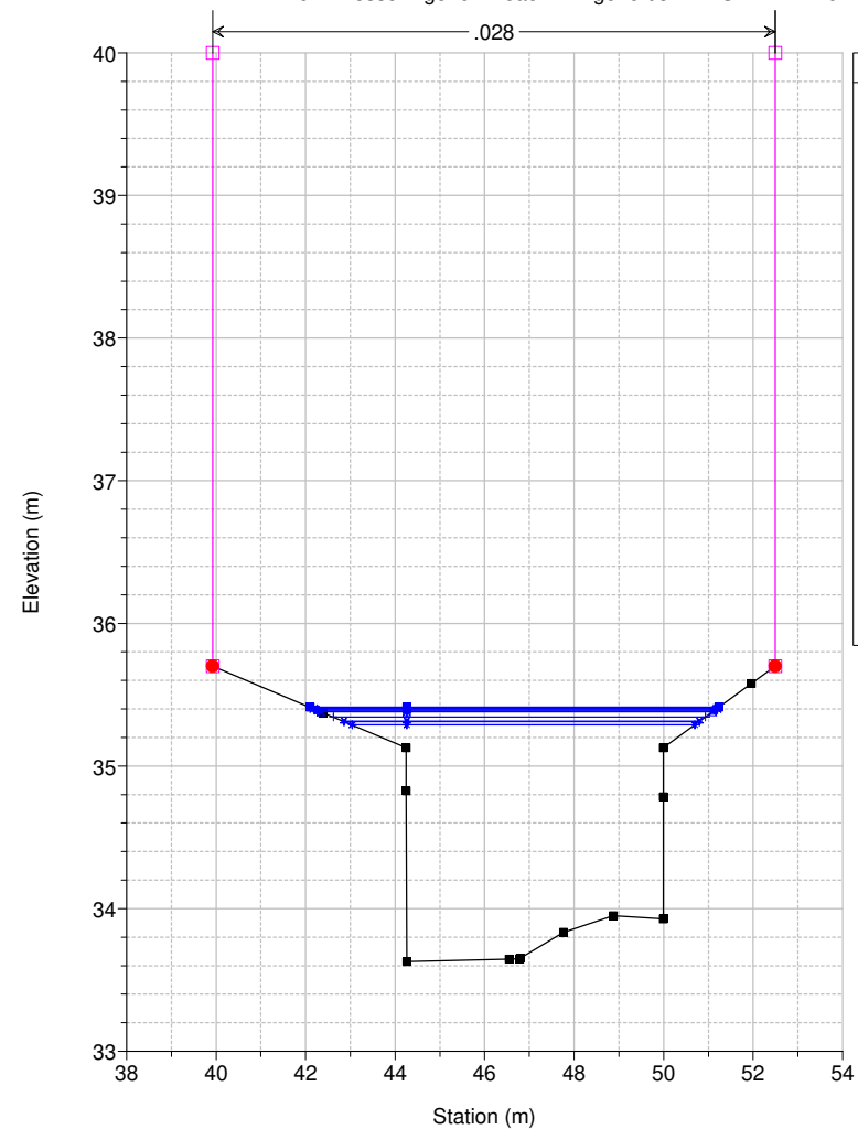
Studio Scandicci Torrenti Greve-Vingone River = Fosso Rigone Reach = Rigone 03 RS = 42 RI1011_C
