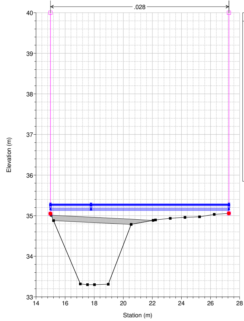
Studio Scandicci Torrenti Greve-Vingone River = Fosso Rigone Reach = Rigone 02 RS = 17 RI1020_D
