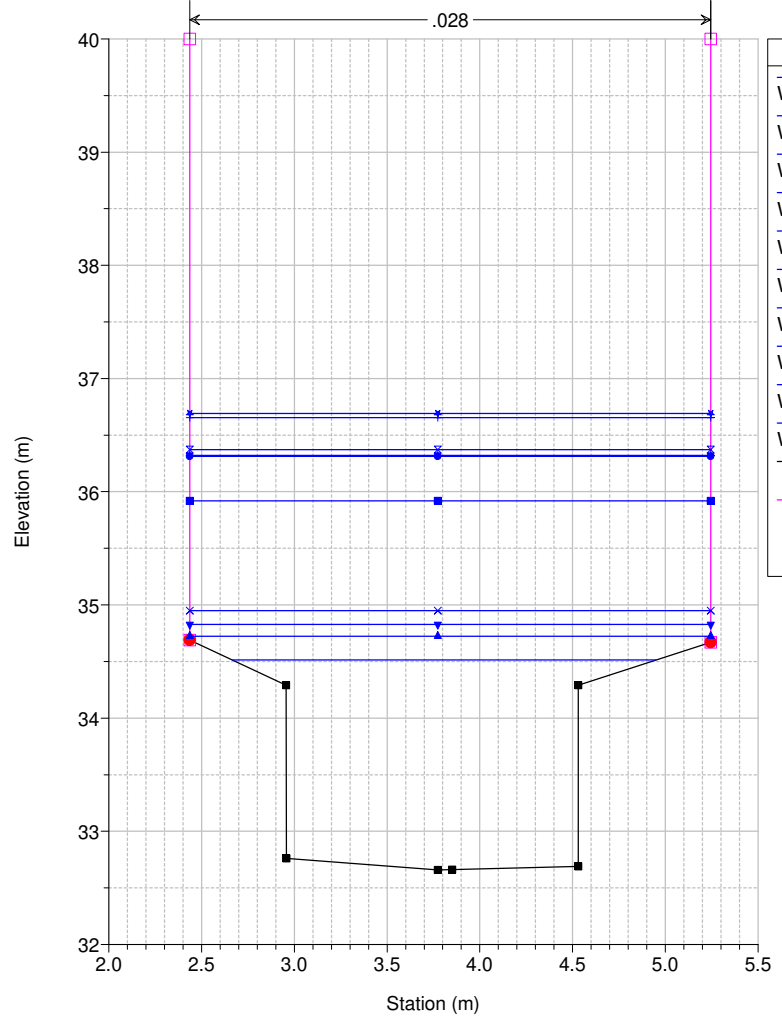
Studio Scandicci Torrenti Greve-Vingone River = Fosso Stagno Reach = Stagno RS = 47 SG0024_R
