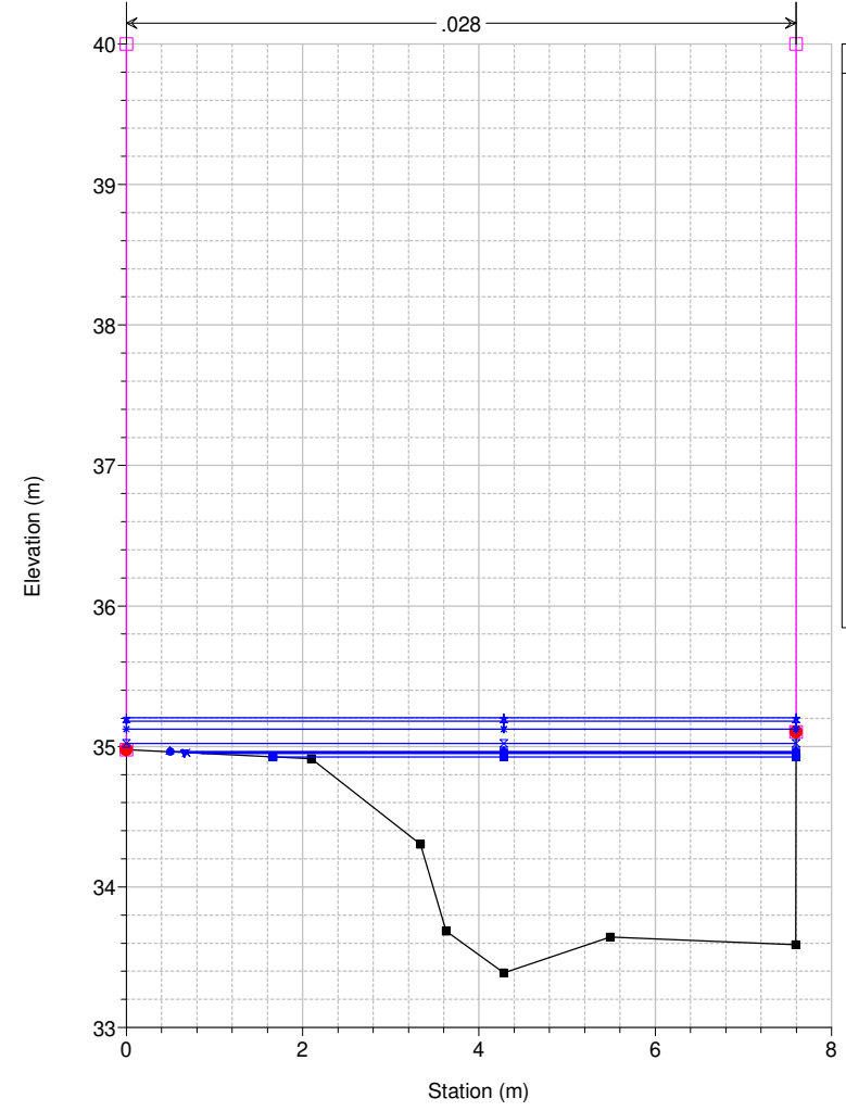
Studio Scandicci Torrenti Greve-Vingone River = Fosso Stagnolo Reach = Stagnolo RS = 103 ST0004_B
