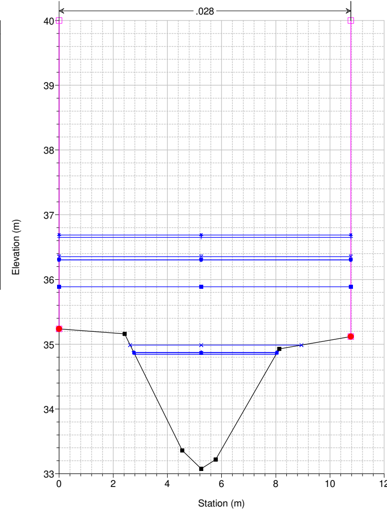
Studio Scandicci Torrenti Greve-Vingone River = Fosso Stagnolo Reach = Stagnolo RS = 46 ST0038_
