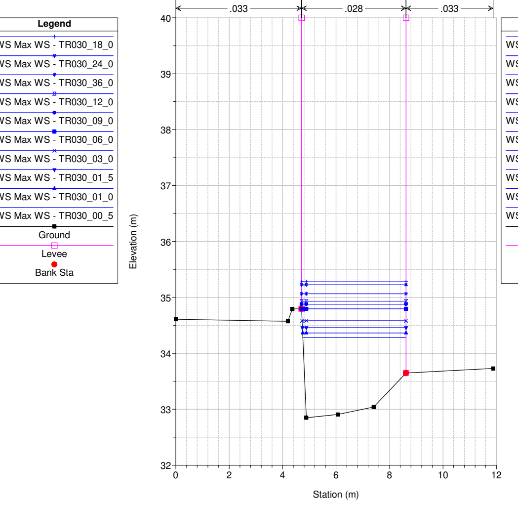
Studio Scandicci Torrenti Greve-Vingone River = Fosso Stagno Reach = Stagno RS = 41 SG0026_
