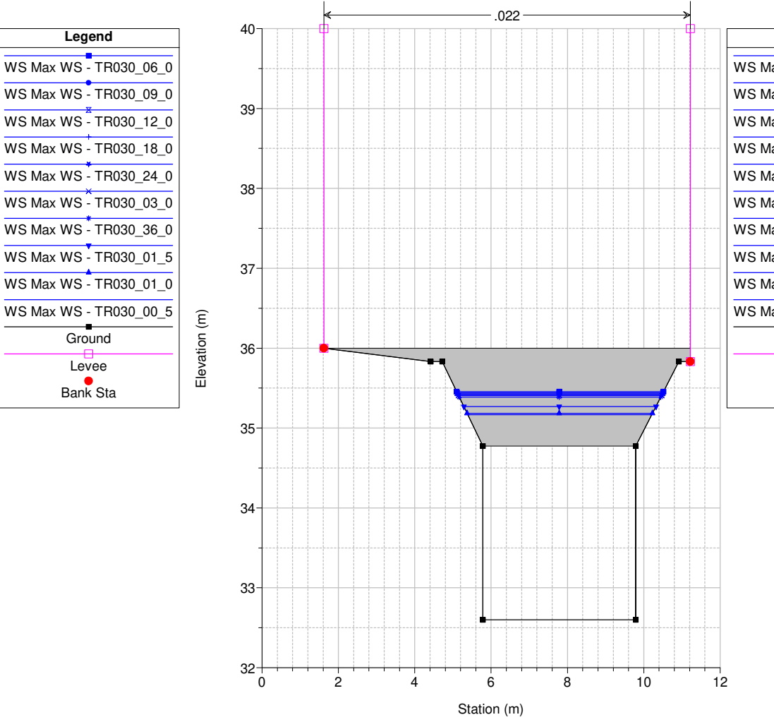
Studio Scandicci Torrenti Greve-Vingone River = Fosso Rigone Reach = Rigone 01 RS = 6 DO1033_D
