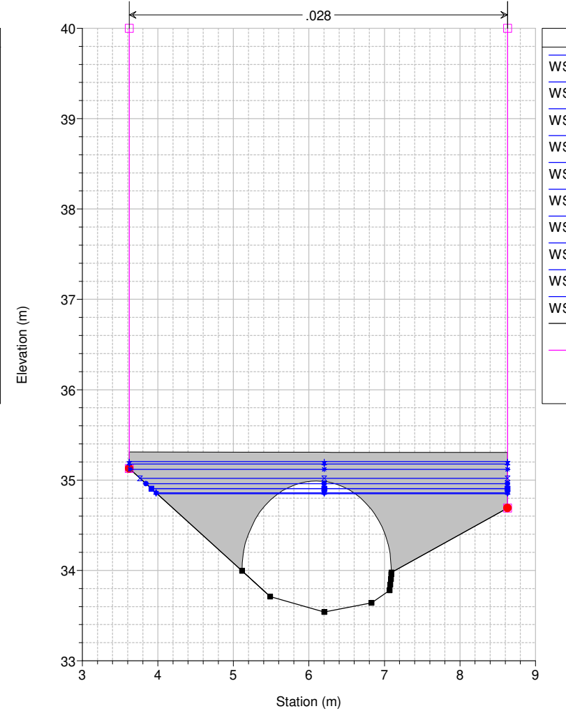
Studio Scandicci Torrenti Greve-Vingone River = Fosso Stagnolo Reach = Stagnolo RS = 90 ST0009_
