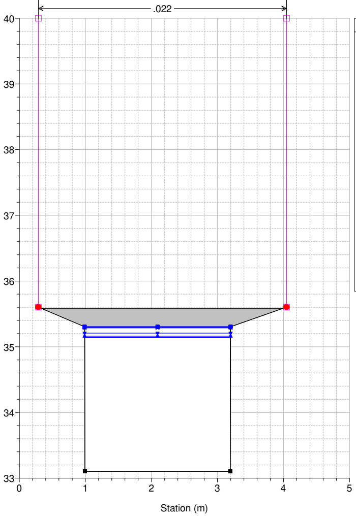
Studio Scandicci Torrenti Greve-Vingone River = Fosso Rigone Reach = Rigone 02 RS = 13.75 Culv
