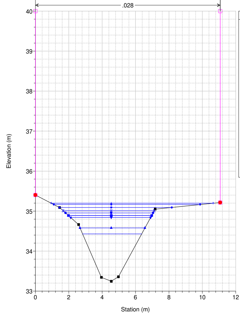
Studio Scandicci Torrenti Greve-Vingone River = Fosso Stagnolo Reach = Stagnolo RS = 58 ST0029__
