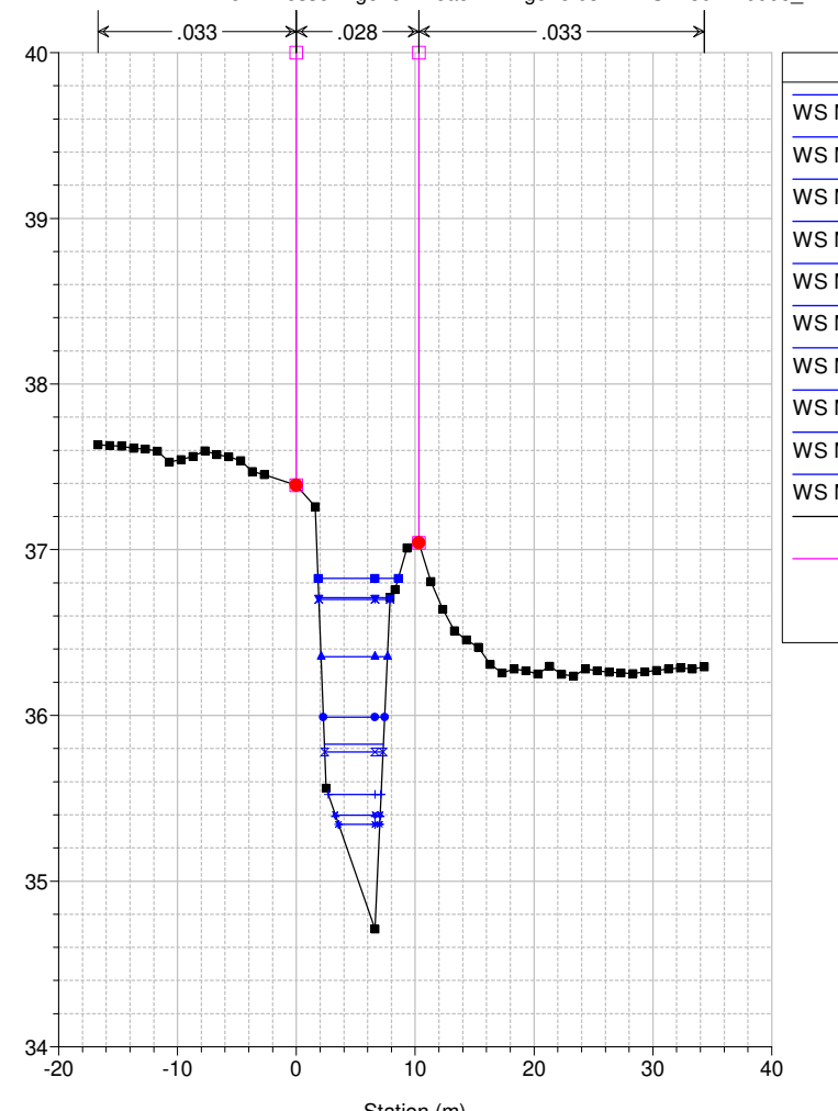
Studio Scandicci Torrenti Greve-Vingone River = Fosso Rigone Reach = Rigone 03 RS = 59 RI0005_A
