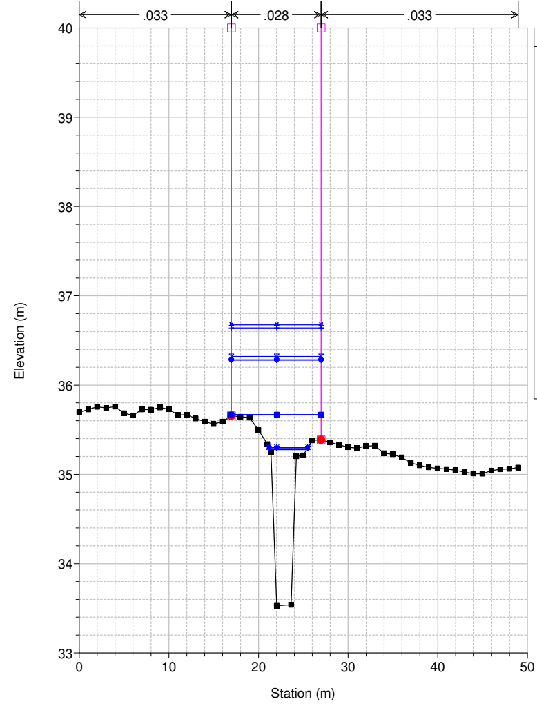
Studio Scandicci Torrenti Greve-Vingone River = Fosso Rigone Reach = Rigone 03 RS = 28.5 BR
