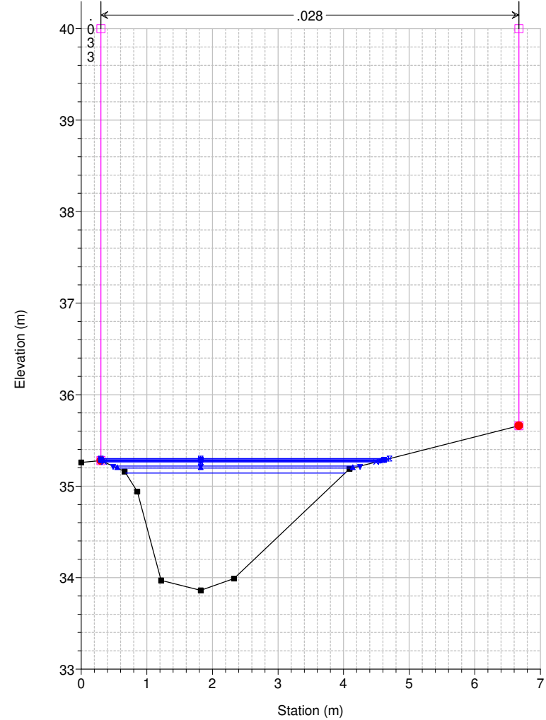
Studio Scandicci Torrenti Greve-Vingone River = Fosso Stagnacci Reach = Stagnacci RS = 4.5 BR
