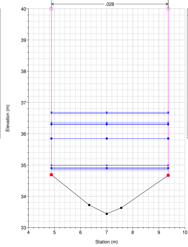
Studio Scandicci Torrenti Greve-Vingone River = Fosso Stagnolo Reach = Stagnolo RS = 86 ST0011_C
