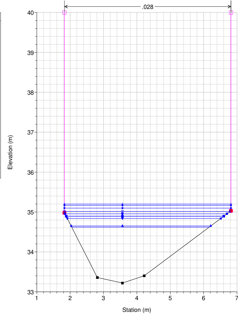
Studio Scandicci Torrenti Greve-Vingone River = Fosso Stagnolo Reach = Stagnolo RS = 71 ST0021_B
