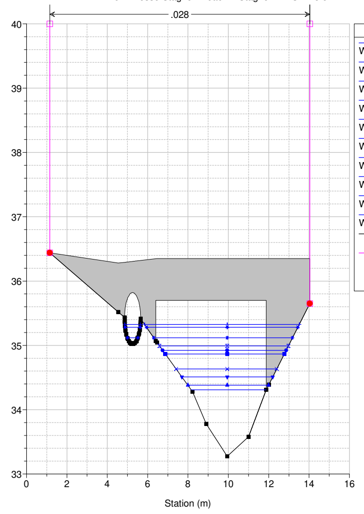
Studio Scandicci Torrenti Greve-Vingone River = Fosso Stagno Reach = Stagno RS = 73.5 BR
