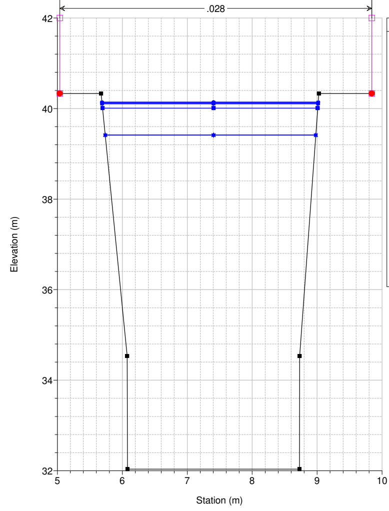
Studio Scandicci Torrenti Greve-Vingone River = Fosso Rigone Reach = Rigone 01 RS = 1 DO1034_E
