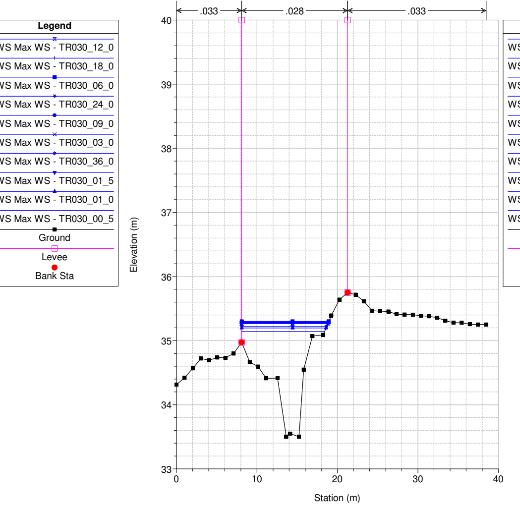
Studio Scandicci Torrenti Greve-Vingone River = Fosso Rigone Reach = Rigone 02 RS = 23.5 BR
