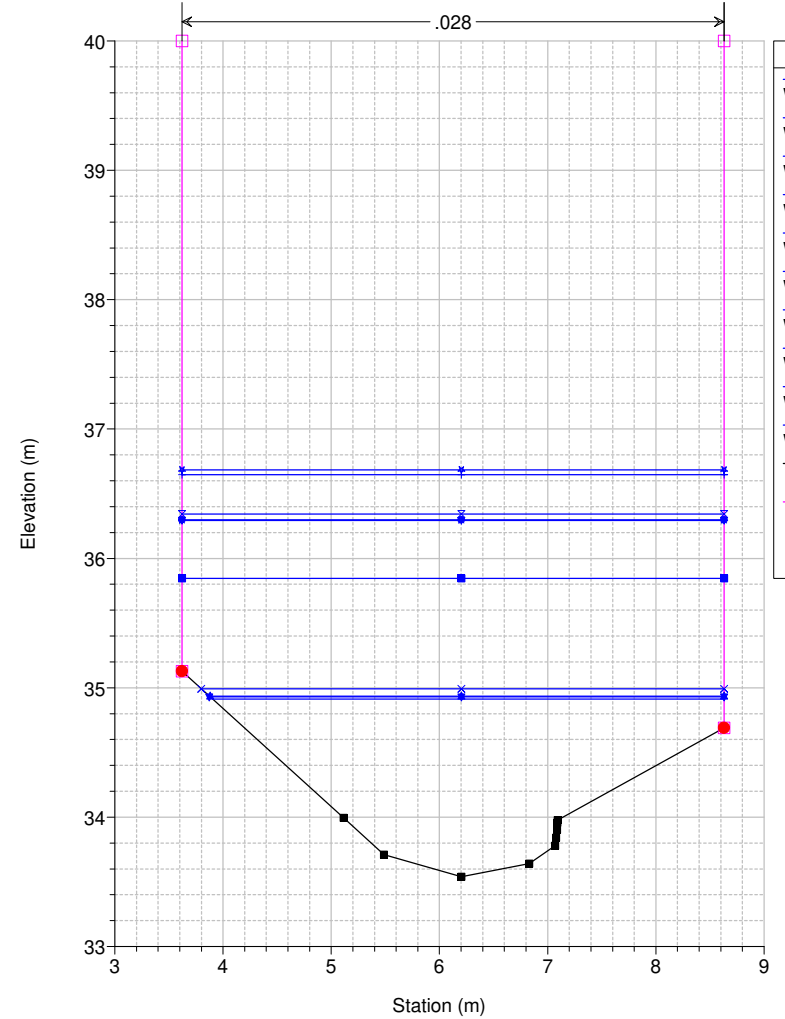
Studio Scandicci Torrenti Greve-Vingone River = Fosso Stagnolo Reach = Stagnolo RS = 92 ST0008_C
