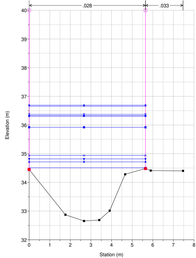
Studio Scandicci Torrenti Greve-Vingone River = Fosso Stagno Reach = Stagno RS = 17 SG0044__
