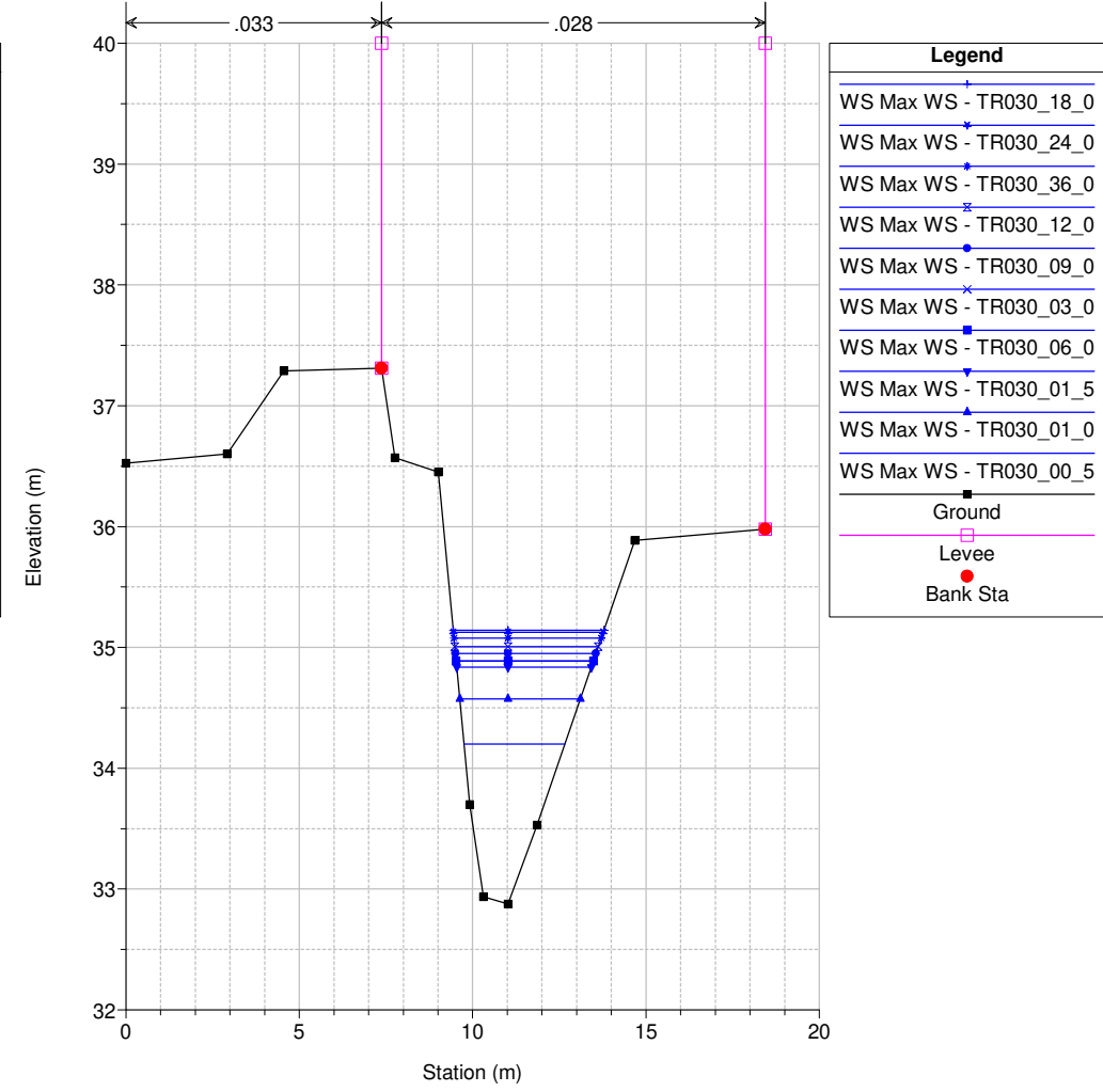
Studio Scandicci Torrenti Greve-Vingone River = Fosso Stagnolo Reach = Stagnolo RS = 8 ST0060_B
