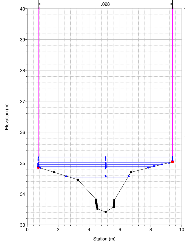
Studio Scandicci Torrenti Greve-Vingone River = Fosso Stagnolo Reach = Stagnolo RS = 62 ST0027_B
