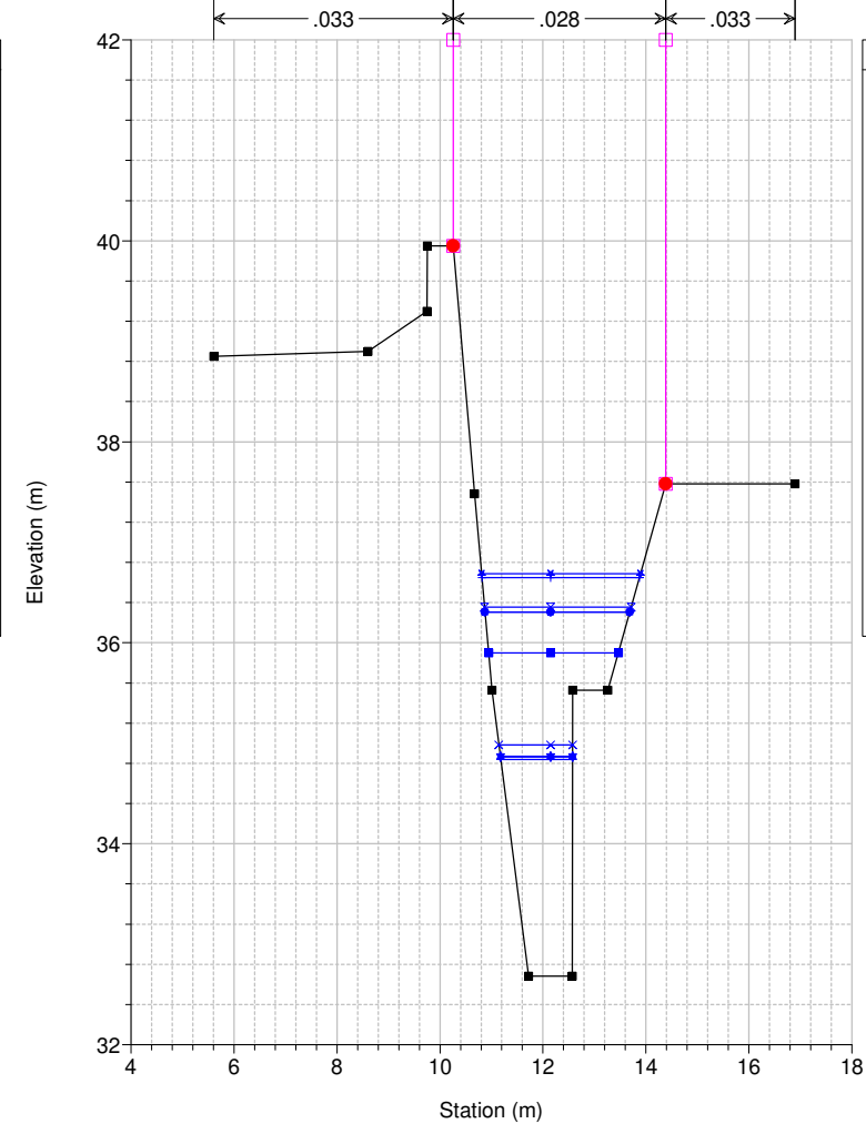
Studio Scandicci Torrenti Greve-Vingone River = Fosso Stagnolo Reach = Stagnolo RS = 8 ST0060_B
