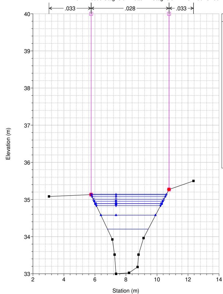
Studio Scandicci Torrenti Greve-Vingone River = Fosso Stagnolo Reach = Stagnolo RS = 30 ST0046_C
