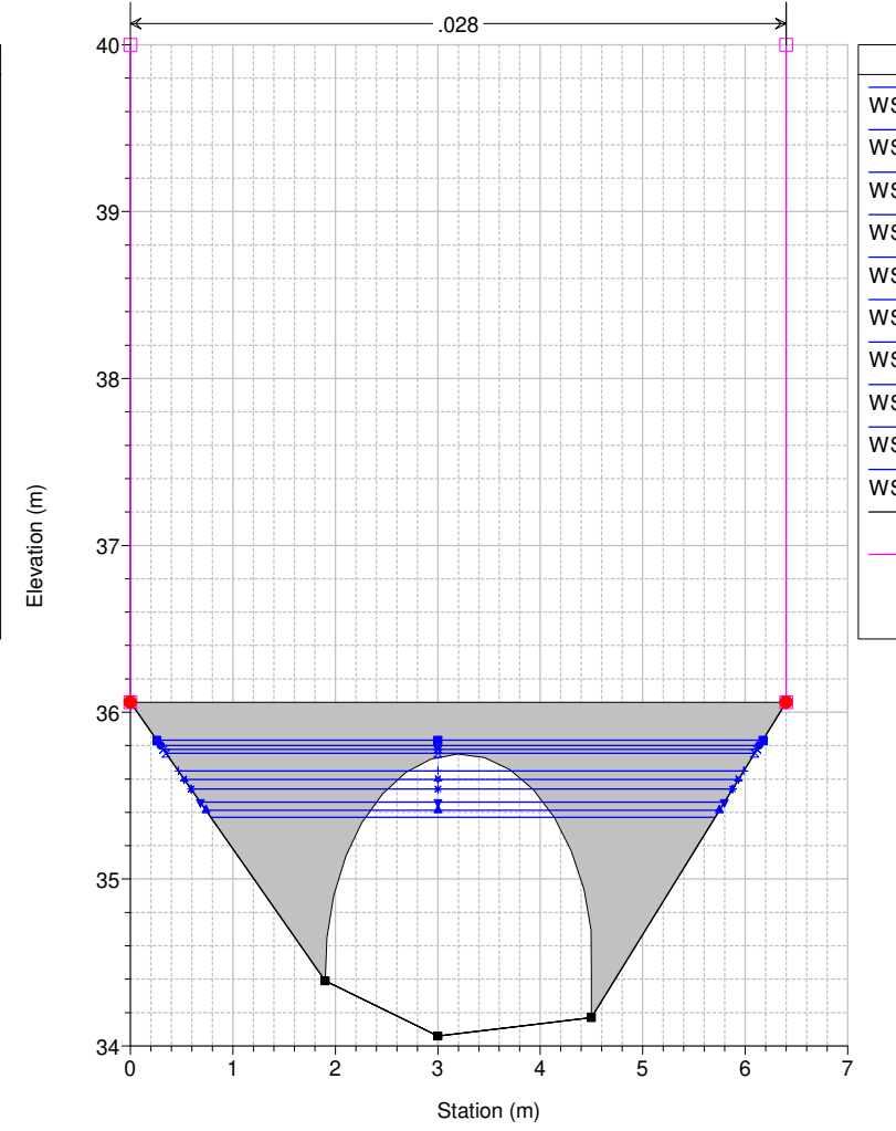
Studio Scandicci Torrenti Greve-Vingone River = Fosso Dogaione Reach = Dogaione RS = 44 DG0010_D
