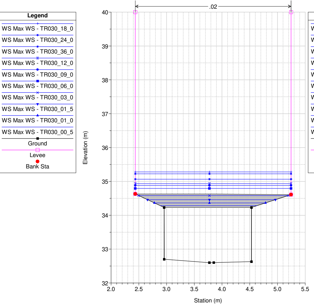
Studio Scandicci Torrenti Greve-Vingone River = Fosso Stagno Reach = Stagno RS = 42 SG0025_
