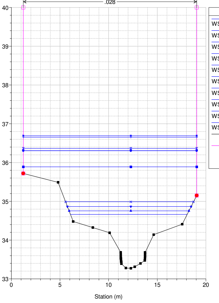
Studio Scandicci Torrenti Greve-Vingone River = Fosso Stagno Reach = Stagno RS = 82 SG0012_B
