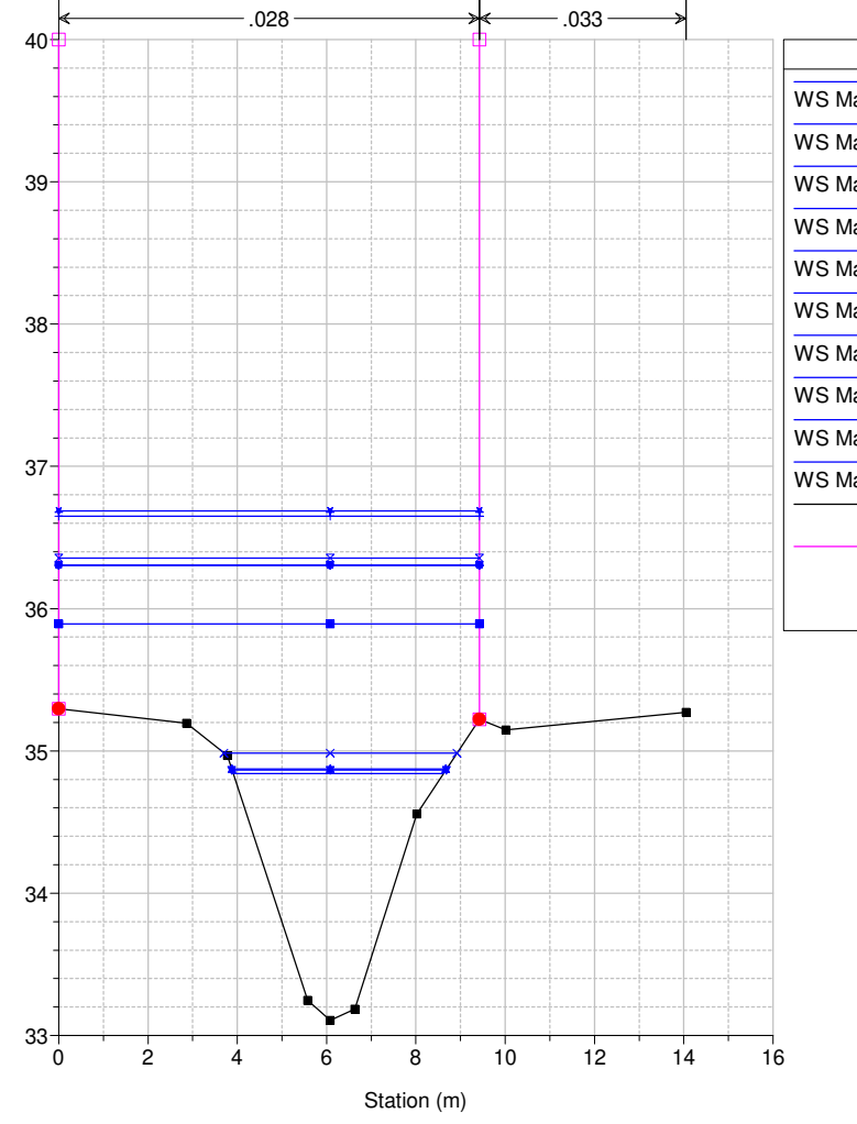
Studio Scandicci Torrenti Greve-Vingone River = Fosso Stagnolo Reach = Stagnolo RS = 33 ST0045_
