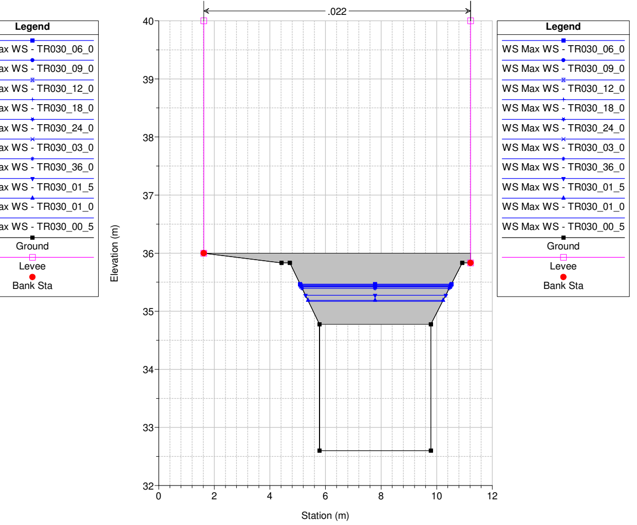
Studio Scandicci Torrenti Greve-Vingone River = Fosso Rigone Reach = Rigone 01 RS = 5 DO1034_A
