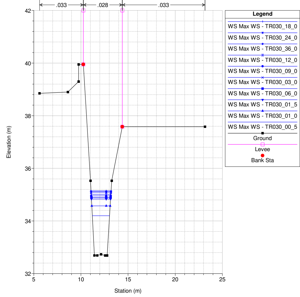
Studio Scandicci Torrenti Greve-Vingone River = Fosso Stagnolo Reach = Stagnolo RS = 9 ST0060_A
