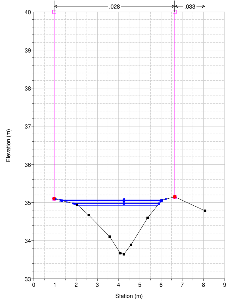
Studio Scandicci Torrenti Greve-Vingone River = Fosso Botteghino Reach = Botteghino RS = 6 SD0003_
