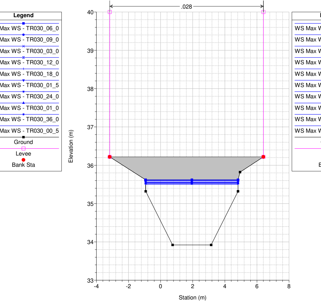
Studio Scandicci Torrenti Greve-Vingone River = Fosso Dogaione Reach = Dogaione RS = 56 DG0007_A
