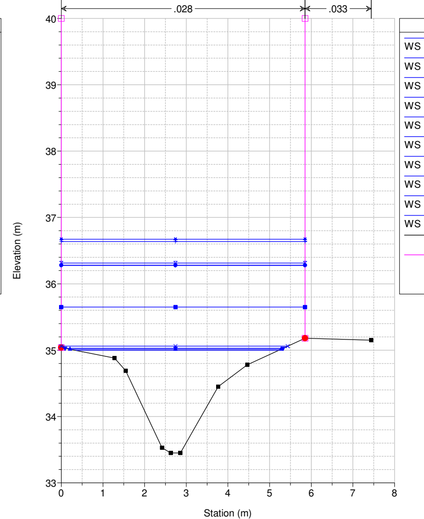
Studio Scandicci Torrenti Greve-Vingone River = Fosso Botteghino Reach = Botteghino RS = 5 SD0002_
