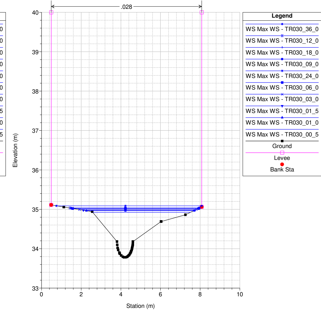
Studio Scandicci Torrenti Greve-Vingone River = Fosso Botteghino Reach = Botteghino RS = 10 SD0006_C
