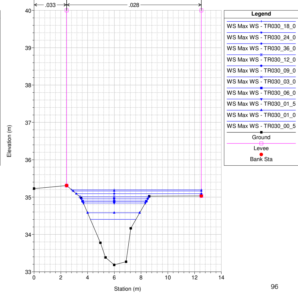
Studio Scandicci Torrenti Greve-Vingone River = Fosso Stagnolo Reach = Stagnolo RS = 56 ST0031__
