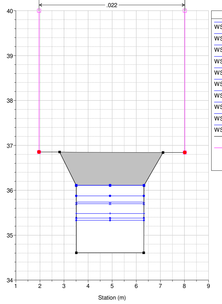
Studio Scandicci Torrenti Greve-Vingone River = Fosso Rigone Reach = Rigone 03 RS = 56.75 Culv
