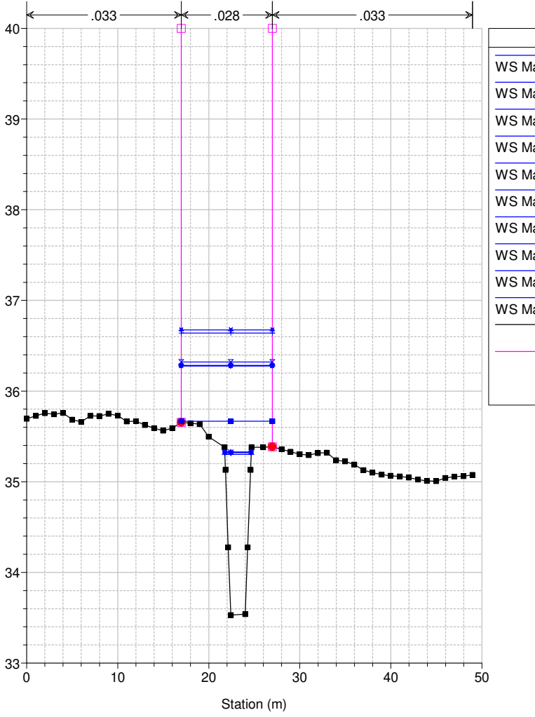
Studio Scandicci Torrenti Greve-Vingone River = Fosso Rigone Reach = Rigone 03 RS = 32 RI0016_C
