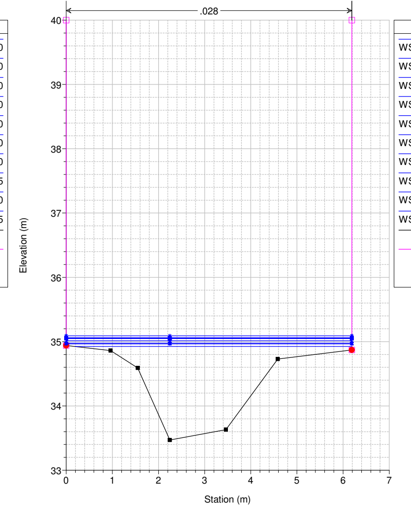
Studio Scandicci Torrenti Greve-Vingone River = Fosso Botteghino Reach = Botteghino RS = 4 SD0001_A
