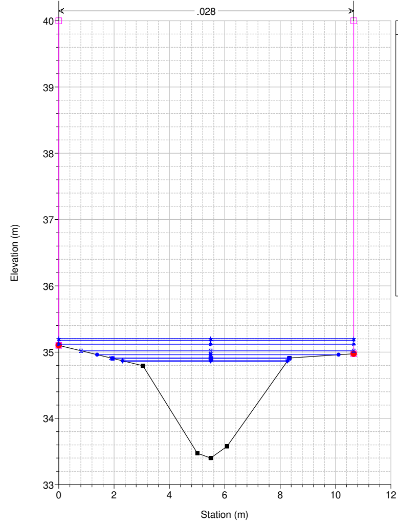
Studio Scandicci Torrenti Greve-Vingone River = Fosso Stagnolo Reach = Stagnolo RS = 86.5 BR
