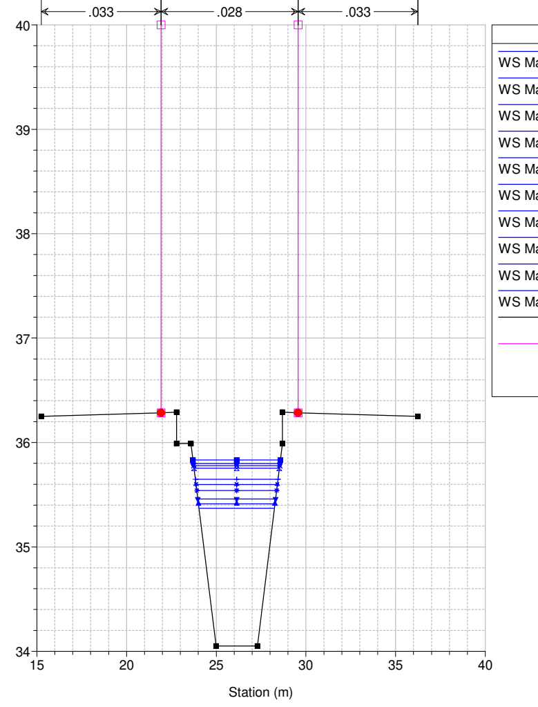
Studio Scandicci Torrenti Greve-Vingone River = Fosso Dogaione Reach = Dogaione RS = 41 DG1011_C
