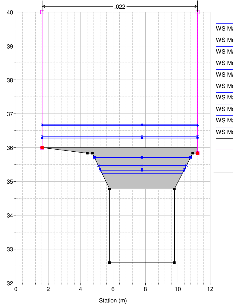
Studio Scandicci Torrenti Greve-Vingone River = Fosso Rigone Reach = Rigone 01 RS = 6 DO1033_D
