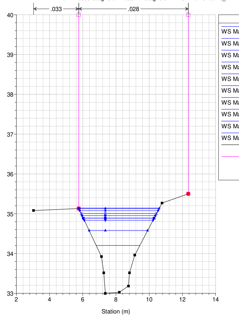
Studio Scandicci Torrenti Greve-Vingone River = Fosso Stagnolo Reach = Stagnolo RS = 29 ST0046_D
