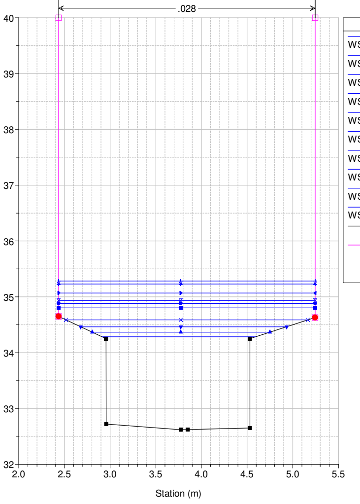
Studio Scandicci Torrenti Greve-Vingone River = Fosso Stagno Reach = Stagno RS = 45 SG0024_T
