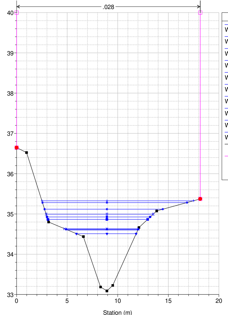
Studio Scandicci Torrenti Greve-Vingone River = Fosso Stagno Reach = Stagno RS = 73.5 BR
