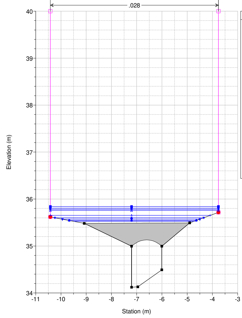
Studio Scandicci Torrenti Greve-Vingone River = Fosso Dogaione Reach = Dogaione RS = 49.5 BR
