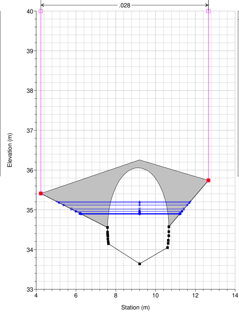
Studio Scandicci Torrenti Greve-Vingone River = Fosso Stagnolo Reach = Stagnolo RS = 98.5 BR
