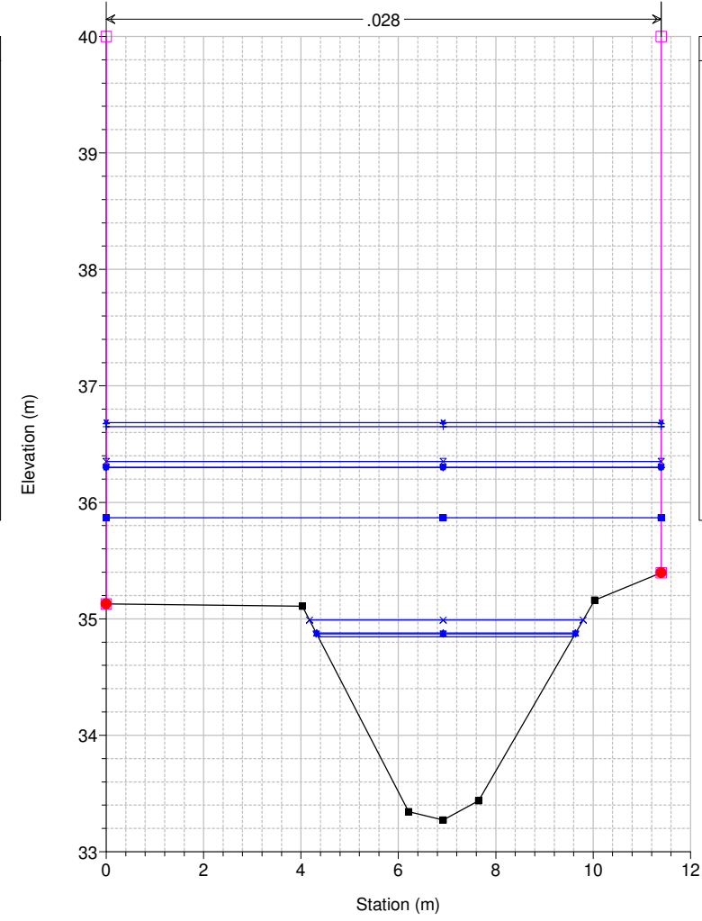
Studio Scandicci Torrenti Greve-Vingone River = Fosso Stagnolo Reach = Stagnolo RS = 70.5 BR
