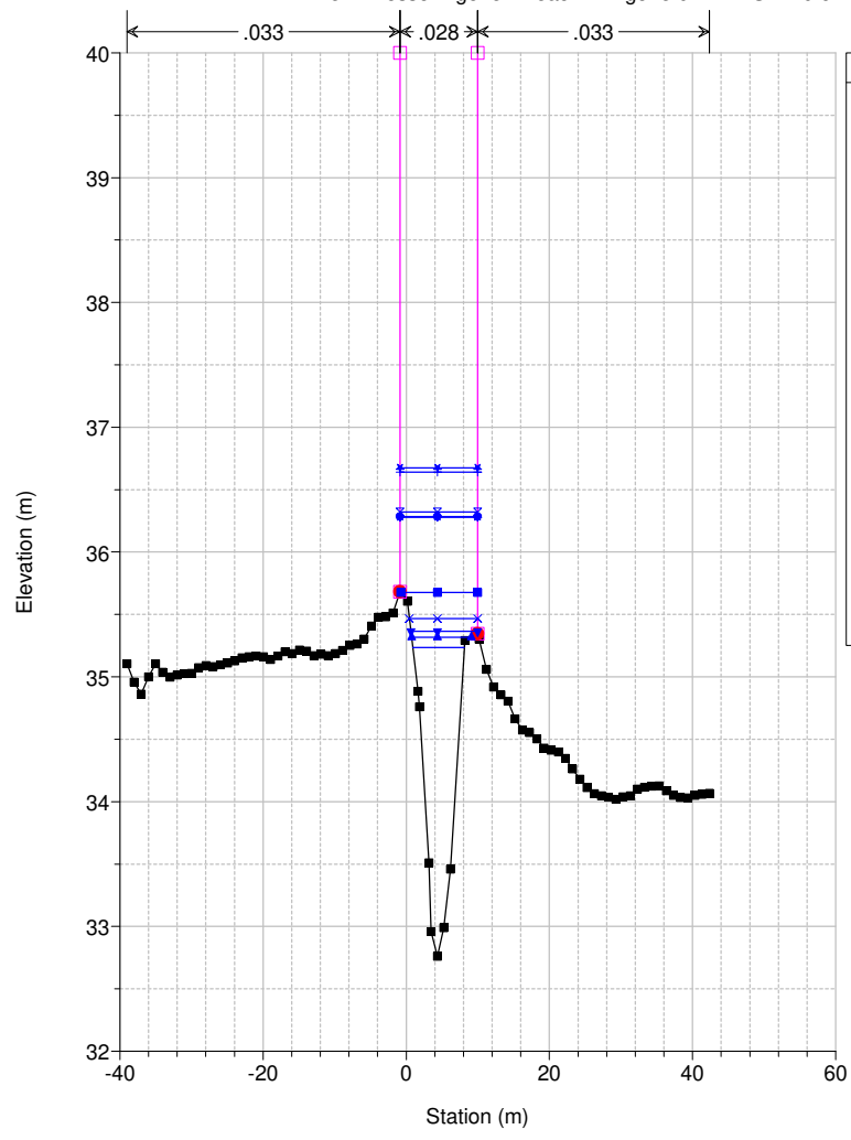
Studio Scandicci Torrenti Greve-Vingone River = Fosso Rigone Reach = Rigone 02 RS = 10.6
