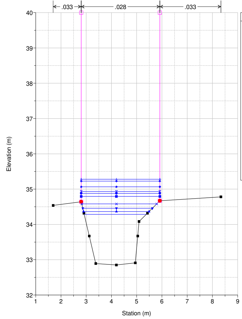
Studio Scandicci Torrenti Greve-Vingone River = Fosso Stagno Reach = Stagno RS = 27 SG0038_C
