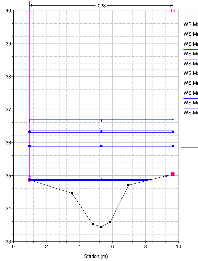
Studio Scandicci Torrenti Greve-Vingone River = Fosso Stagnolo Reach = Stagnolo RS = 57 ST0030__
