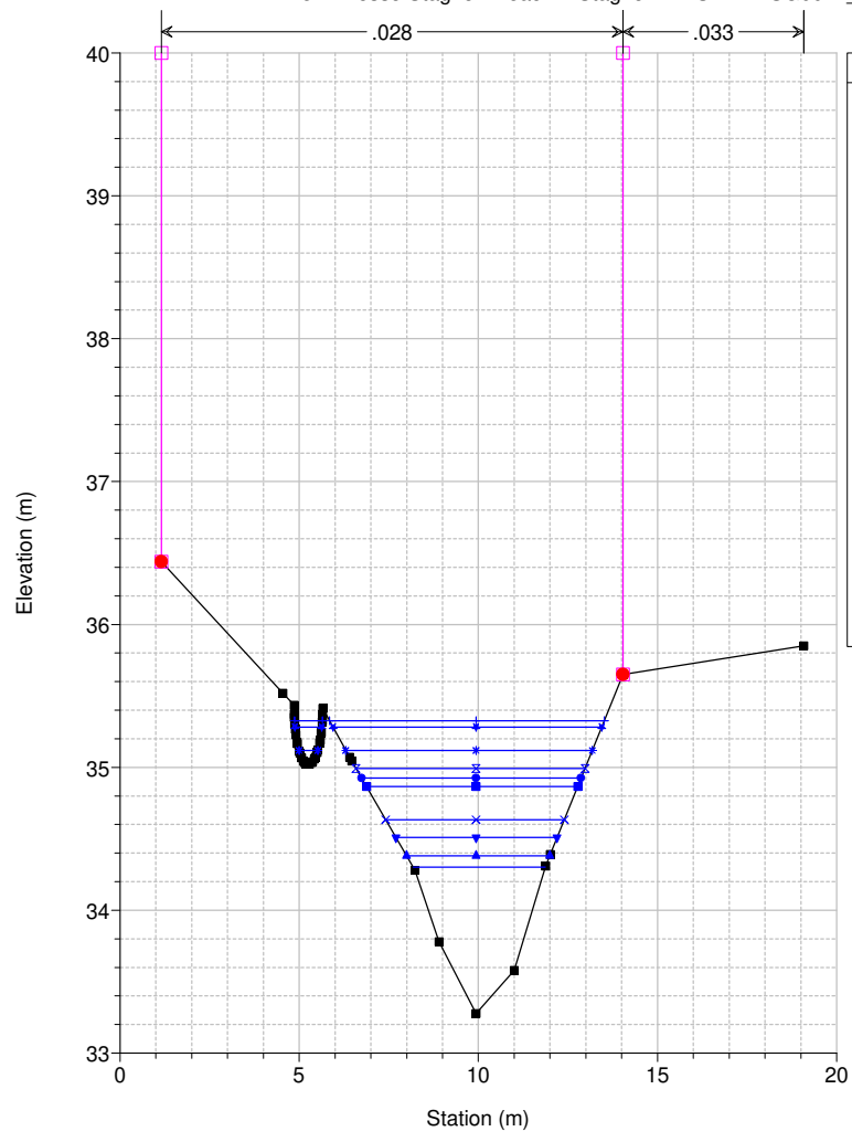
Studio Scandicci Torrenti Greve-Vingone River = Fosso Stagno Reach = Stagno RS = 74 SG0017_B
