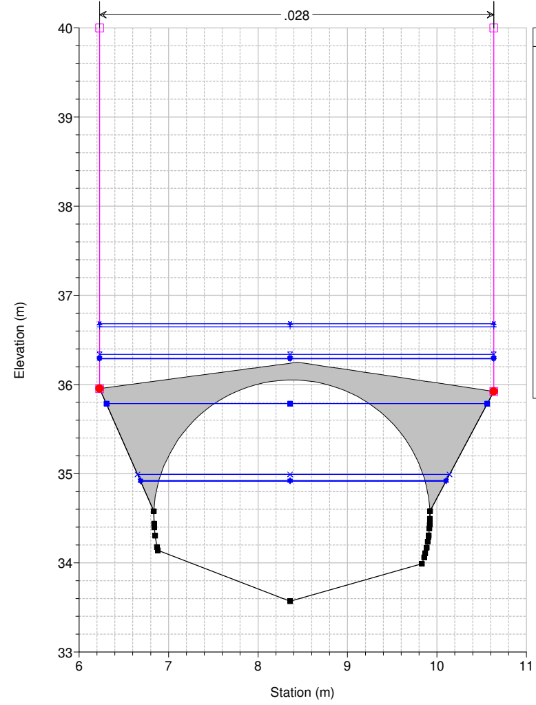
Studio Scandicci Torrenti Greve-Vingone River = Fosso Stagnolo Reach = Stagnolo RS = 96 ST0006_
