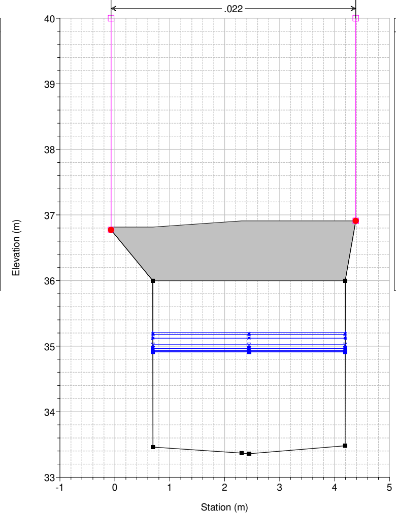
Studio Scandicci Torrenti Greve-Vingone River = Fosso Stagnolo Reach = Stagnolo RS = 102.5 BR
