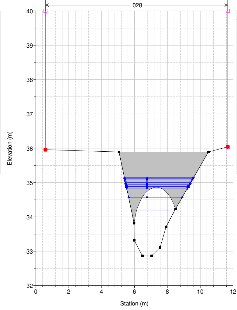
Studio Scandicci Torrenti Greve-Vingone River = Fosso Stagnolo Reach = Stagnolo RS = 13.5 BR
