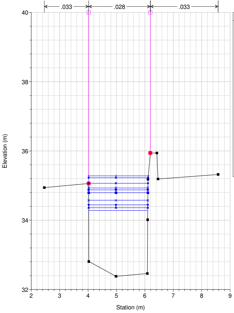
Studio Scandicci Torrenti Greve-Vingone River = Fosso Stagno Reach = Stagno RS = 7 SG0049_C
