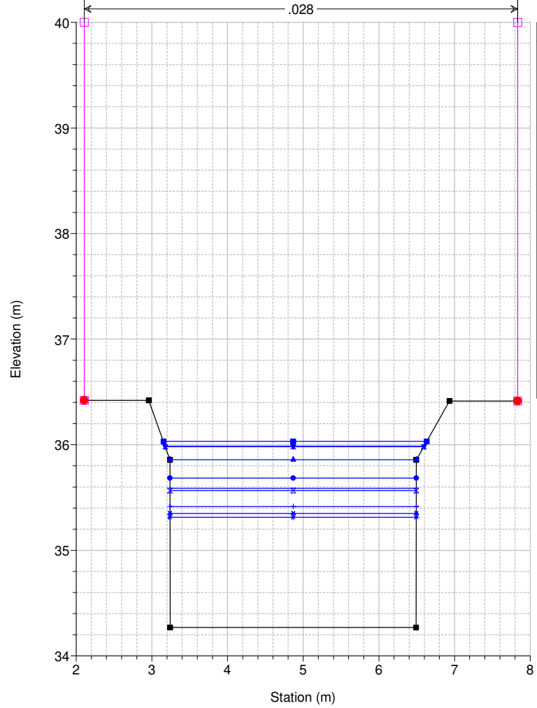
Studio Scandicci Torrenti Greve-Vingone River = Fosso Rigone Reach = Rigone 03 RS = 55 RI0006_A
