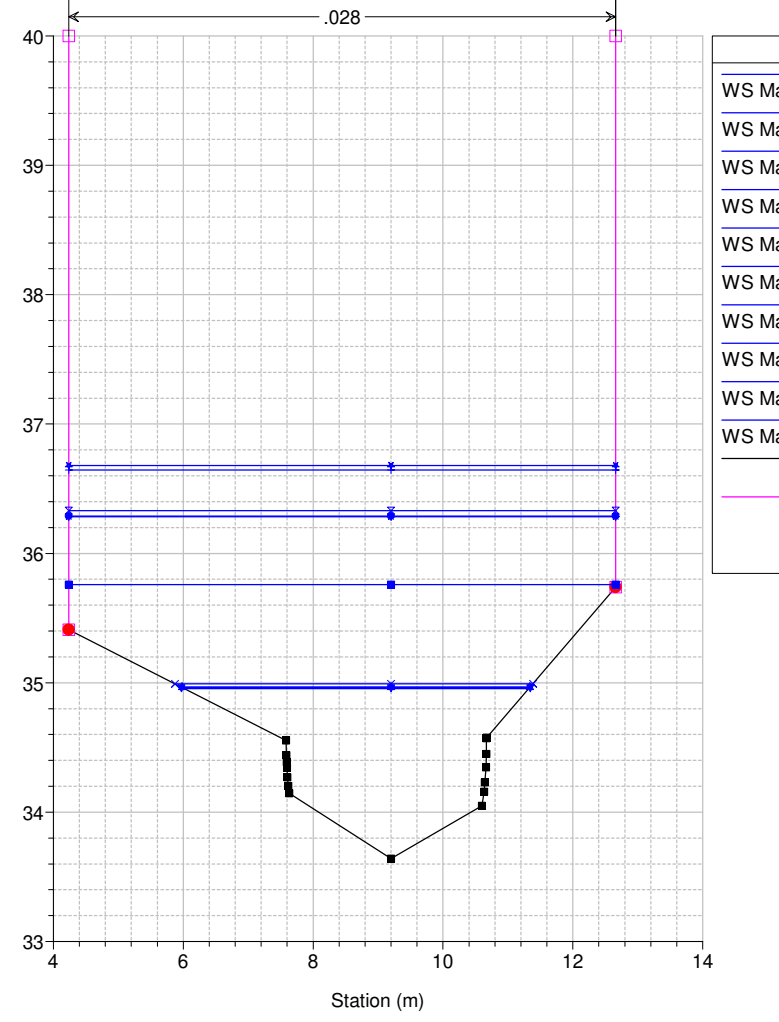
Studio Scandicci Torrenti Greve-Vingone River = Fosso Stagnolo Reach = Stagnolo RS = 99 ST0005_B
