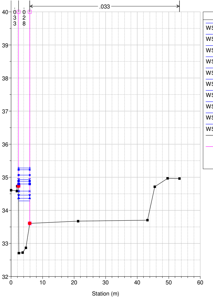
Studio Scandicci Torrenti Greve-Vingone River = Fosso Stagno Reach = Stagno RS = 29 SG0038_A
