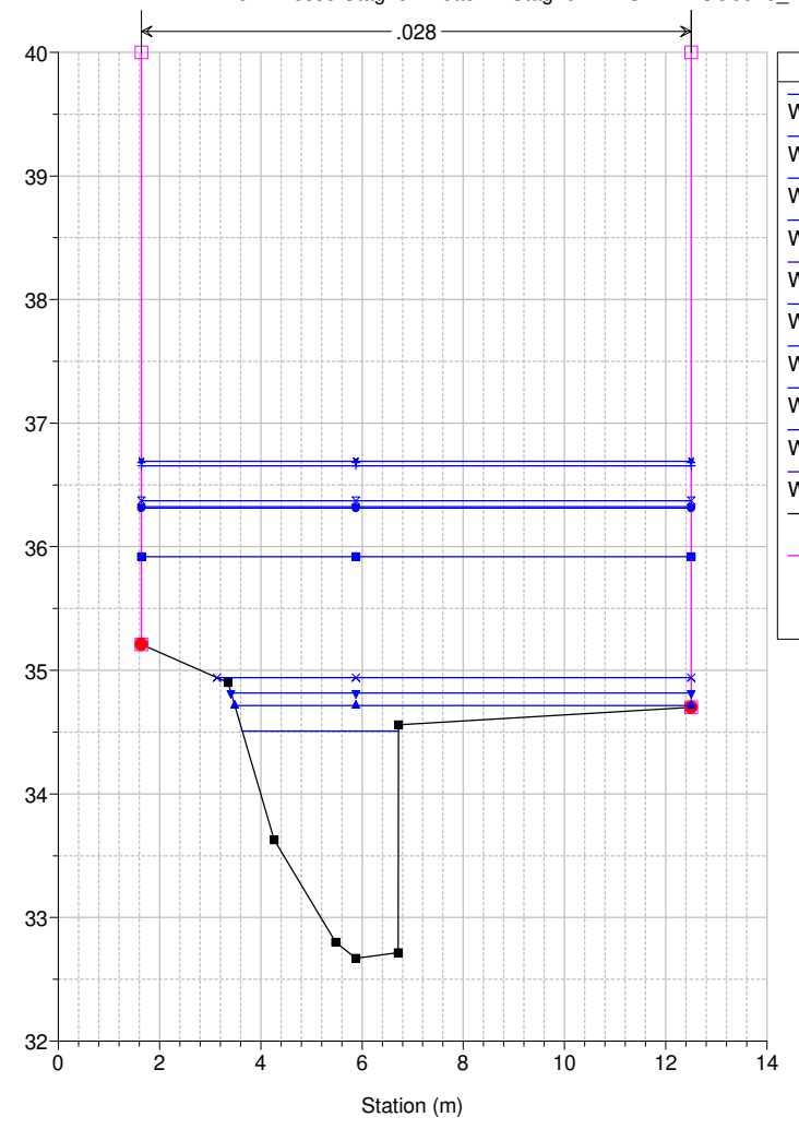
Studio Scandicci Torrenti Greve-Vingone River = Fosso Stagno Reach = Stagno RS = 12 SG0046_D
