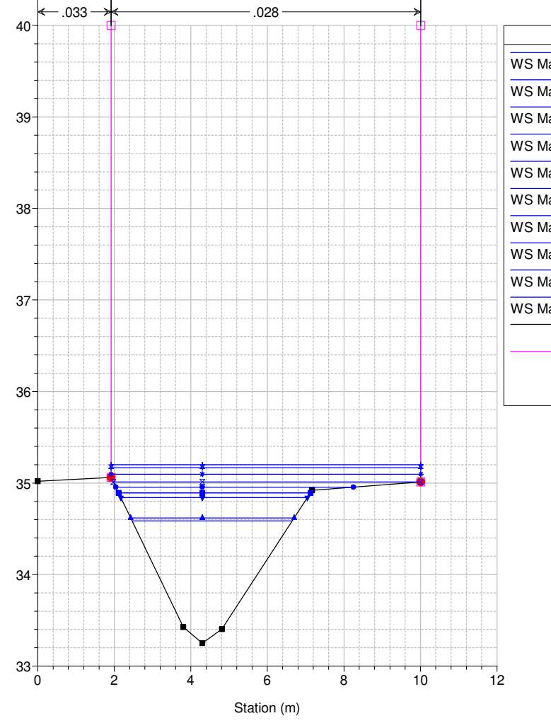
Studio Scandicci Torrenti Greve-Vingone River = Fosso Stagnolo Reach = Stagnolo RS = 67 ST0023_
