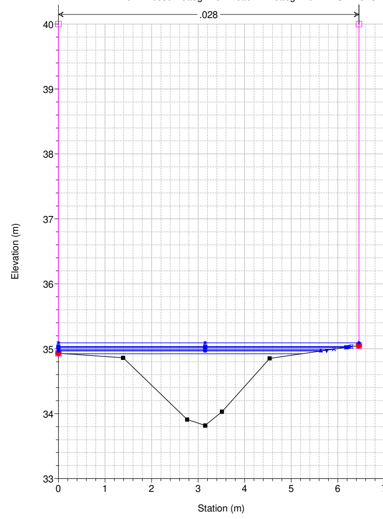
Studio Scandicci Torrenti Greve-Vingone River = Fosso Botteghino Reach = Botteghino RS = 15 SD0009_
