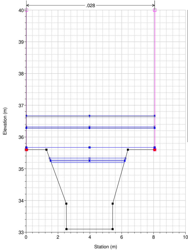
Studio Scandicci Torrenti Greve-Vingone River = Fosso Rigone Reach = Rigone 02 RS = 12.4
