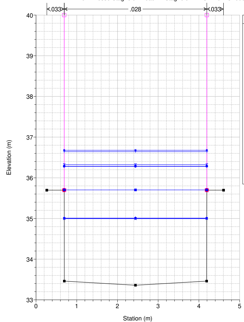
Studio Scandicci Torrenti Greve-Vingone River = Fosso Stagnolo Reach = Stagnolo RS = 104 ST0004_A
