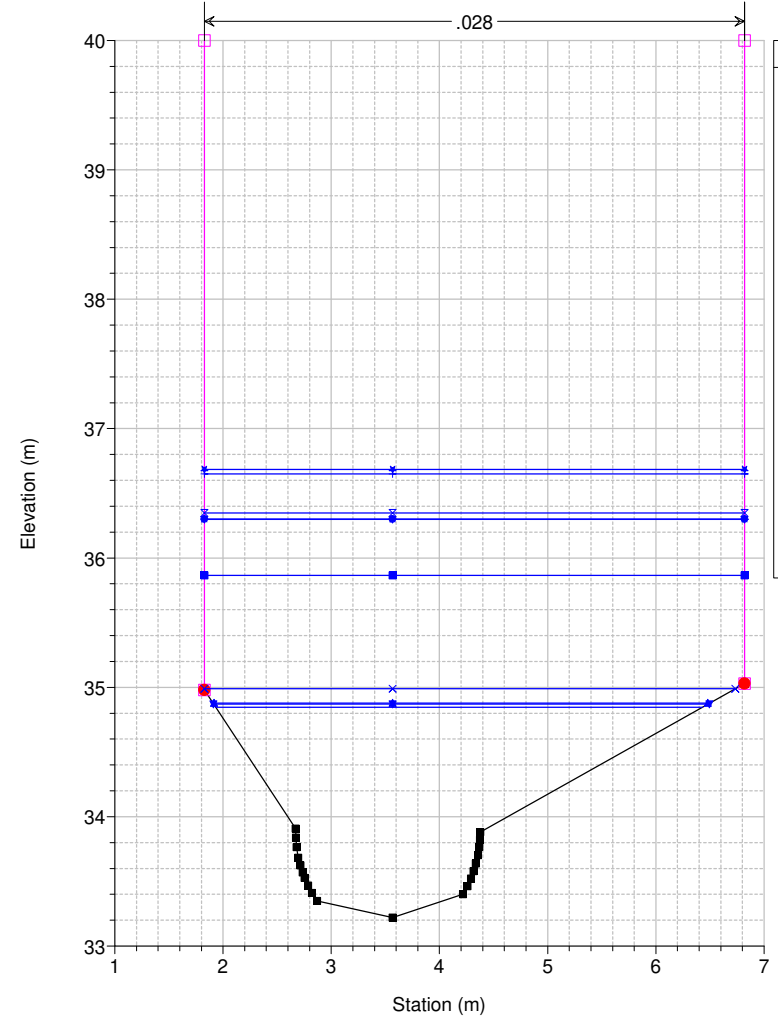
Studio Scandicci Torrenti Greve-Vingone River = Fosso Stagnolo Reach = Stagnolo RS = 72 ST0021_A
