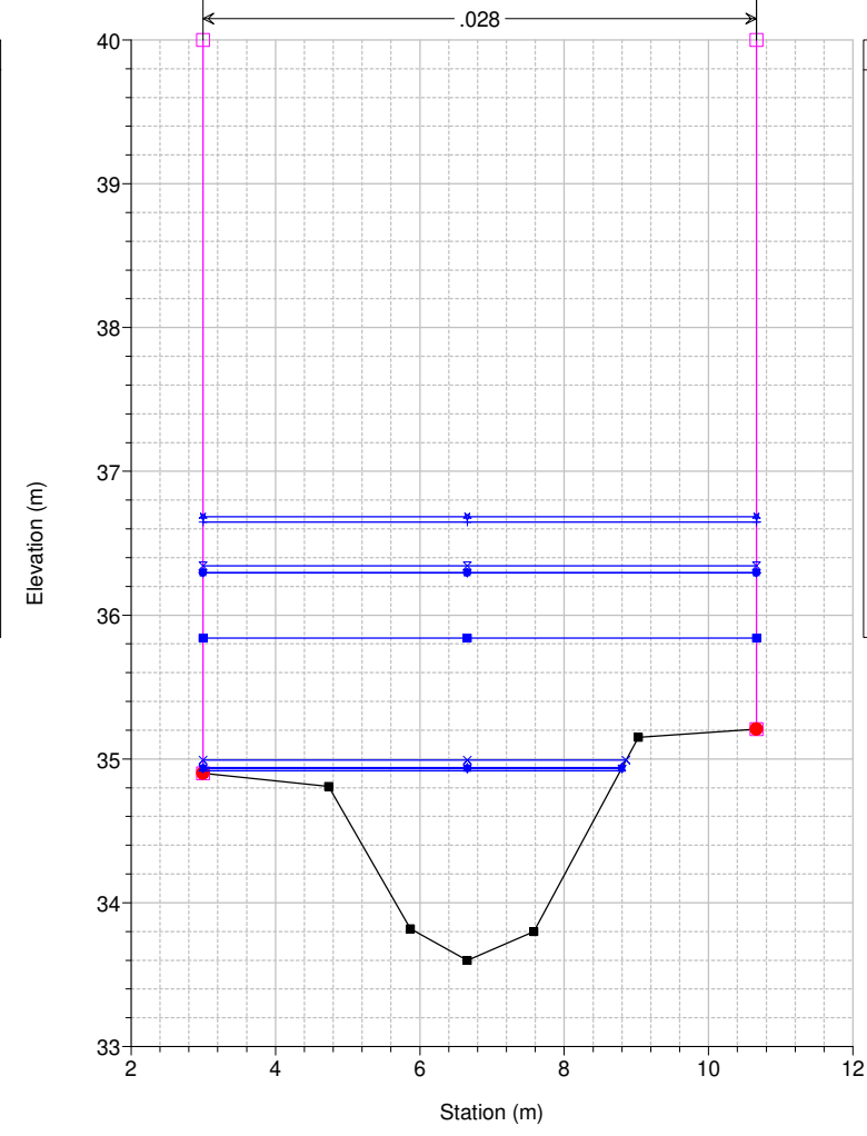
Studio Scandicci Torrenti Greve-Vingone River = Fosso Stagnolo Reach = Stagnolo RS = 94 ST0008_A
