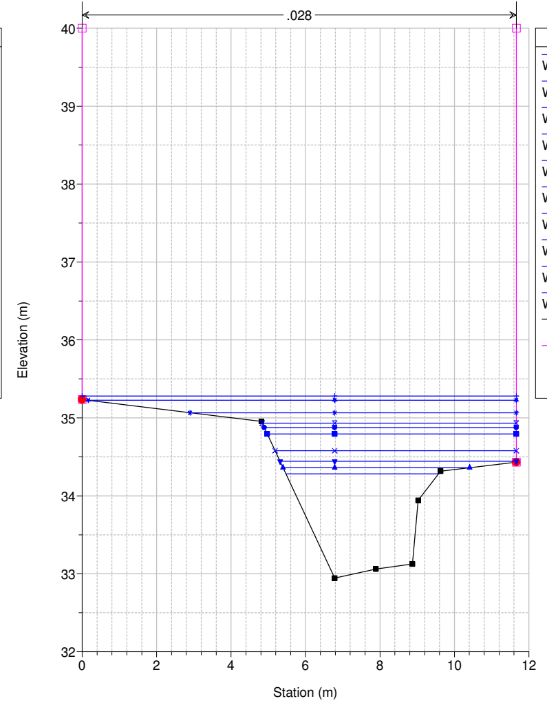
Studio Scandicci Torrenti Greve-Vingone River = Fosso Stagno Reach = Stagno RS = 16 SG0045__
