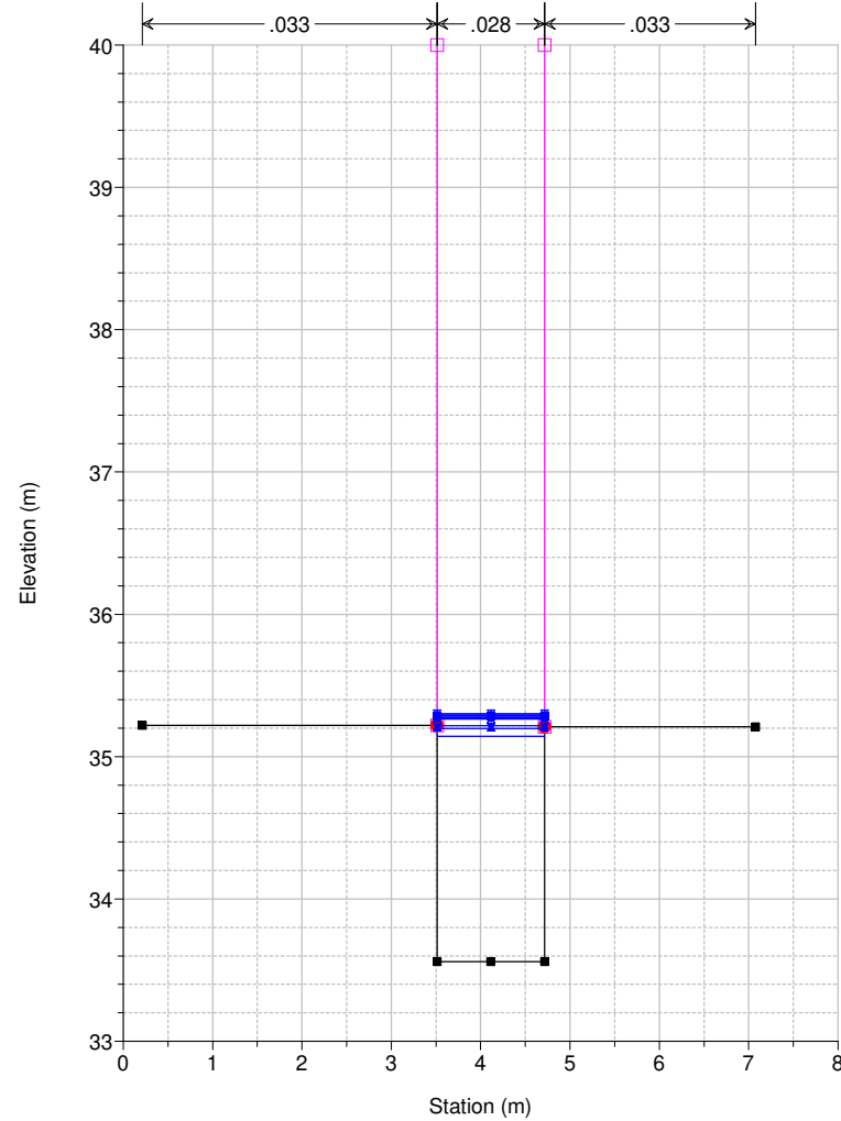
Studio Scandicci Torrenti Greve-Vingone River = Fosso Stagnacci Reach = Stagnacci RS = 4 SR0003_C
