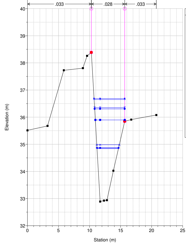
Studio Scandicci Torrenti Greve-Vingone River = Fosso Stagnolo Reach = Stagnolo RS = 10 ST0059__
