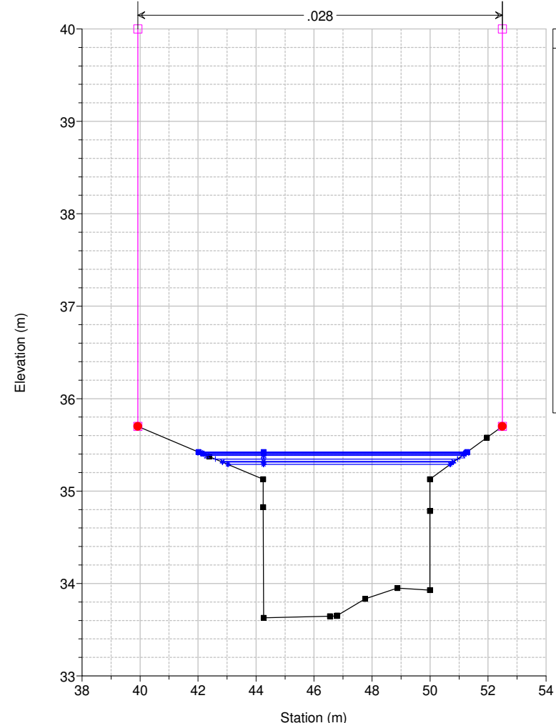
Studio Scandicci Torrenti Greve-Vingone River = Fosso Rigone Reach = Rigone 03 RS = 42 RI1011_C
