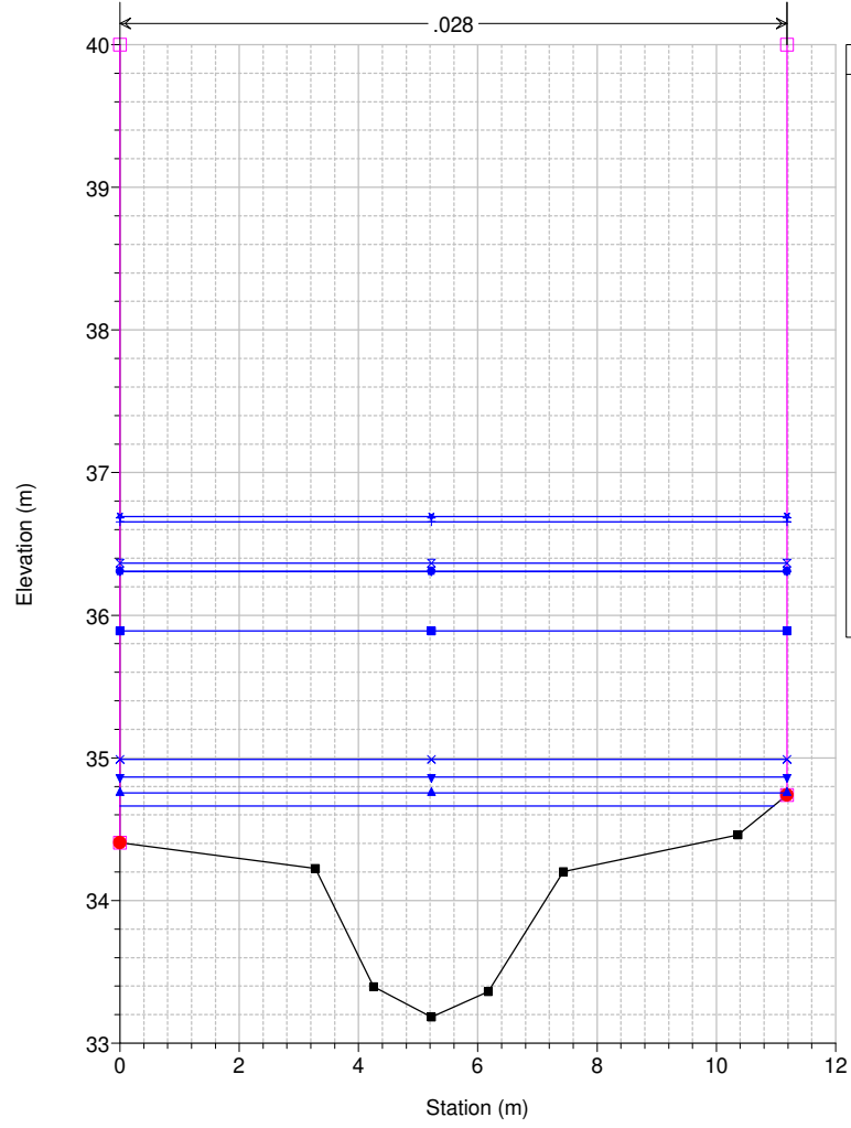
Studio Scandicci Torrenti Greve-Vingone River = Fosso Stagno Reach = Stagno RS = 84 SG0011
