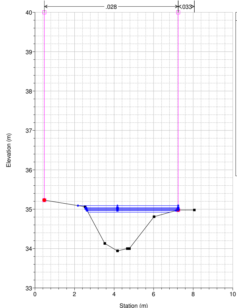
Studio Scandicci Torrenti Greve-Vingone River = Fosso Botteghino Reach = Botteghino RS = 16 SD0010_
