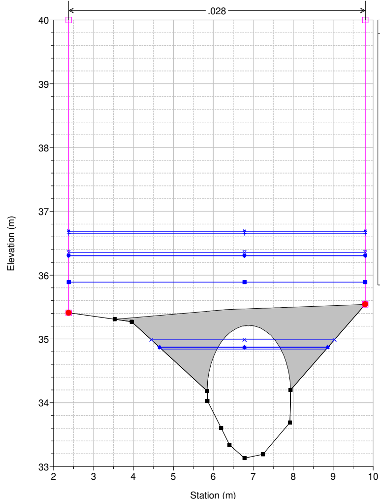
Studio Scandicci Torrenti Greve-Vingone River = Fosso Stagnolo Reach = Stagnolo RS = 38 ST0043_
