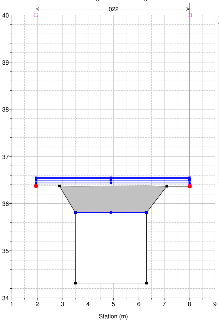
Studio Scandicci Torrenti Greve-Vingone River = Fosso Rigone Reach = Rigone 03 RS = 56.75 Culv
