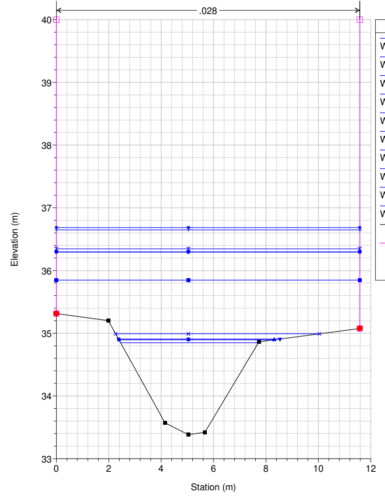
Studio Scandicci Torrenti Greve-Vingone River = Fosso Stagnolo Reach = Stagnolo RS = 81 ST0015_
