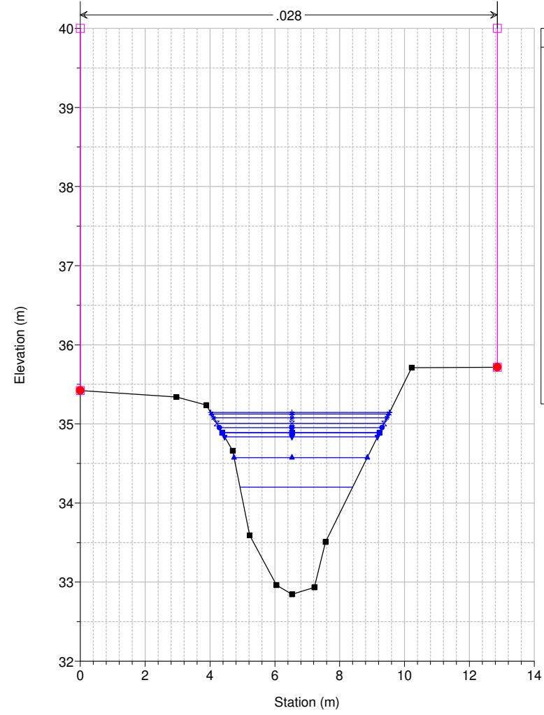
Studio Scandicci Torrenti Greve-Vingone River = Fosso Stagnolo Reach = Stagnolo RS = 14 ST0057_B
