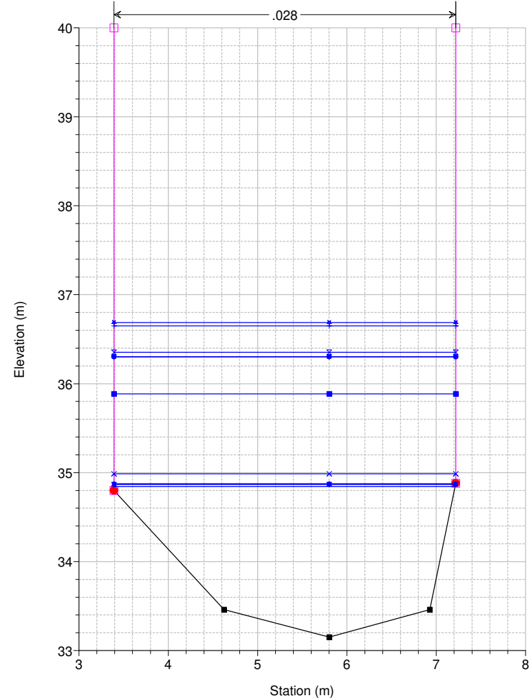
Studio Scandicci Torrenti Greve-Vingone River = Fosso Stagnolo Reach = Stagnolo RS = 48 ST0037_C
