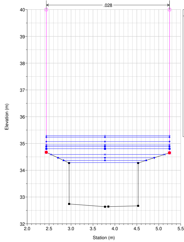
Studio Scandicci Torrenti Greve-Vingone River = Fosso Stagno Reach = Stagno RS = 45.75 BR
