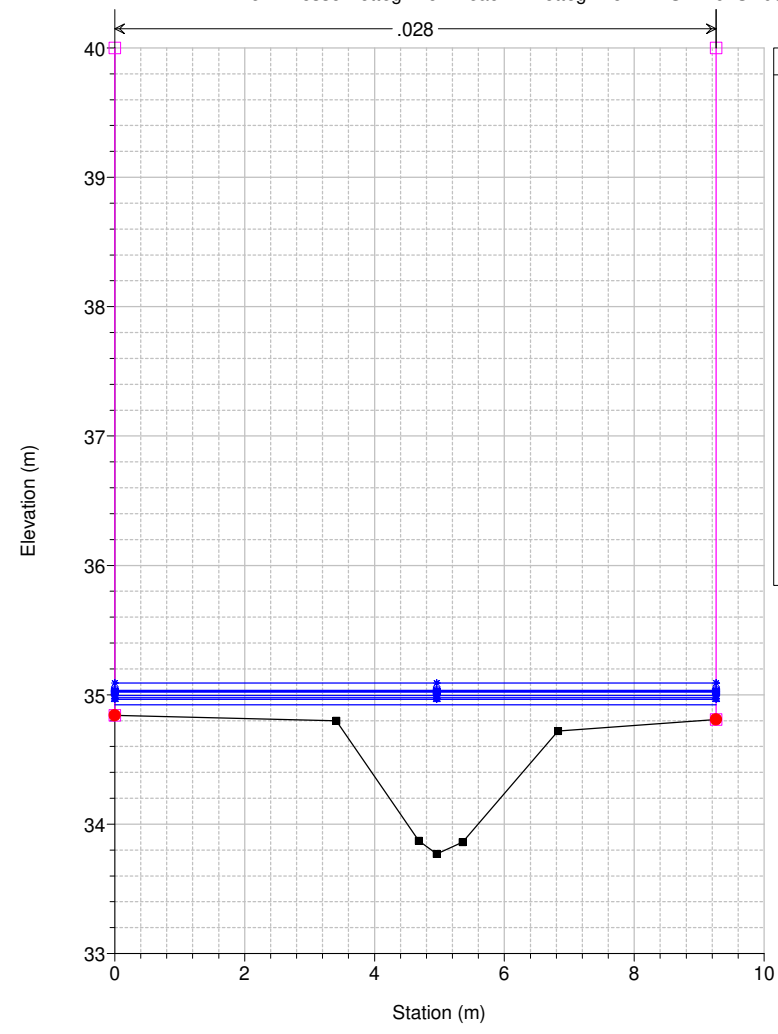
Studio Scandicci Torrenti Greve-Vingone River = Fosso Botteghino Reach = Botteghino RS = 16 SD0010_
