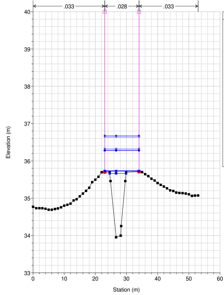
Studio Scandicci Torrenti Greve-Vingone River = Fosso Rigone Reach = Rigone 03 RS = 50 RI0007_B
