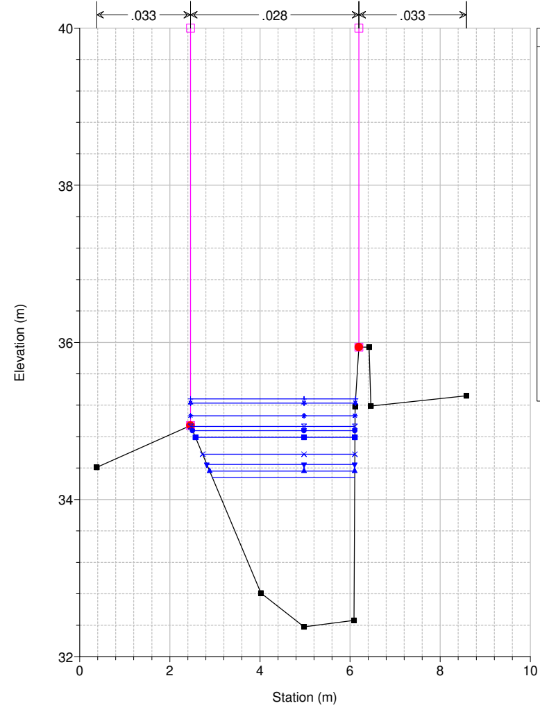
Studio Scandicci Torrenti Greve-Vingone River = Fosso Stagno Reach = Stagno RS = 3 SG0052_A
