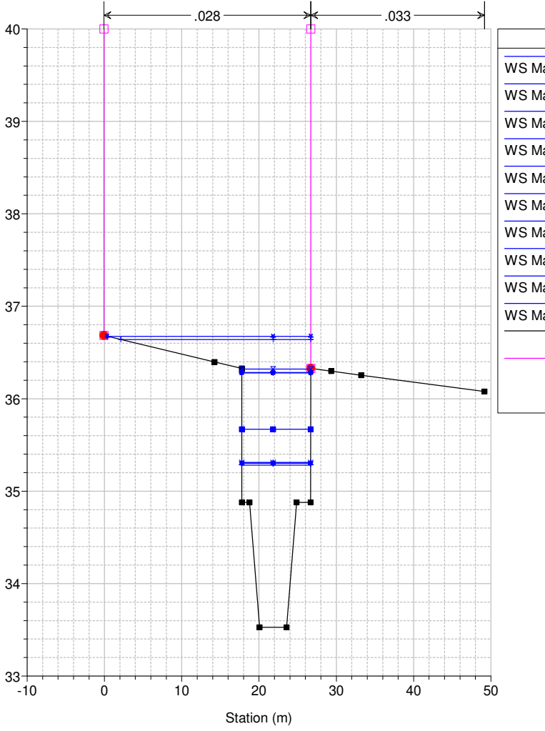
Studio Scandicci Torrenti Greve-Vingone River = Fosso Rigone Reach = Rigone 03 RS = 28 RI1016_C
