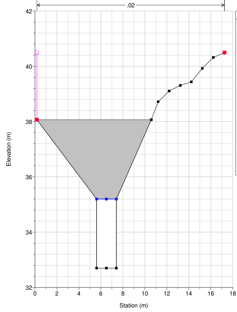
Studio Scandicci Torrenti Greve-Vingone River = Fosso Dogaione Reach = Dogaione RS = 2.75 Culv
