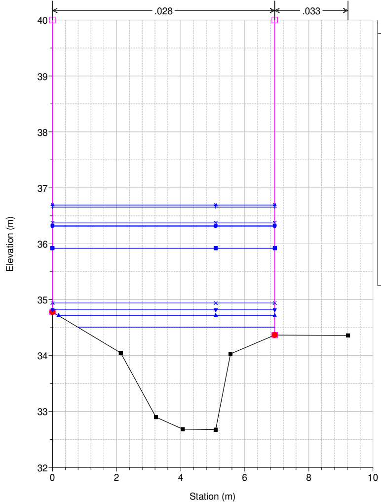
Studio Scandicci Torrenti Greve-Vingone River = Fosso Stagno Reach = Stagno RS = 16 SG0045__
