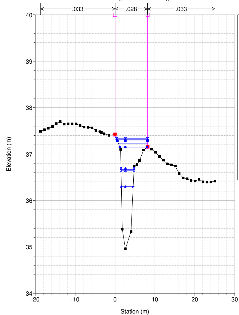
Studio Scandicci Torrenti Greve-Vingone River = Fosso Rigone Reach = Rigone 03 RS = 60 RI0004_
