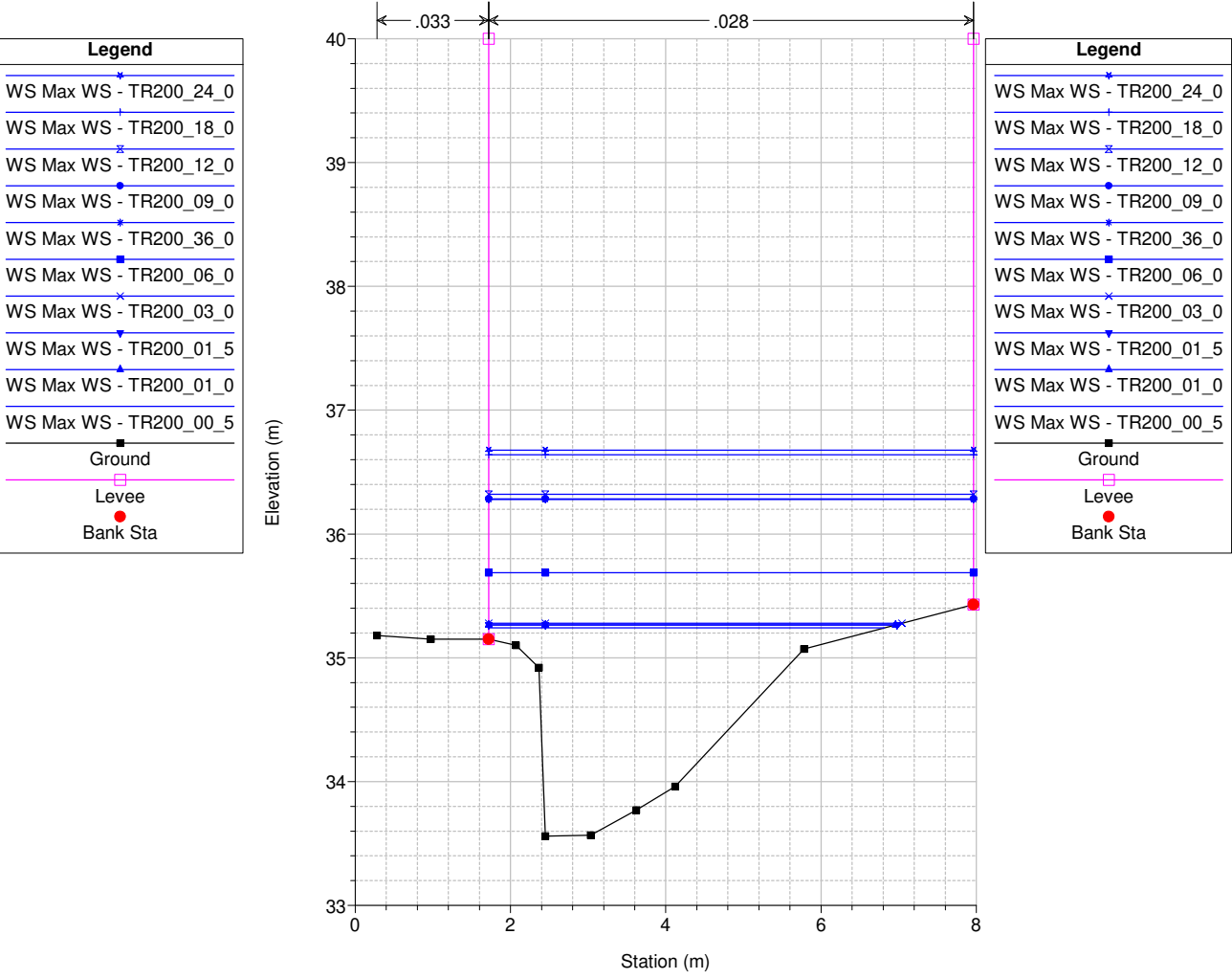
Studio Scandicci Torrenti Greve-Vingone River = Fosso Stagnacci Reach = Stagnacci RS = 4.5 BR
