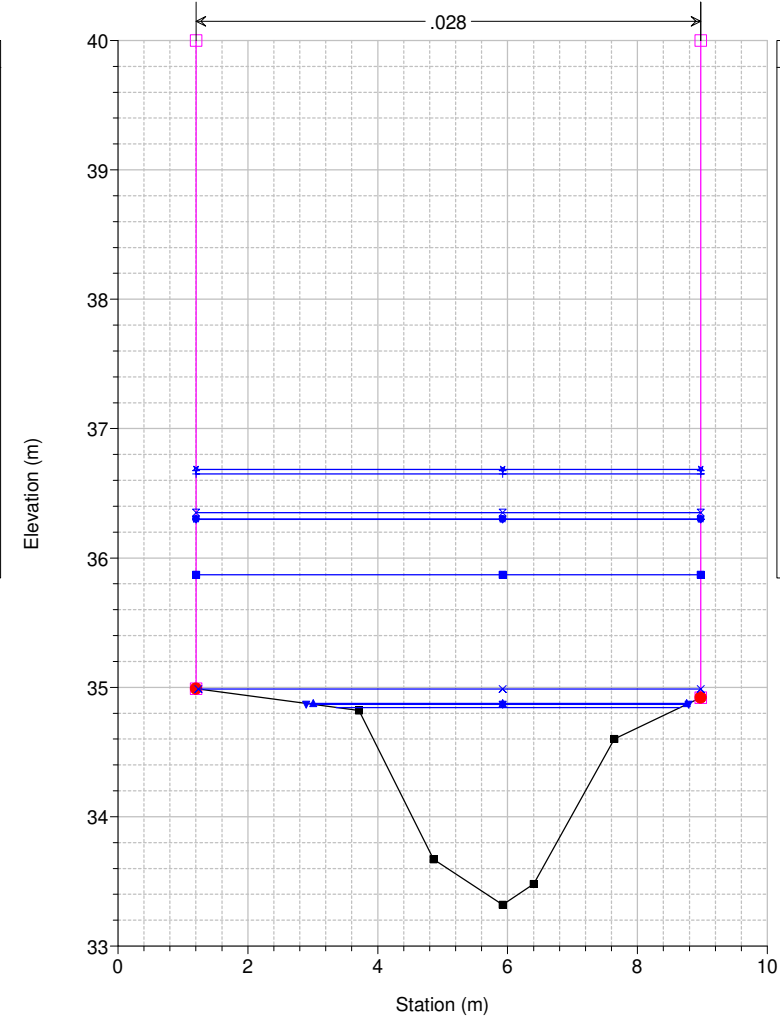
Studio Scandicci Torrenti Greve-Vingone River = Fosso Stagnolo Reach = Stagnolo RS = 66 ST0024__
