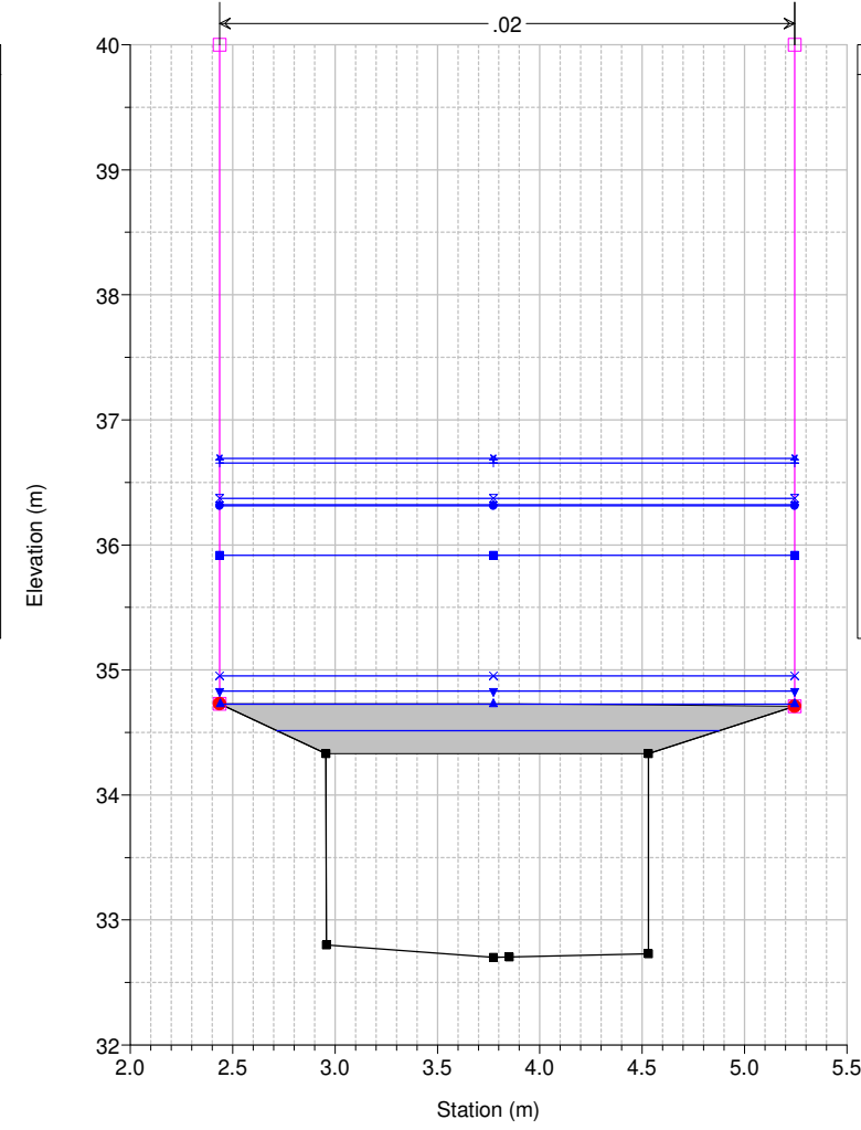
Studio Scandicci Torrenti Greve-Vingone River = Fosso Stagno Reach = Stagno RS = 48 SG0024_Q
