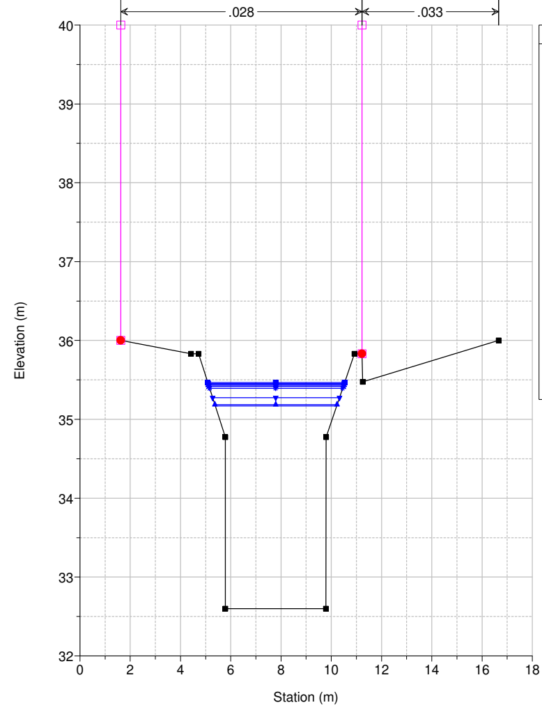
Studio Scandicci Torrenti Greve-Vingone River = Fosso Rigone Reach = Rigone 01 RS = 7 DO1033_C
