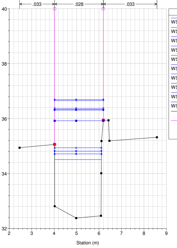
Studio Scandicci Torrenti Greve-Vingone River = Fosso Stagno Reach = Stagno RS = 7 SG0049_C
