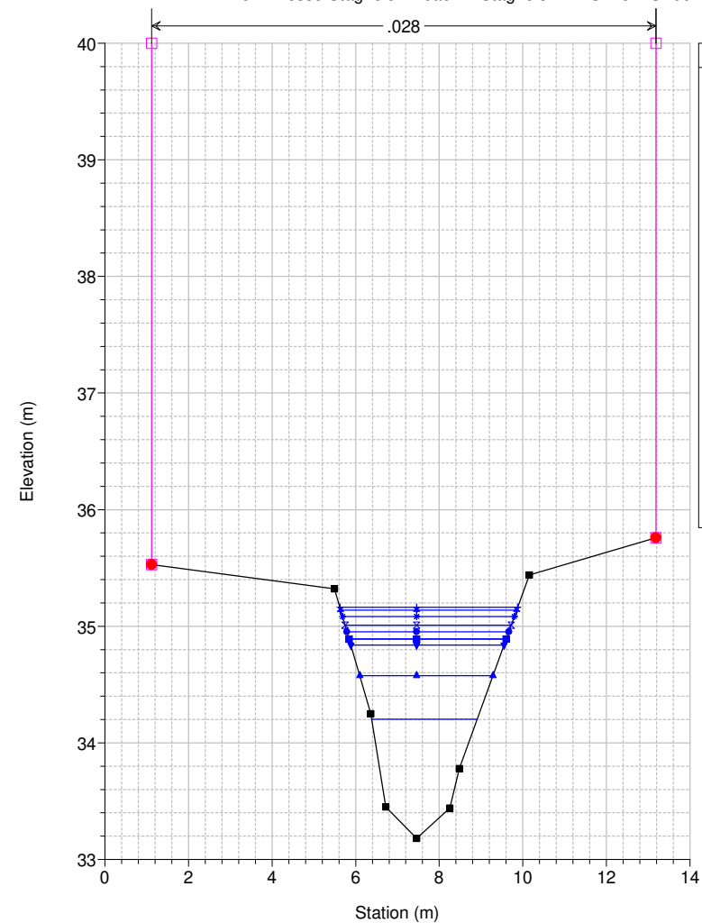
Studio Scandicci Torrenti Greve-Vingone River = Fosso Stagnolo Reach = Stagnolo RS = 37 ST0044_A
