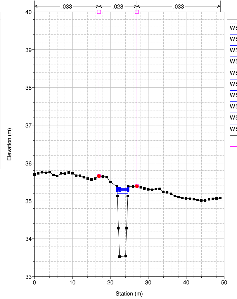
Studio Scandicci Torrenti Greve-Vingone River = Fosso Rigone Reach = Rigone 03 RS = 32 RI0016_C
