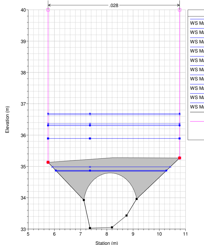
Studio Scandicci Torrenti Greve-Vingone River = Fosso Stagnolo Reach = Stagnolo RS = 29 ST0046_D
