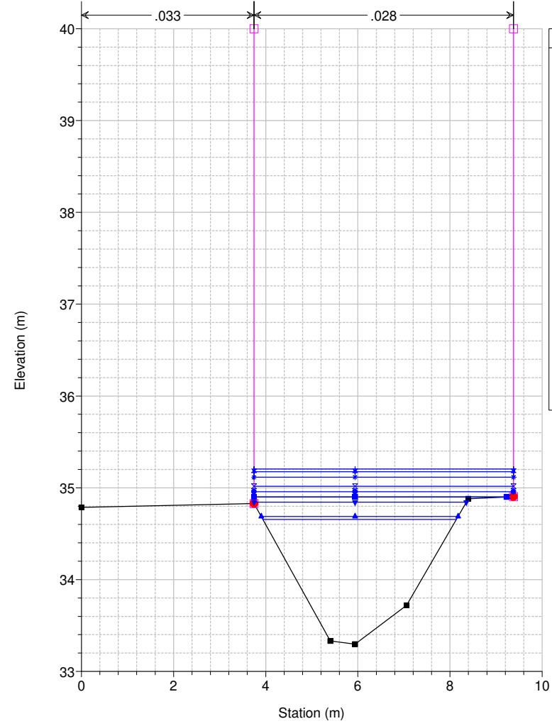
Studio Scandicci Torrenti Greve-Vingone River = Fosso Stagnolo Reach = Stagnolo RS = 76 ST0019_B
