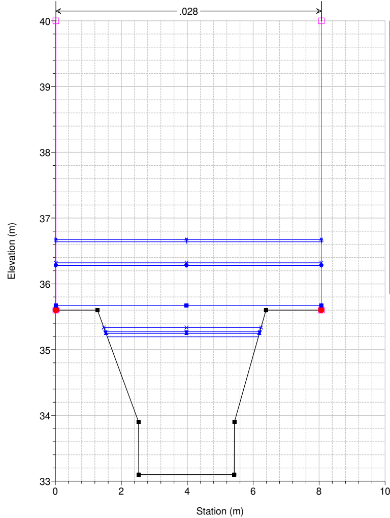
Studio Scandicci Torrenti Greve-Vingone River = Fosso Rigone Reach = Rigone 02 RS = 12 RI0022_B
