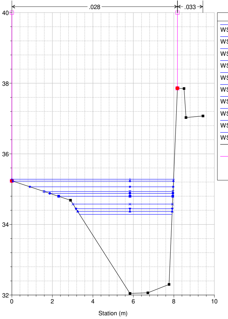
Studio Scandicci Torrenti Greve-Vingone River = Fosso Stagno Reach = Stagno RS = 1.5 IS
