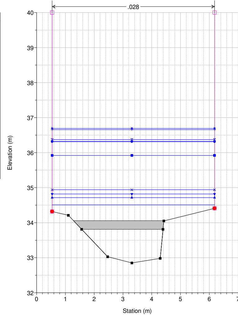
Studio Scandicci Torrenti Greve-Vingone River = Fosso Stagno Reach = Stagno RS = 21 SG0040_
