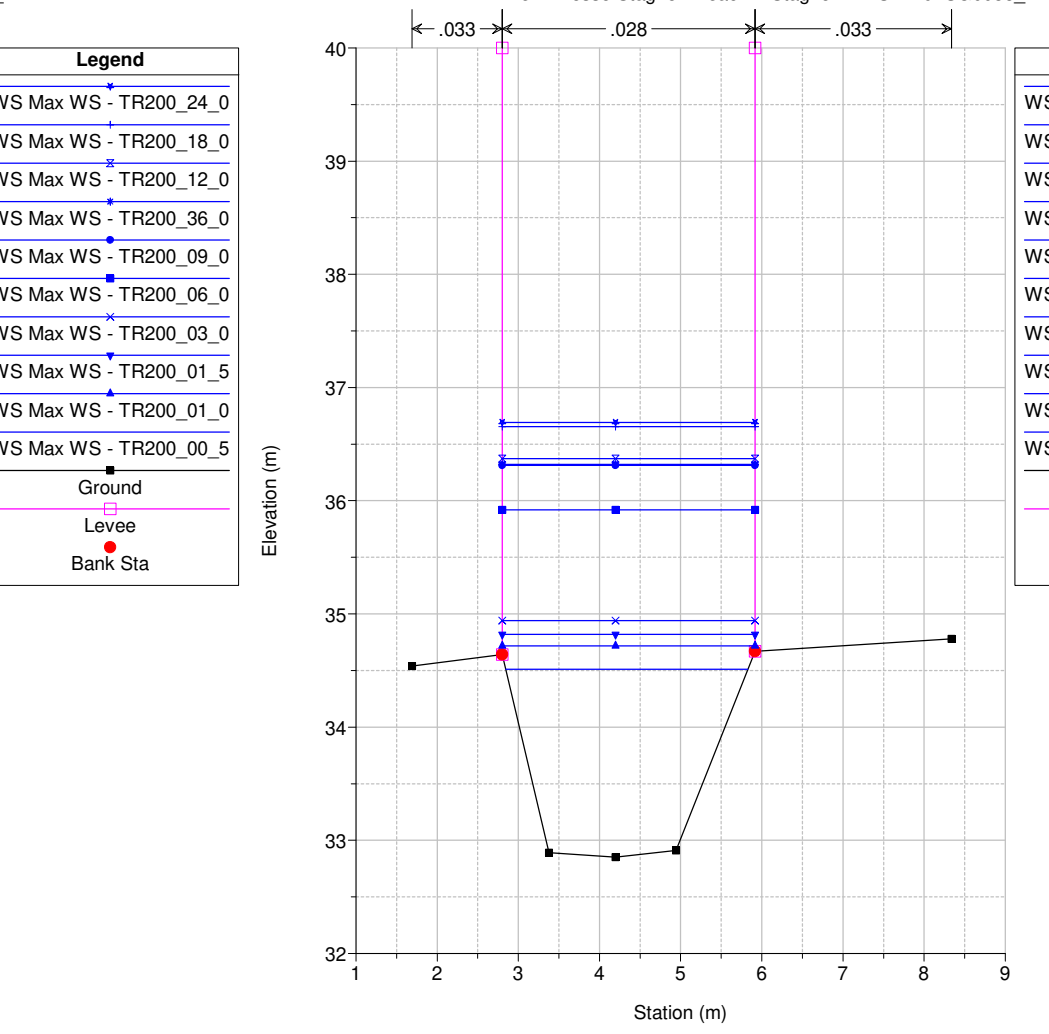
Studio Scandicci Torrenti Greve-Vingone River = Fosso Stagno Reach = Stagno RS = 29 SG0038_A
