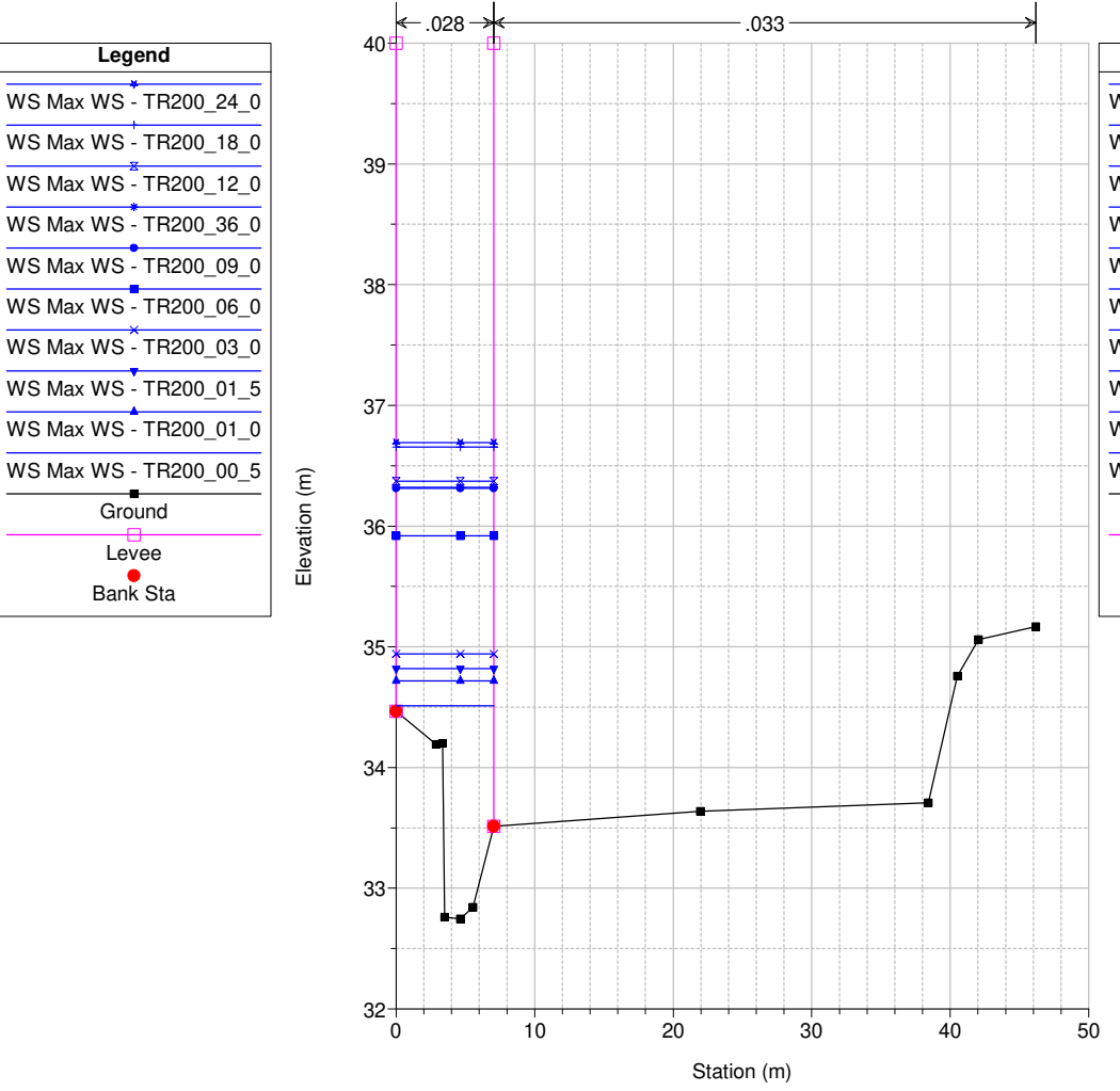
Studio Scandicci Torrenti Greve-Vingone River = Fosso Stagno Reach = Stagno RS = 30 SG0037
