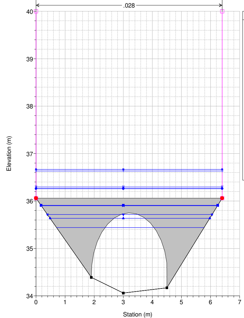
Studio Scandicci Torrenti Greve-Vingone River = Fosso Dogaione Reach = Dogaione RS = 45.5 BR
