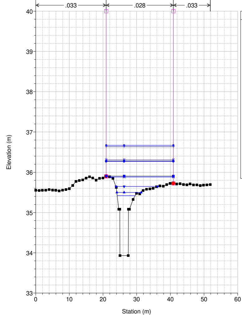
Studio Scandicci Torrenti Greve-Vingone River = Fosso Dogaione Reach = Dogaione RS = 24 DG1015_D
