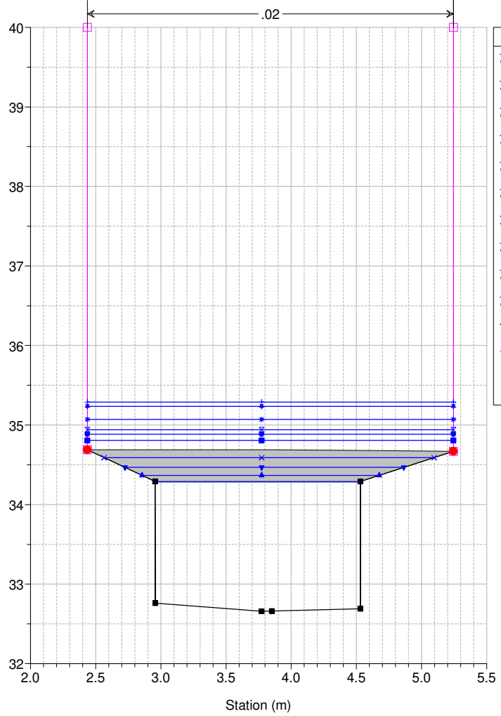
Studio Scandicci Torrenti Greve-Vingone River = Fosso Stagno Reach = Stagno RS = 46.75 BR
