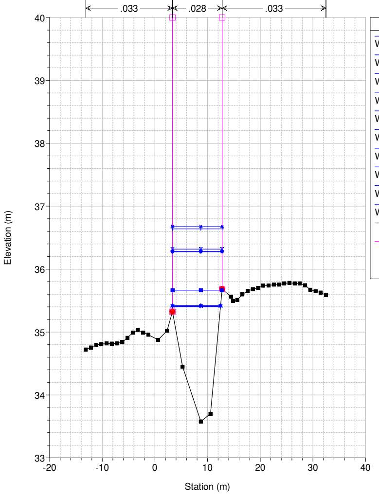
Studio Scandicci Torrenti Greve-Vingone River = Fosso Rigone Reach = Rigone 03 RS = 40 RI1012_
