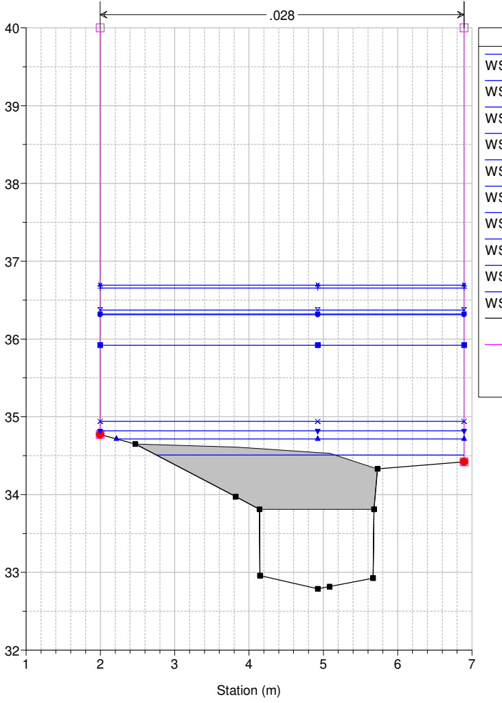
Studio Scandicci Torrenti Greve-Vingone River = Fosso Stagno Reach = Stagno RS = 25 SG0039_A
