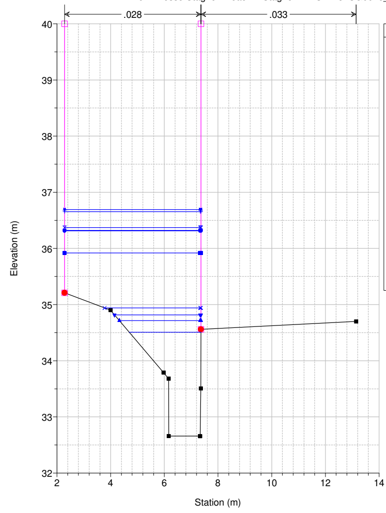
Studio Scandicci Torrenti Greve-Vingone River = Fosso Stagno Reach = Stagno RS = 13 SG0046_C
