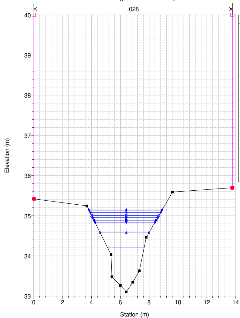
Studio Scandicci Torrenti Greve-Vingone River = Fosso Stagnolo Reach = Stagnolo RS = 38 ST0043_
