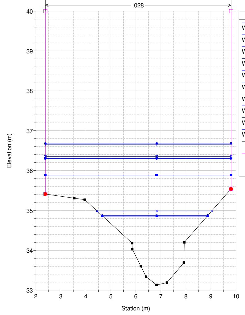
Studio Scandicci Torrenti Greve-Vingone River = Fosso Stagnolo Reach = Stagnolo RS = 41 ST0042_B
