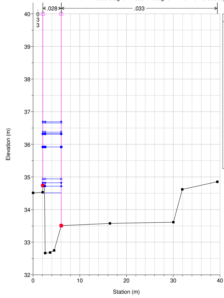
Studio Scandicci Torrenti Greve-Vingone River = Fosso Stagno Reach = Stagno RS = 31 SG0036
