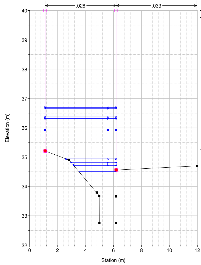
Studio Scandicci Torrenti Greve-Vingone River = Fosso Stagno Reach = Stagno RS = 13 SG0046_C
