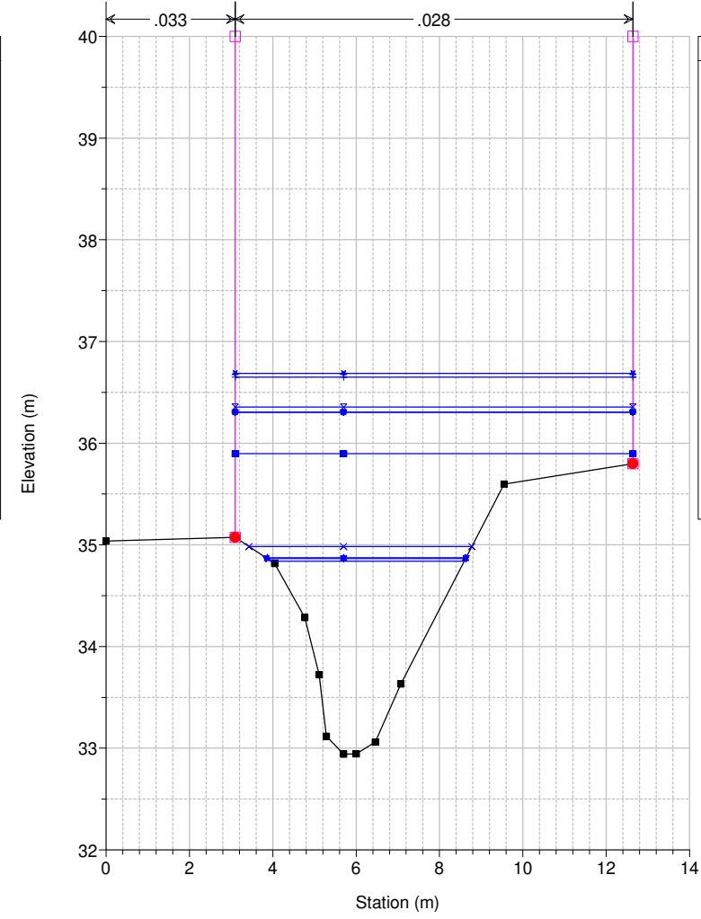
Studio Scandicci Torrenti Greve-Vingone River = Fosso Stagnolo Reach = Stagnolo RS = 18 ST0054_
