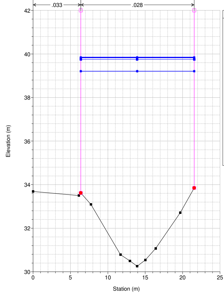
Studio Scandicci Torrenti Greve-Vingone River = Fosso Stagnolo Reach = Stagnolo RS = 1 ST0062_
