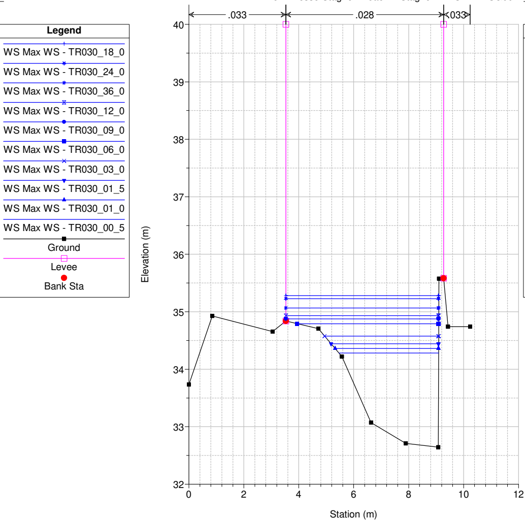
Studio Scandicci Torrenti Greve-Vingone River = Fosso Stagno Reach = Stagno RS = 11 SG0047_
