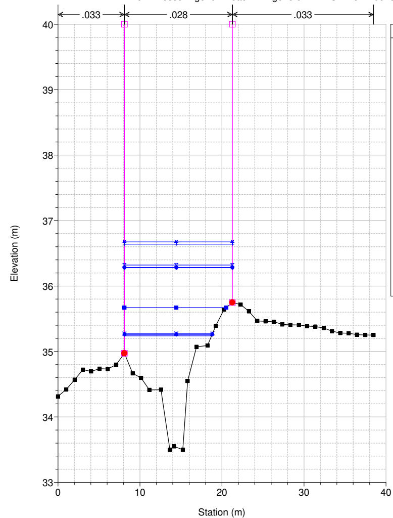
Studio Scandicci Torrenti Greve-Vingone River = Fosso Rigone Reach = Rigone 02 RS = 25 RI0018_A
