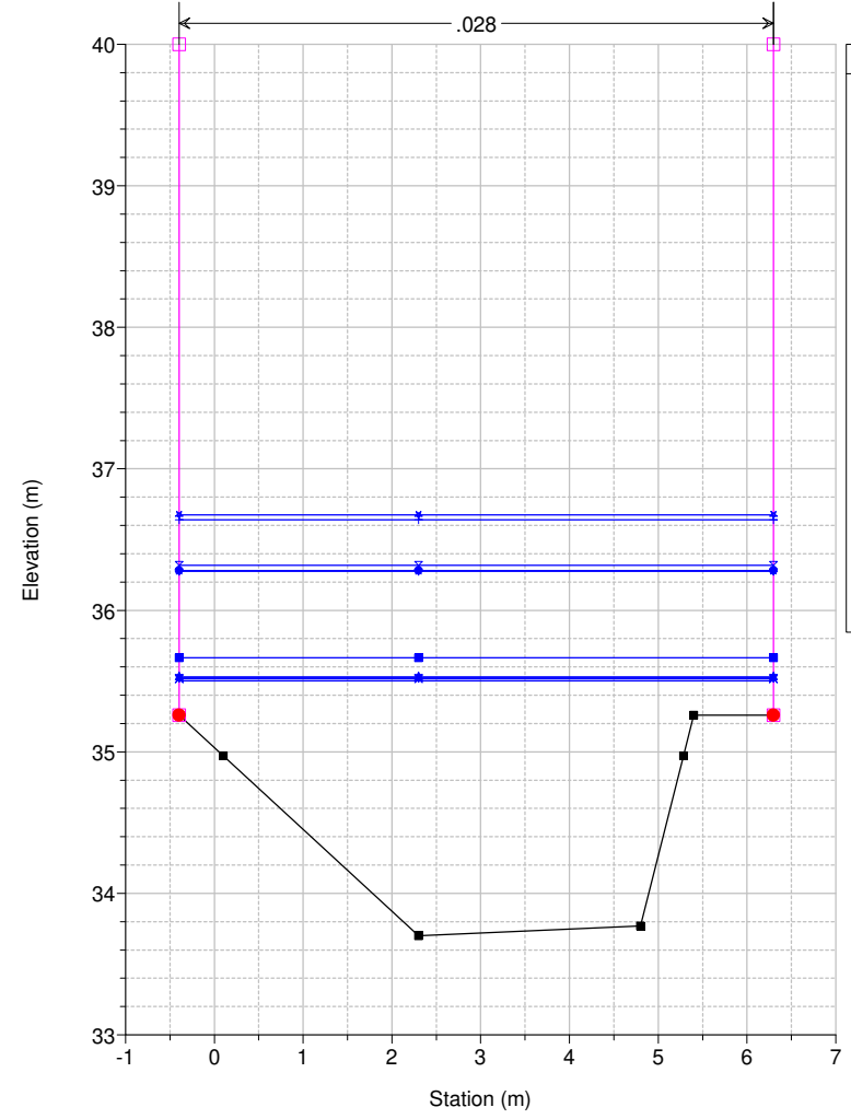
Studio Scandicci Torrenti Greve-Vingone River = Fosso Rigone Reach = Rigone 03 RS = 46 RI0010__
