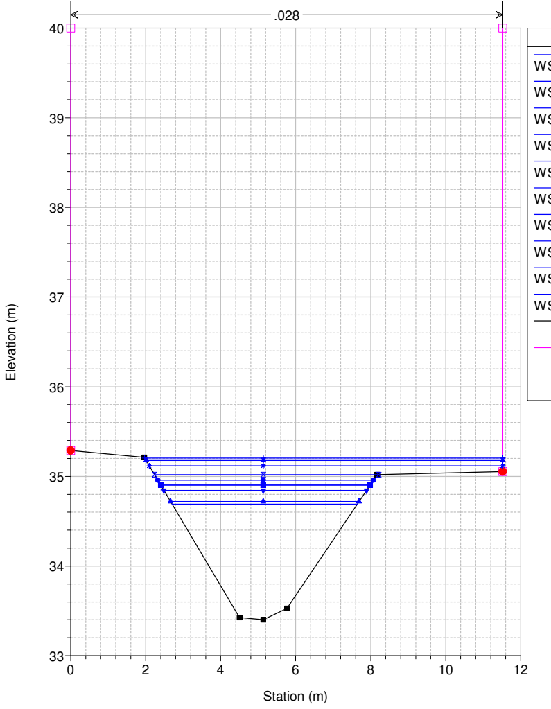
Studio Scandicci Torrenti Greve-Vingone River = Fosso Stagnolo Reach = Stagnolo RS = 80 ST0016_
