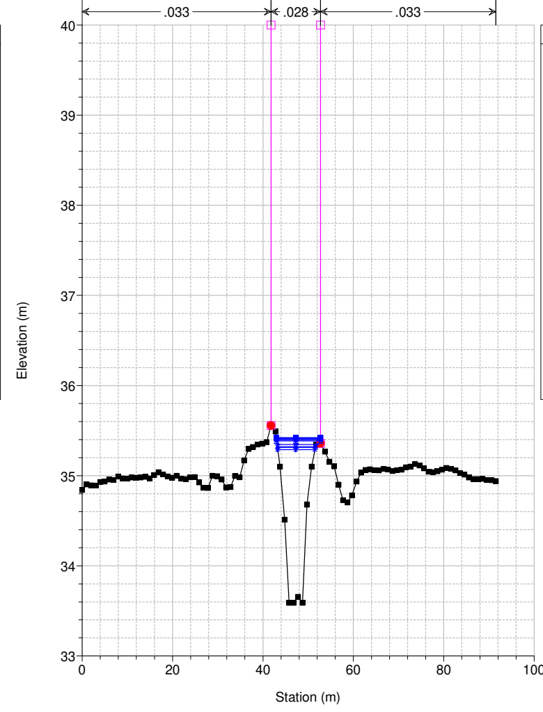
Studio Scandicci Torrenti Greve-Vingone River = Fosso Rigone Reach = Rigone 03 RS = 44 RI1011_A
