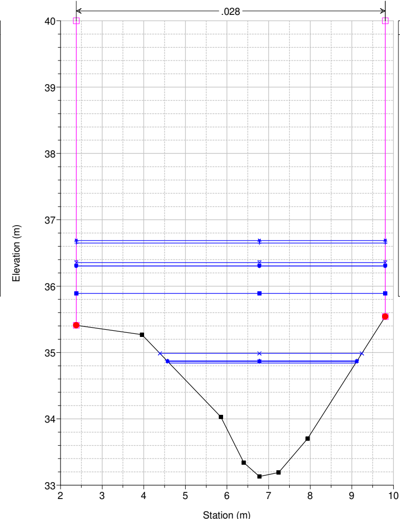
Studio Scandicci Torrenti Greve-Vingone River = Fosso Stagnolo Reach = Stagnolo RS = 36 ST0044_B
