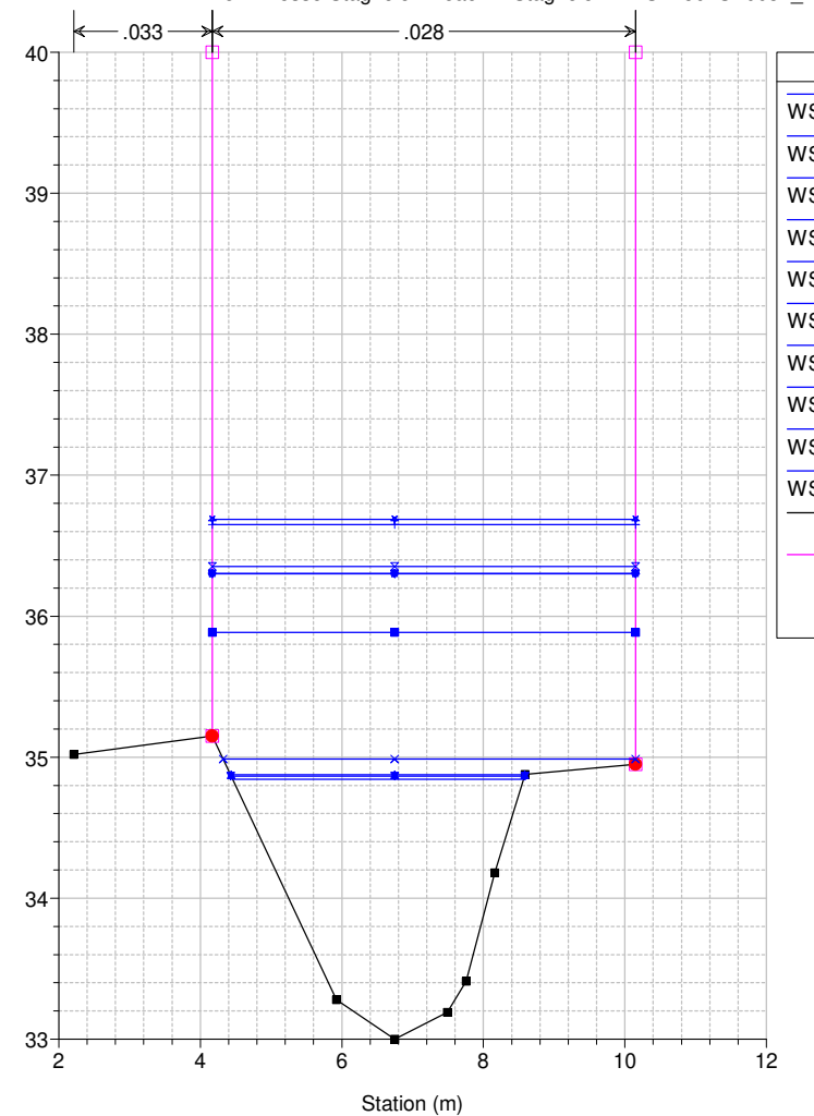
Studio Scandicci Torrenti Greve-Vingone River = Fosso Stagnolo Reach = Stagnolo RS = 50 ST0037_A
