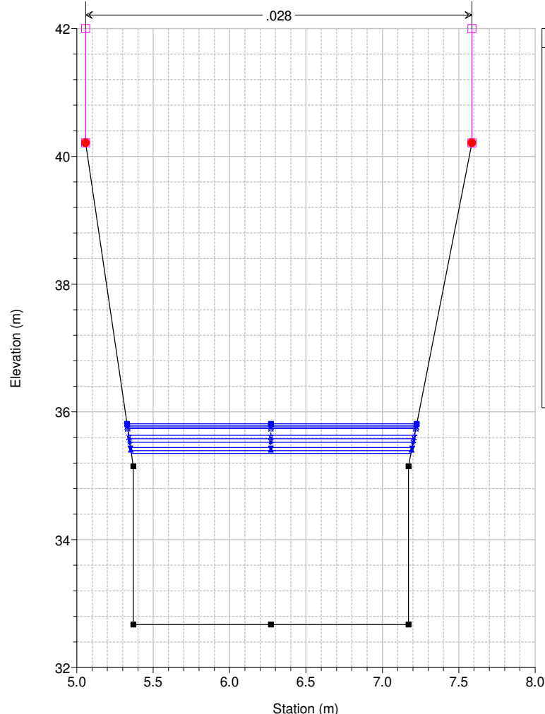
Studio Scandicci Torrenti Greve-Vingone River = Fosso Dogaione Reach = Dogaione RS = 1 DG0018_D
