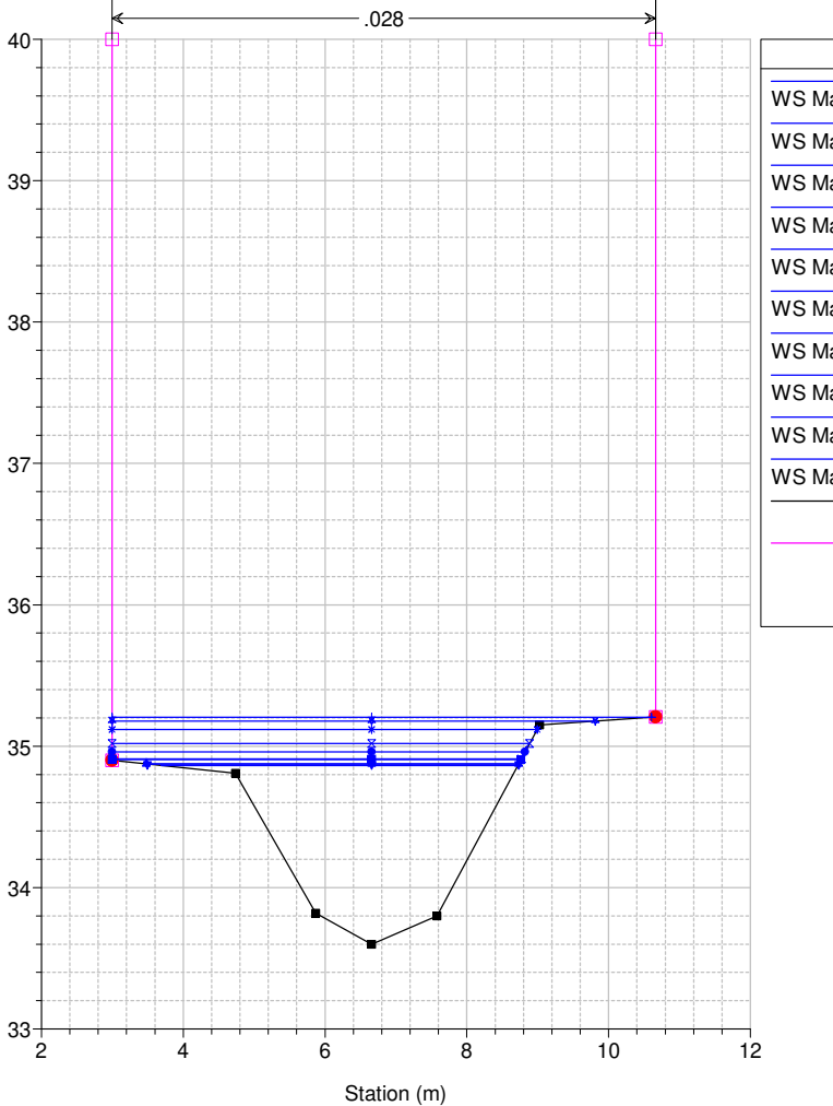
Studio Scandicci Torrenti Greve-Vingone River = Fosso Stagnolo Reach = Stagnolo RS = 94 ST0008_A
