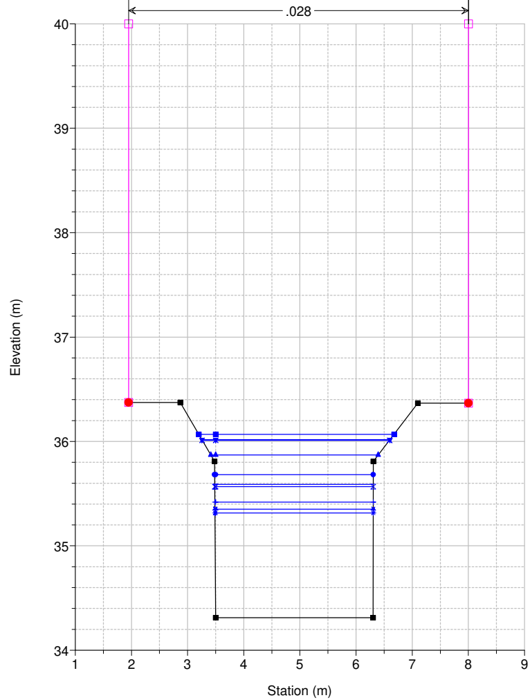
Studio Scandicci Torrenti Greve-Vingone River = Fosso Rigone Reach = Rigone 03 RS = 55.75 BR
