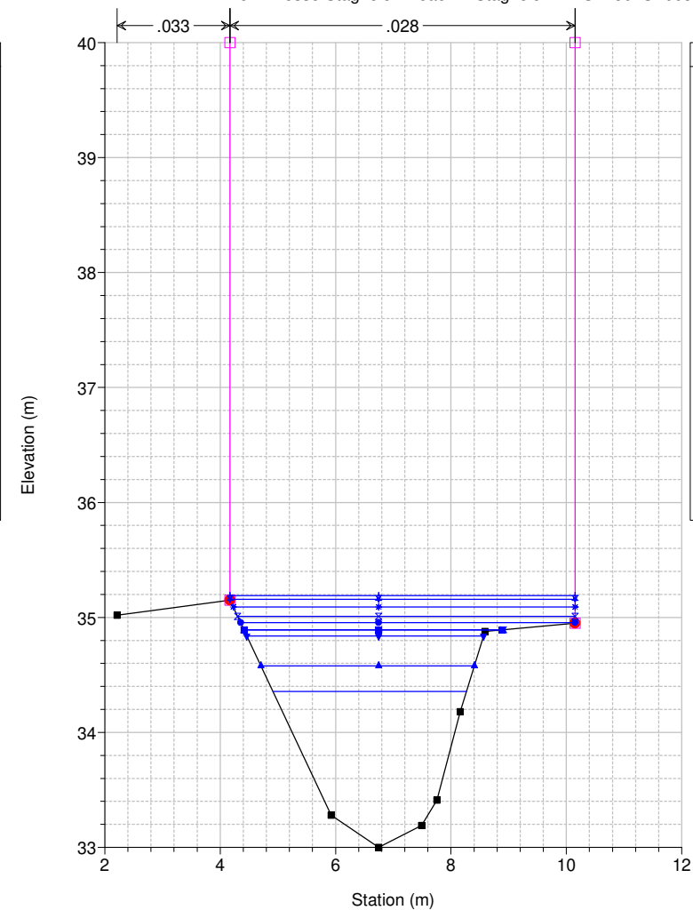
Studio Scandicci Torrenti Greve-Vingone River = Fosso Stagnolo Reach = Stagnolo RS = 50 ST0037_A
