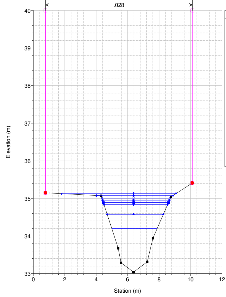
Studio Scandicci Torrenti Greve-Vingone River = Fosso Stagnolo Reach = Stagnolo RS = 24 ST0050_B
