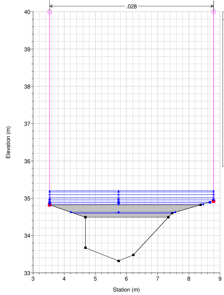
Studio Scandicci Torrenti Greve-Vingone River = Fosso Stagnolo Reach = Stagnolo RS = 68 ST0022_
