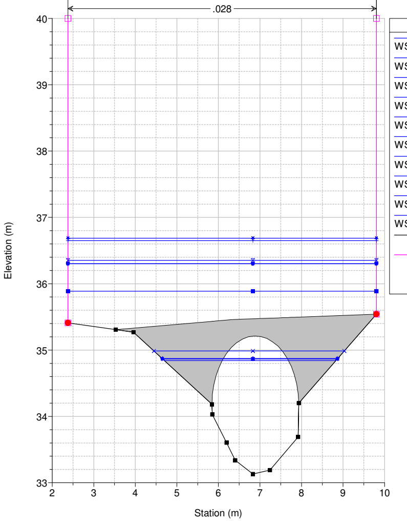
Studio Scandicci Torrenti Greve-Vingone River = Fosso Stagnolo Reach = Stagnolo RS = 40.5 BR
