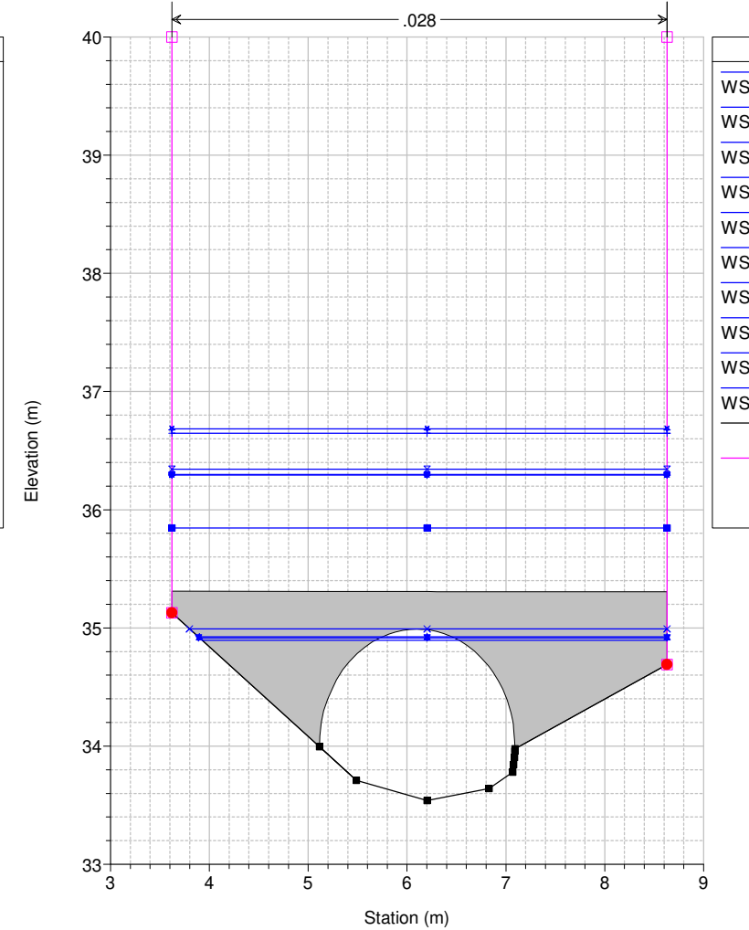
Studio Scandicci Torrenti Greve-Vingone River = Fosso Stagnolo Reach = Stagnolo RS = 90 ST0009_
