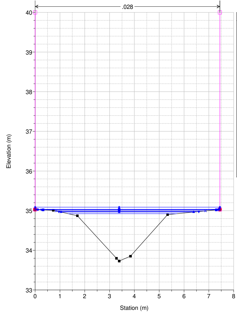
Studio Scandicci Torrenti Greve-Vingone River = Fosso Botteghino Reach = Botteghino RS = 10.5 BR
