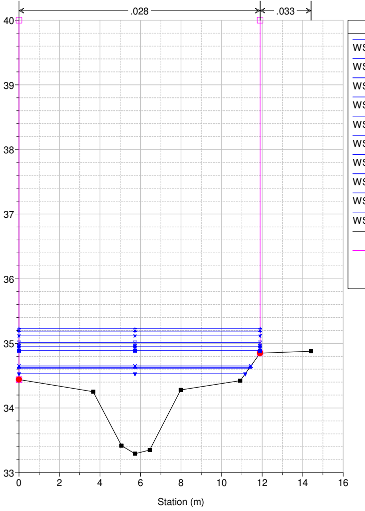
Studio Scandicci Torrenti Greve-Vingone River = Fosso Stagno Reach = Stagno RS = 82 SG0012_B
