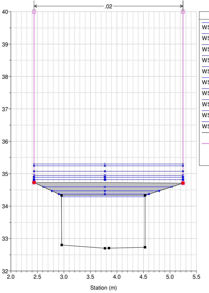
Studio Scandicci Torrenti Greve-Vingone River = Fosso Stagno Reach = Stagno RS = 48 SG0024_Q
