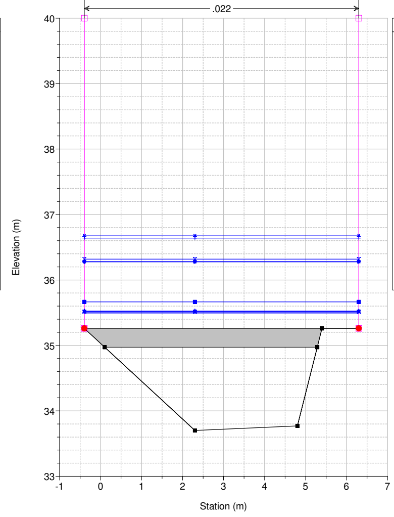
Studio Scandicci Torrenti Greve-Vingone River = Fosso Rigone Reach = Rigone 03 RS = 49.5 BR
