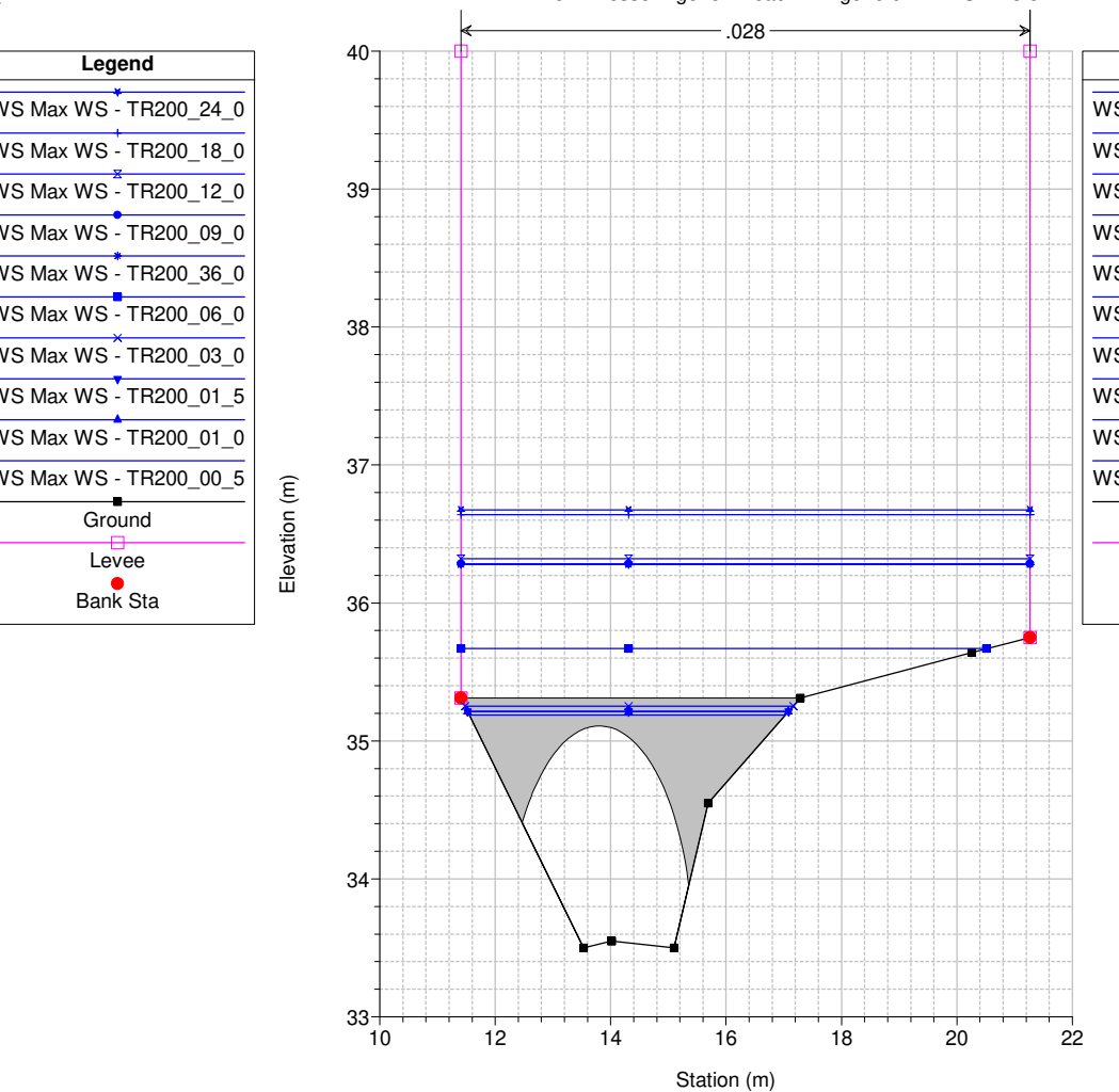
Studio Scandicci Torrenti Greve-Vingone River = Fosso Rigone Reach = Rigone 02 RS = 23.5 BR
