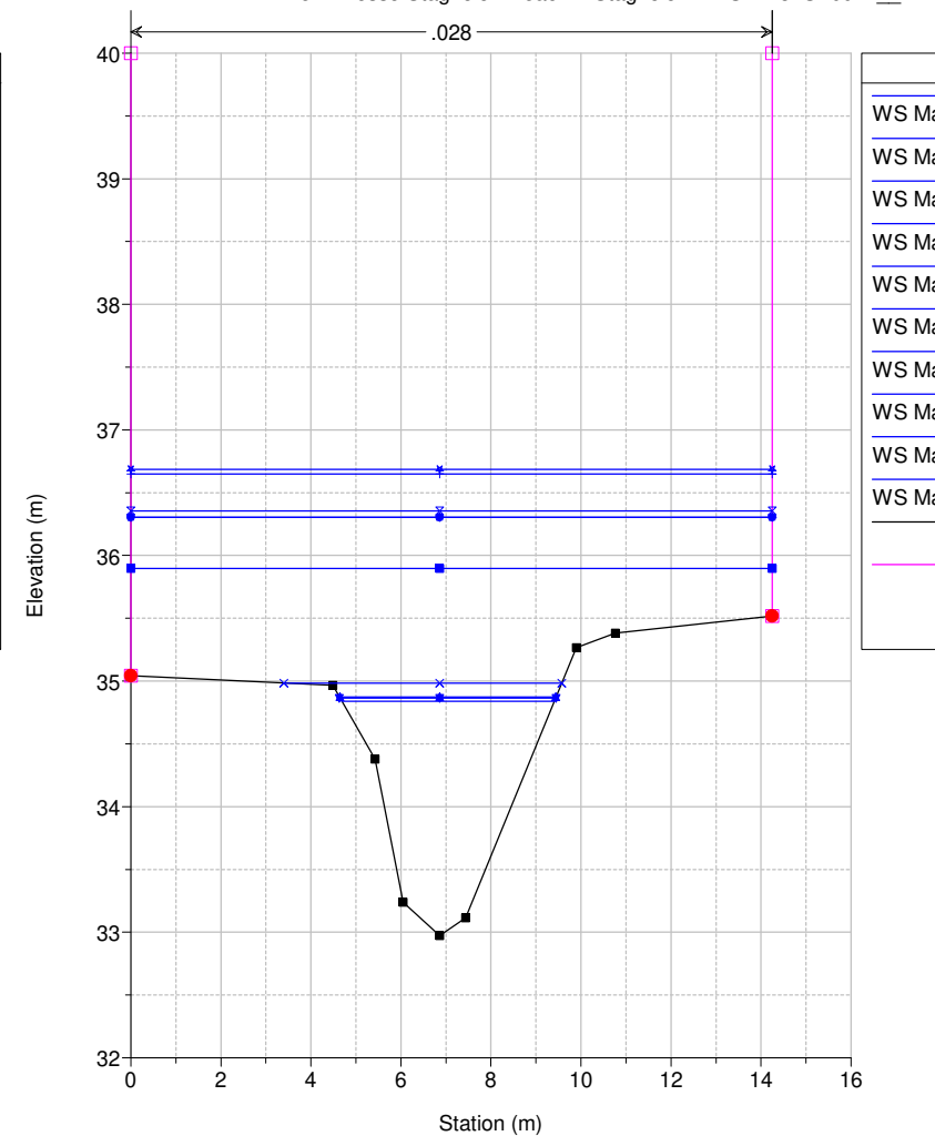
Studio Scandicci Torrenti Greve-Vingone River = Fosso Stagnolo Reach = Stagnolo RS = 28 ST0047_
