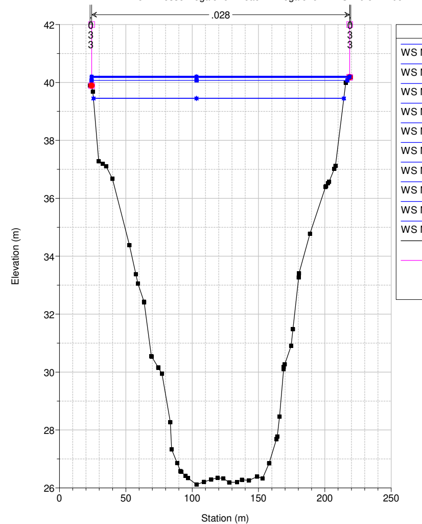
Studio Scandicci Torrenti Greve-Vingone River = Fosso Dogaione Reach = Dogaione RS = 0.5 AR0521
