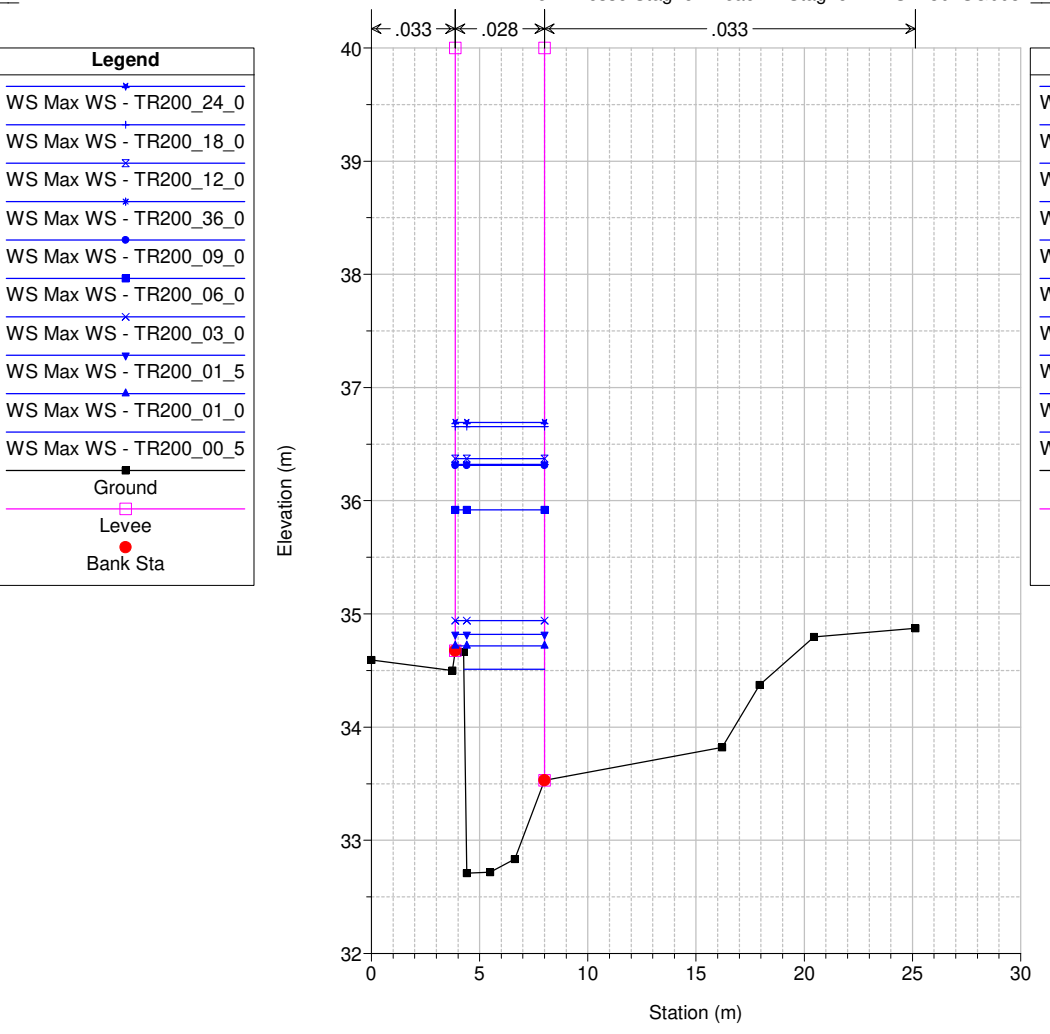
Studio Scandicci Torrenti Greve-Vingone River = Fosso Stagno Reach = Stagno RS = 30 SG0037
